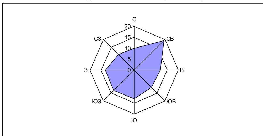
Рисунок 1.2.12.4 - Среднегодовая роза ветров, %
