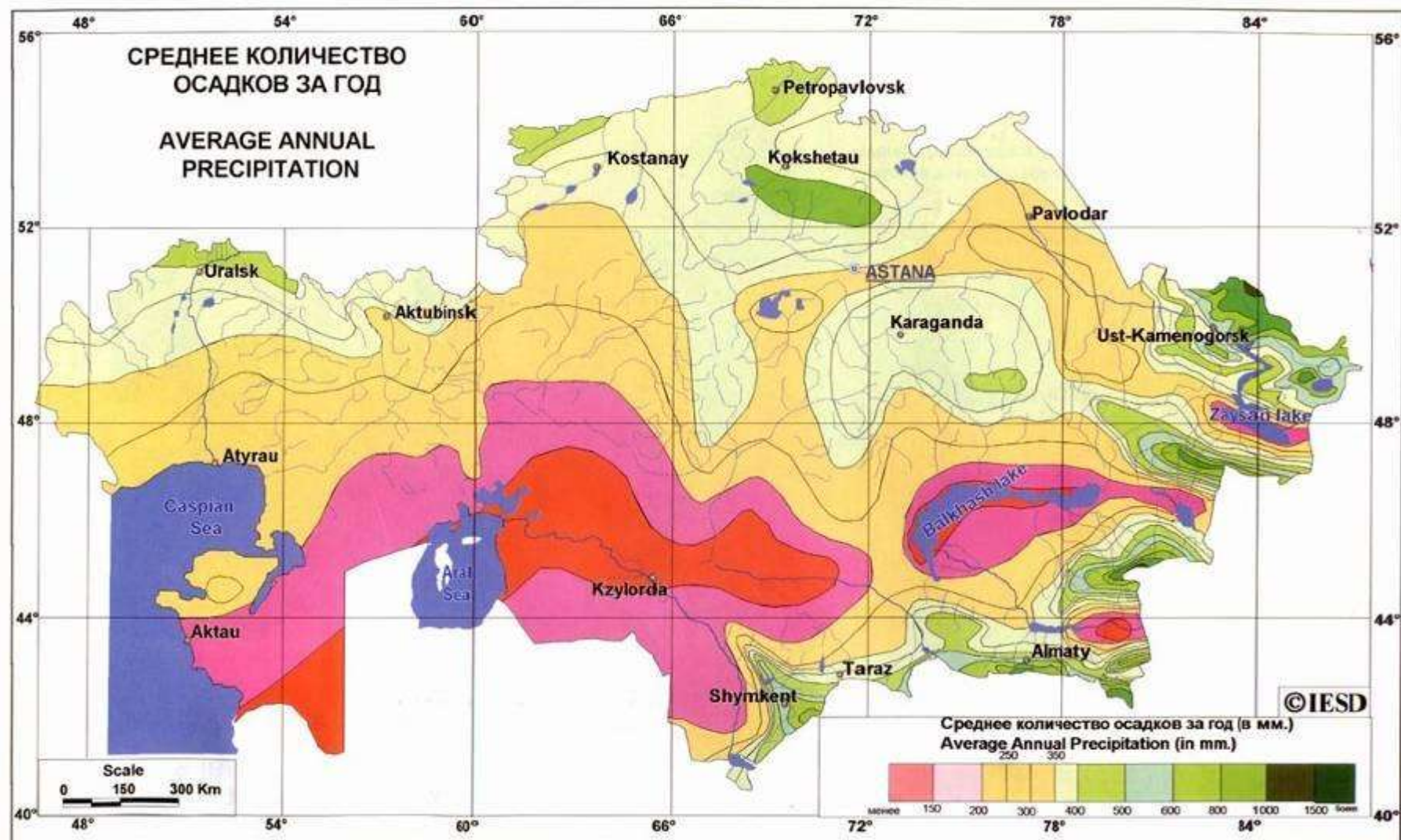
Рисунок 1.2.12.3 – Среднегодовое количество осадков
