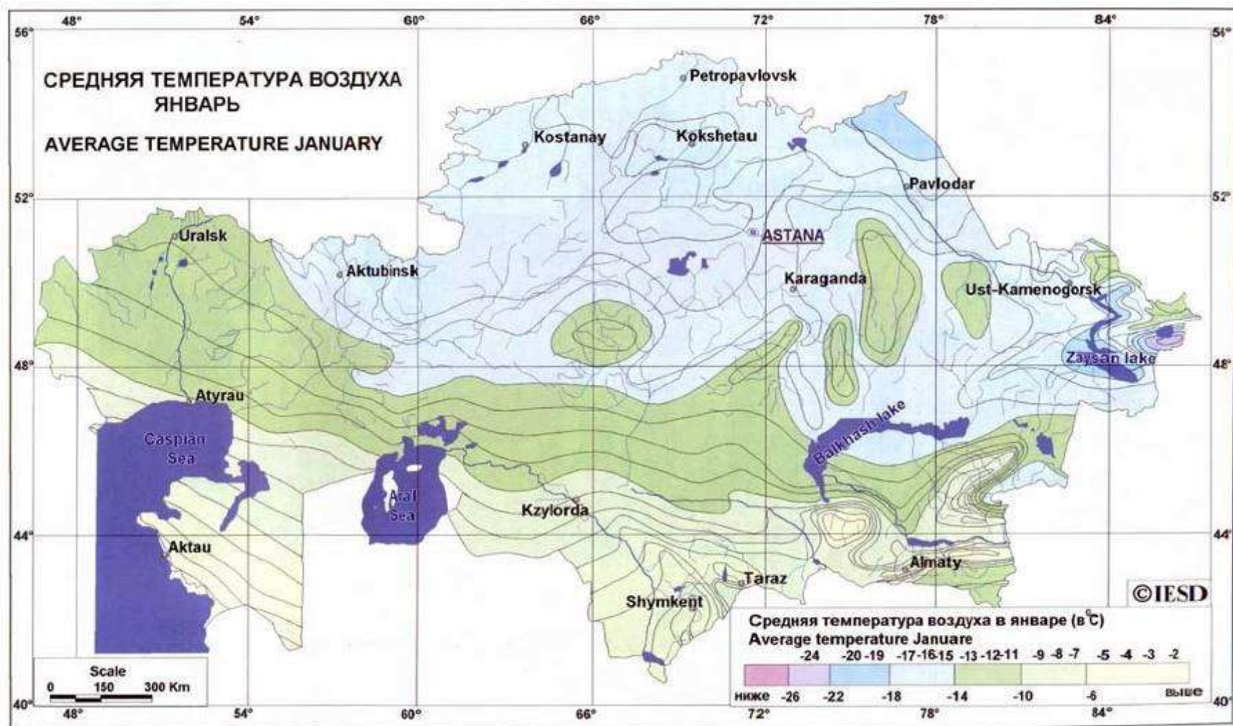
Рисунок 1.2.12.2 – Средняя температура воздуха. Январь
