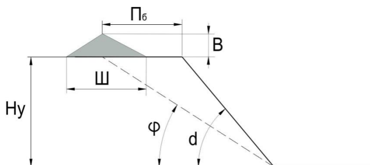
Рис.7Схема уступа
