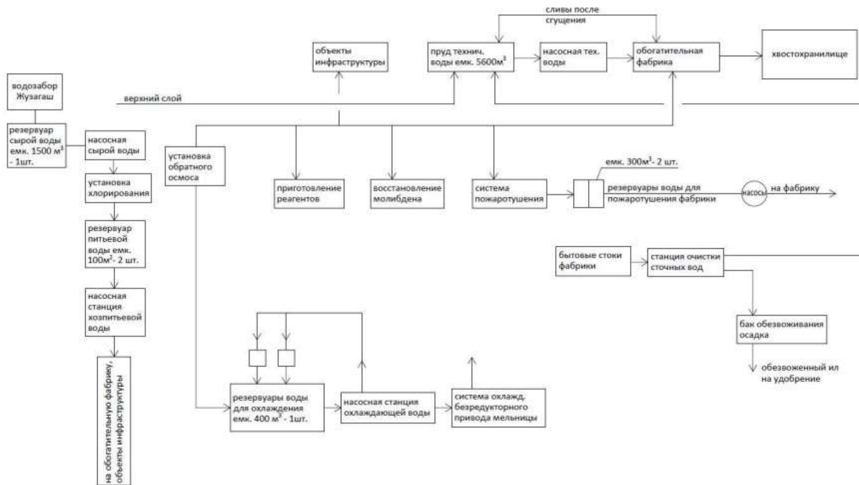
Рисунок 5.2 - Схема водопотребления и водоотведения
