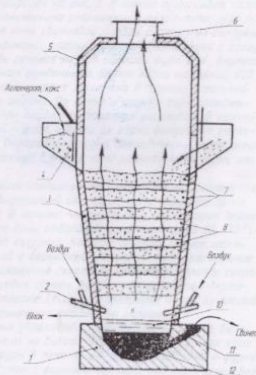
Рис.1. Схема шахтной печи свинцовой плавки
