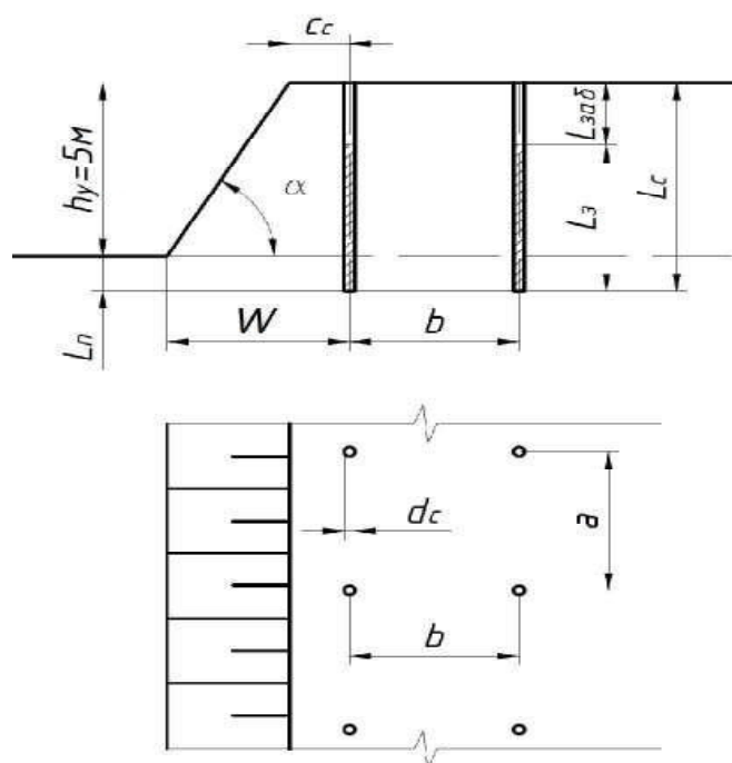
Рисунок 3.7 – Схема расположения технологических скважин в массиве горных пород
