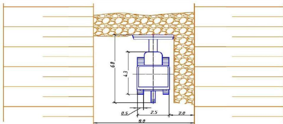
Рисунок 3.8 – Схема механизированной очистки предохранительной бермы с применением бульдозера.
