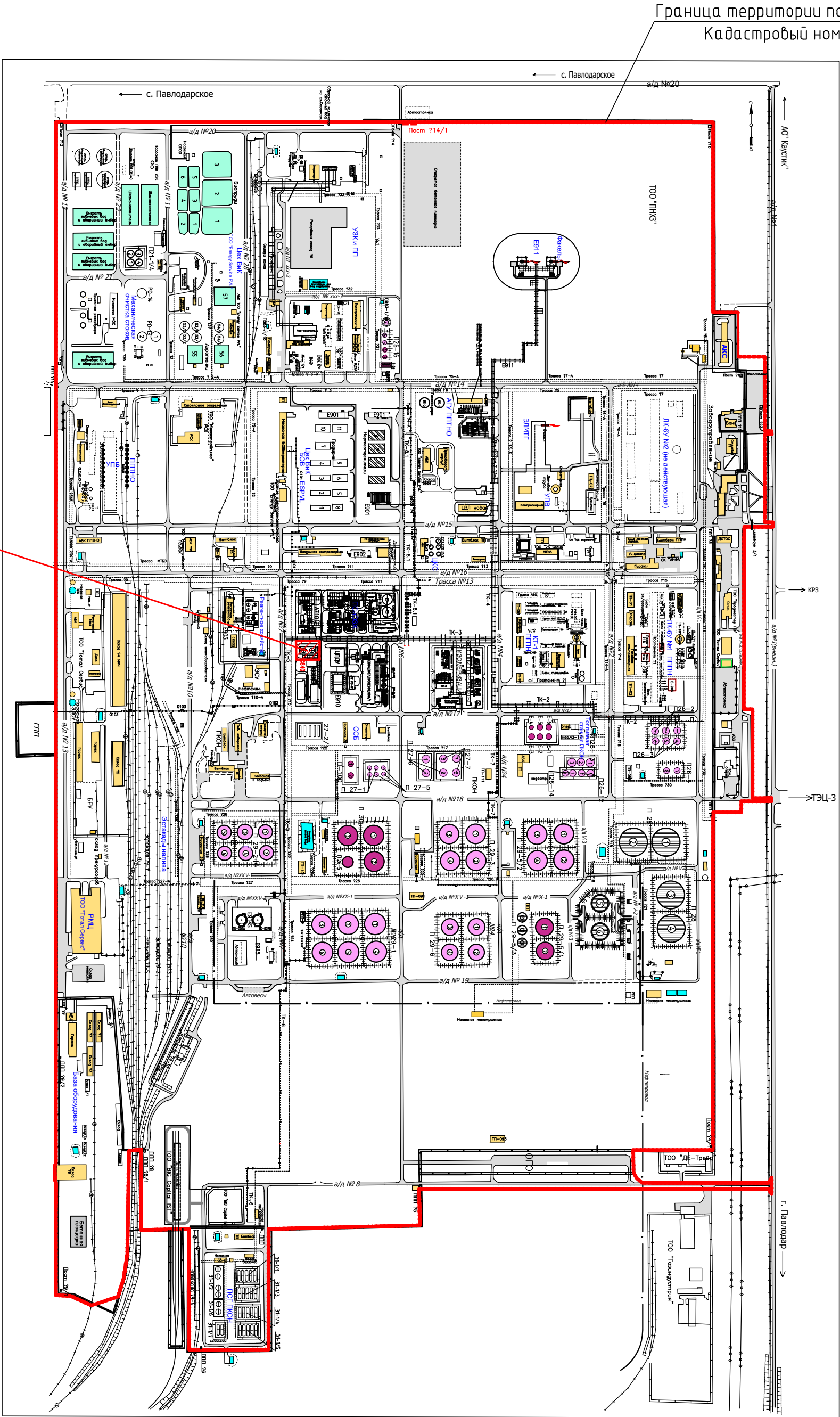
Ситуационная схема ТОО "ПНХЗ"
