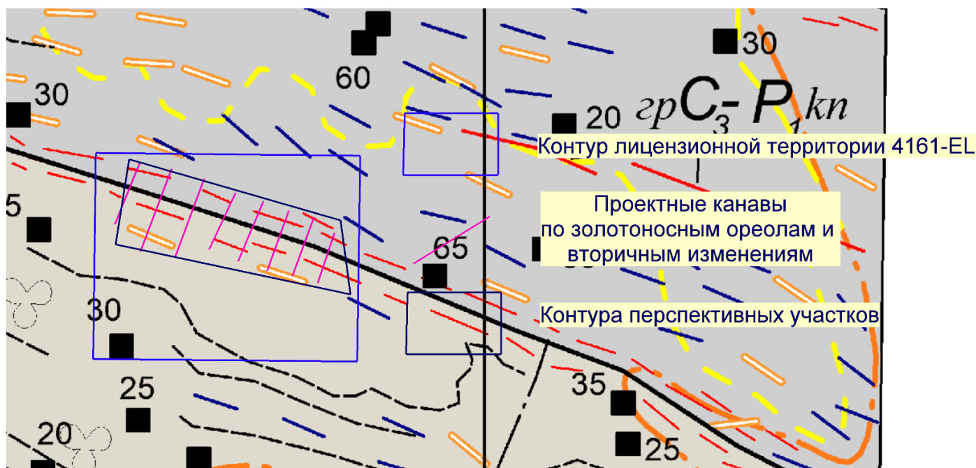
Рис.2 Схематическая карта расположения вторичных ореолов и полезных ископаемых с нанесёнными проектными горными выработками
