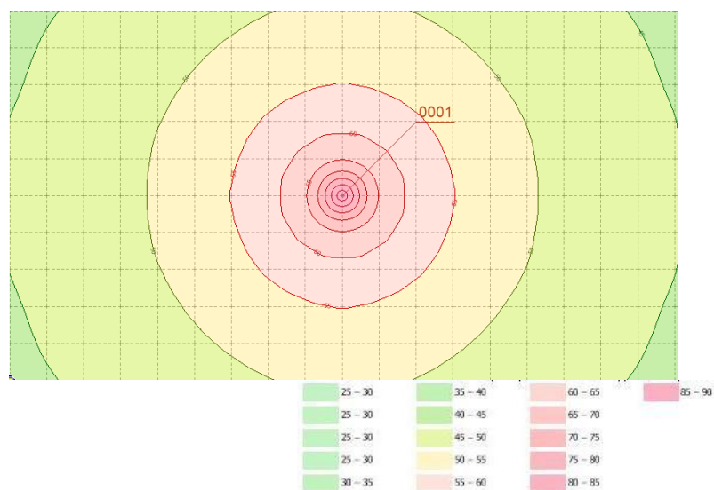
Рисунок 2 – Результаты расчёта затухания звука в графической форме в рабочей зоне оборудования при проведении разведочных работ (эквивалентный уровень звука – интегральный показатель)
