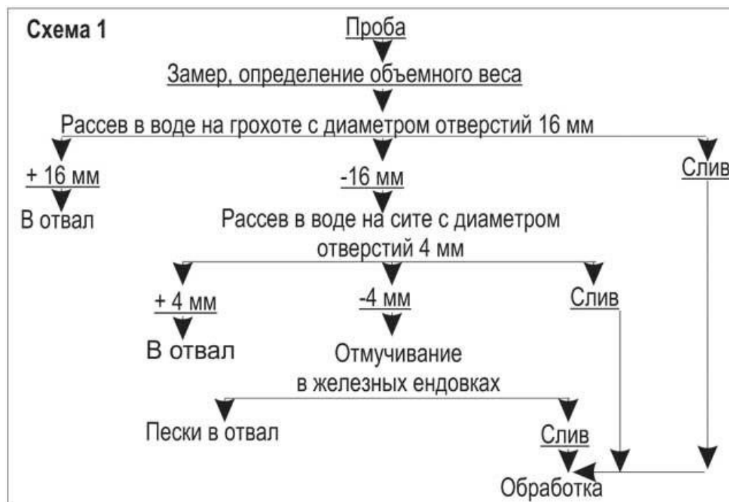
Рисунок 2. Схема обработки технологических проб
