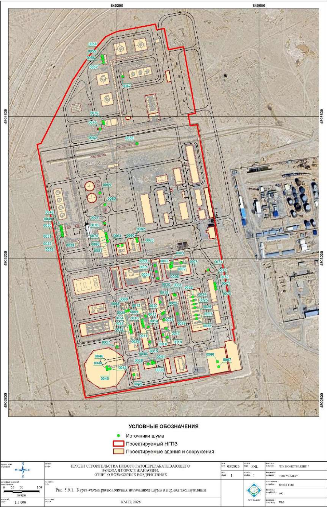
Рисунок 5.9.1 Карта-схема расположения источниками шума на период эксплуатации
