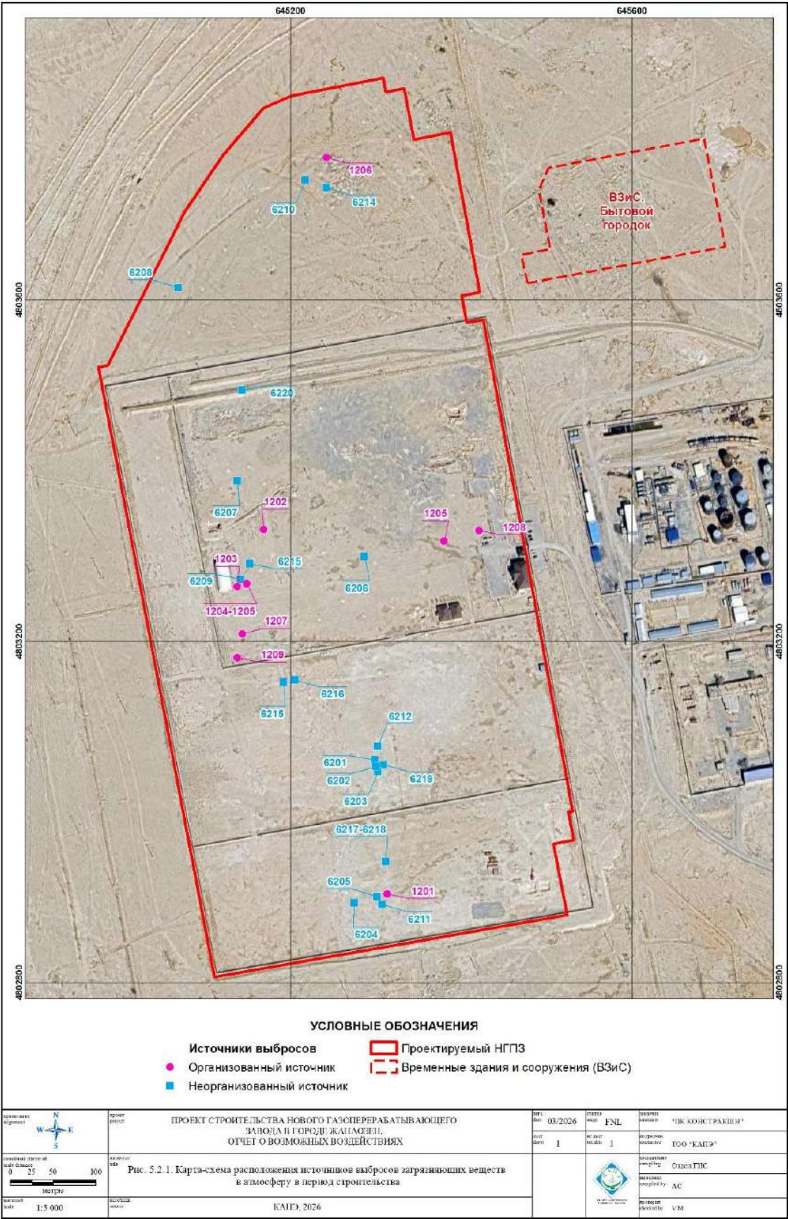
Рисунок 5.2.1 Карта-схема расположения источников выбросов загрязняющих веществ в атмосферу в период строительства
