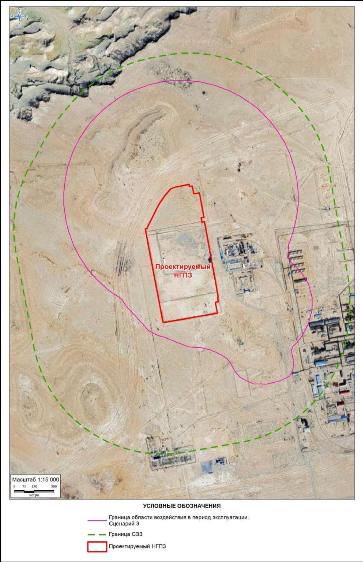
Рисунок 5.2.6 Граница области воздействия в период эксплуатации. Сценарий 3
