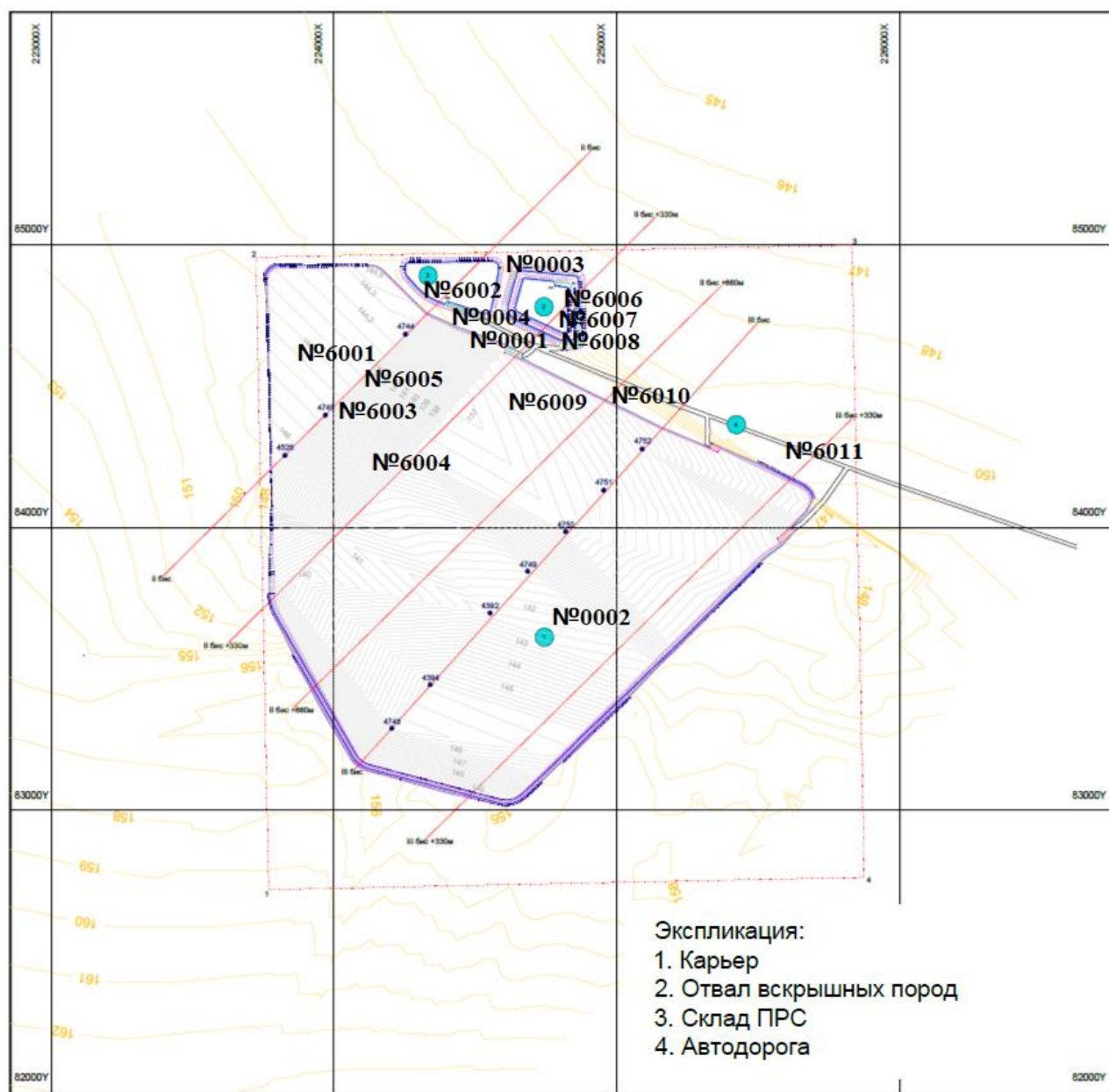
Рис. 1.8.1 – Карта-схема источников выбросов при проведении работ на период эксплуатации месторождения Дружба
