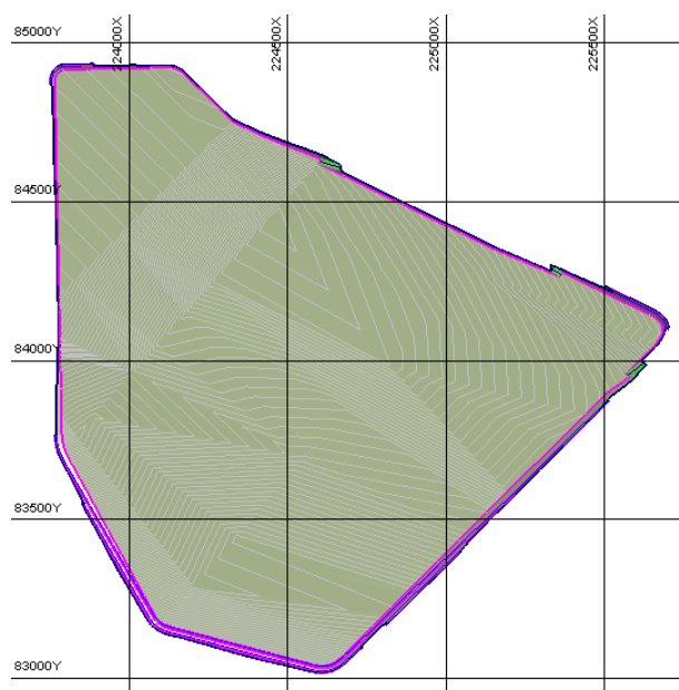
Рис. 1.8 – План Карьера на конец отработки
