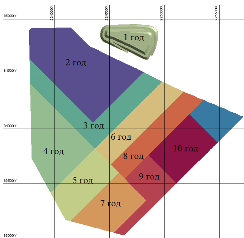
Рис. 1.10 – Схема размещения вскрышных пород в отвалах
