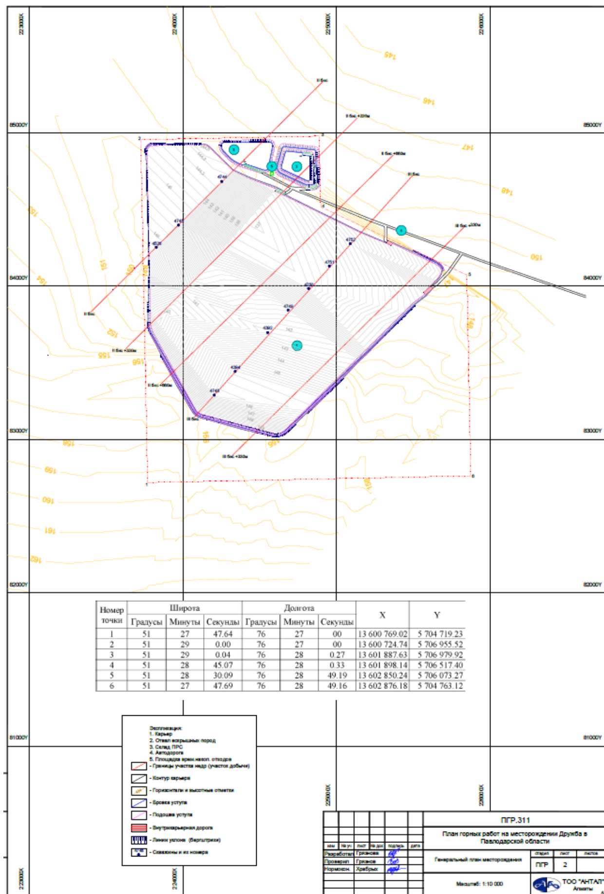
Рис. 1.9.1 Генеральный план горных работ с площадкой временного накопления отходов
