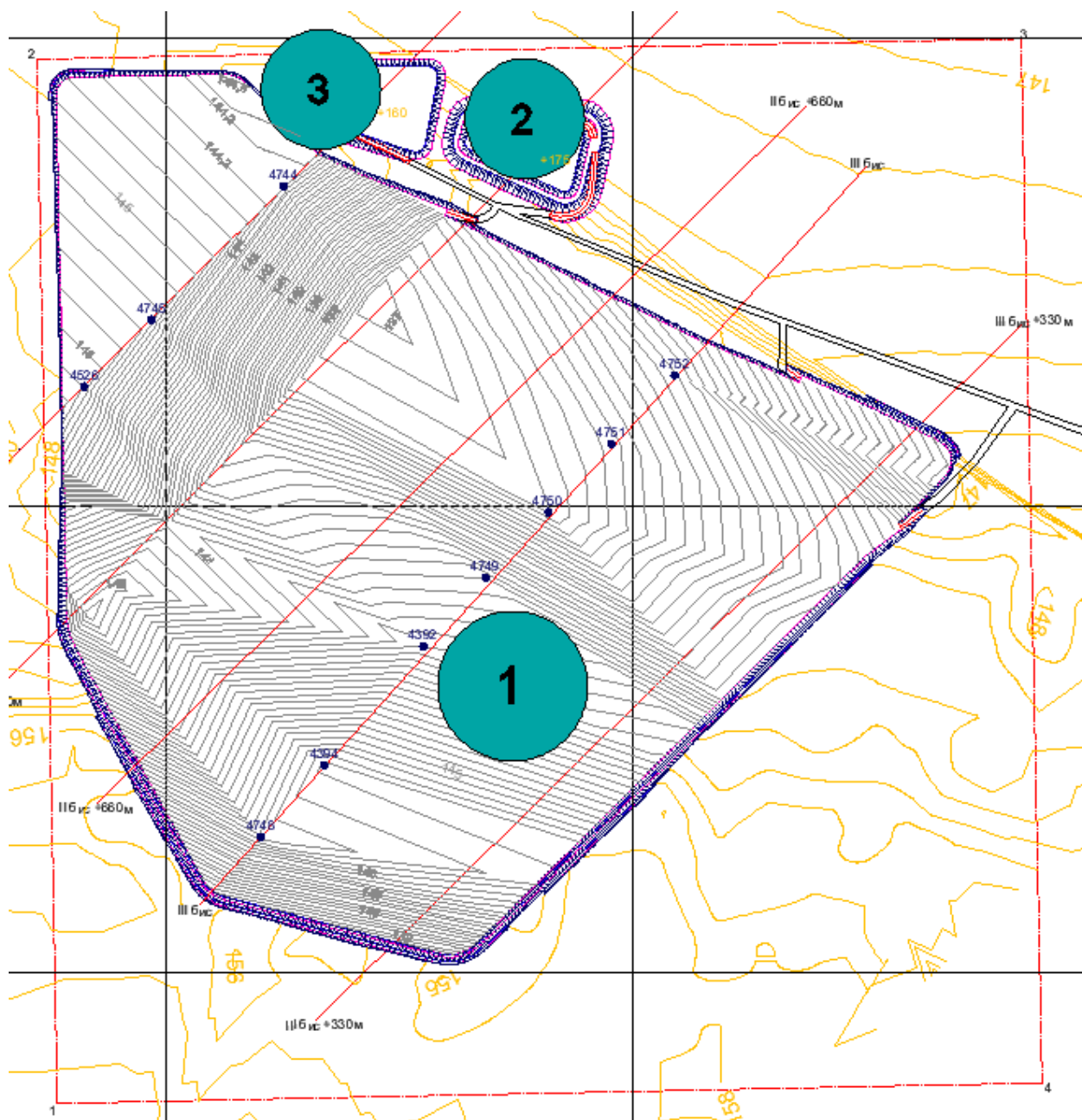
Рис. 1.3 – Карта-схема с проектируемыми объектами горного производства
