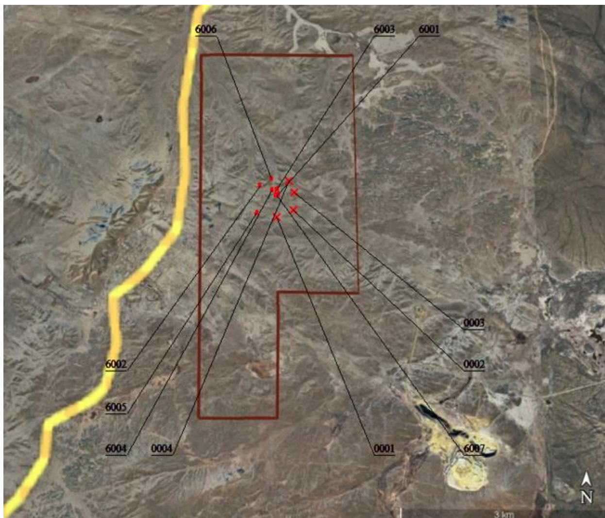
Рисунок 1.4 Карта-схема района расположения участка работ с указанием источников выбросов
