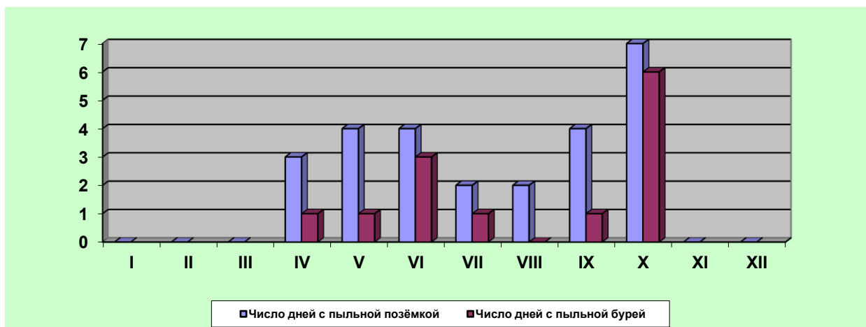
Рисунок 9 Пыльные бури
