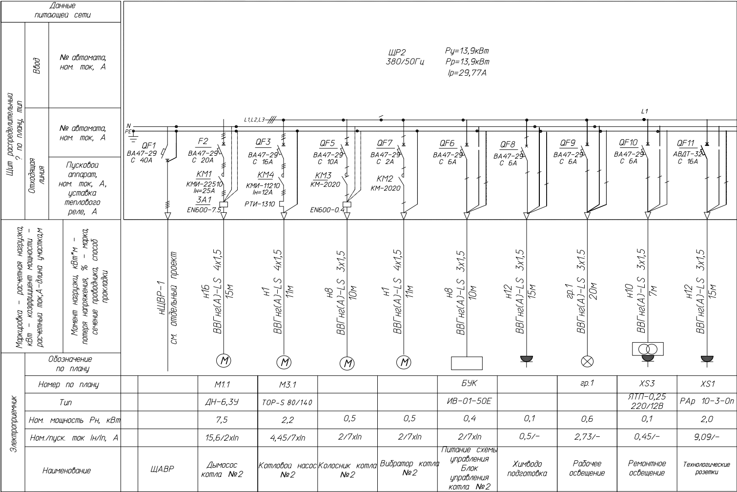
Рисунок 4.4. Однолинейная схема ЩР2
