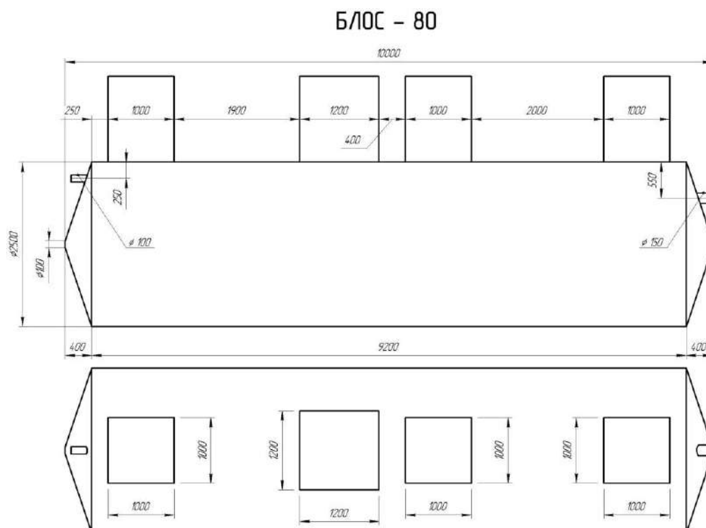
Рис. 1б Общий вид подземной части (технологический блок) установки БЛОС-80
