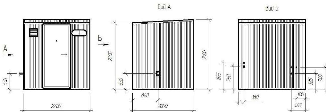
Рис. 1а Общий вид надземной части (блок управления) установки БЛОС-80
