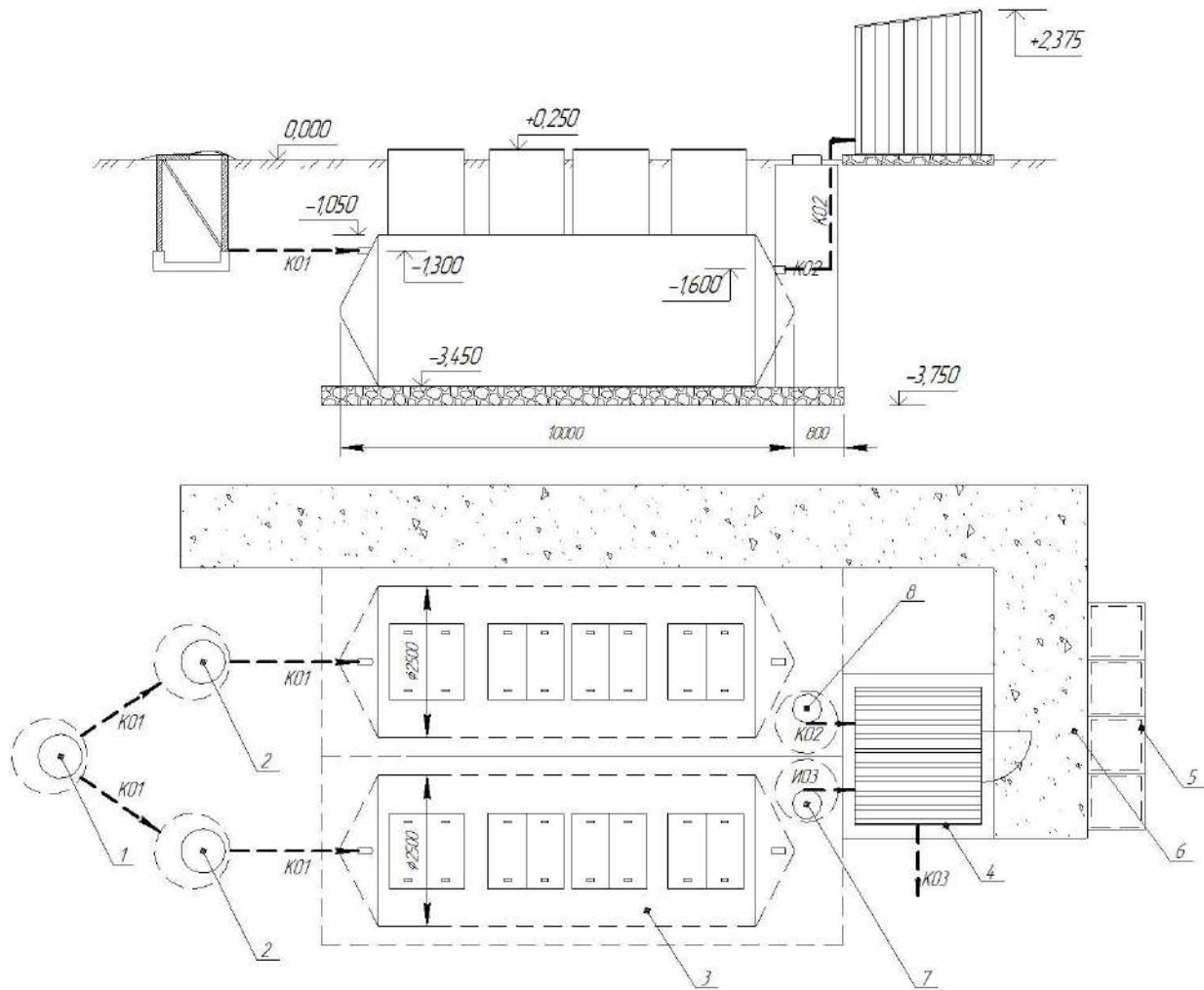
Рис. 2 Схема установки БЛОС-80
