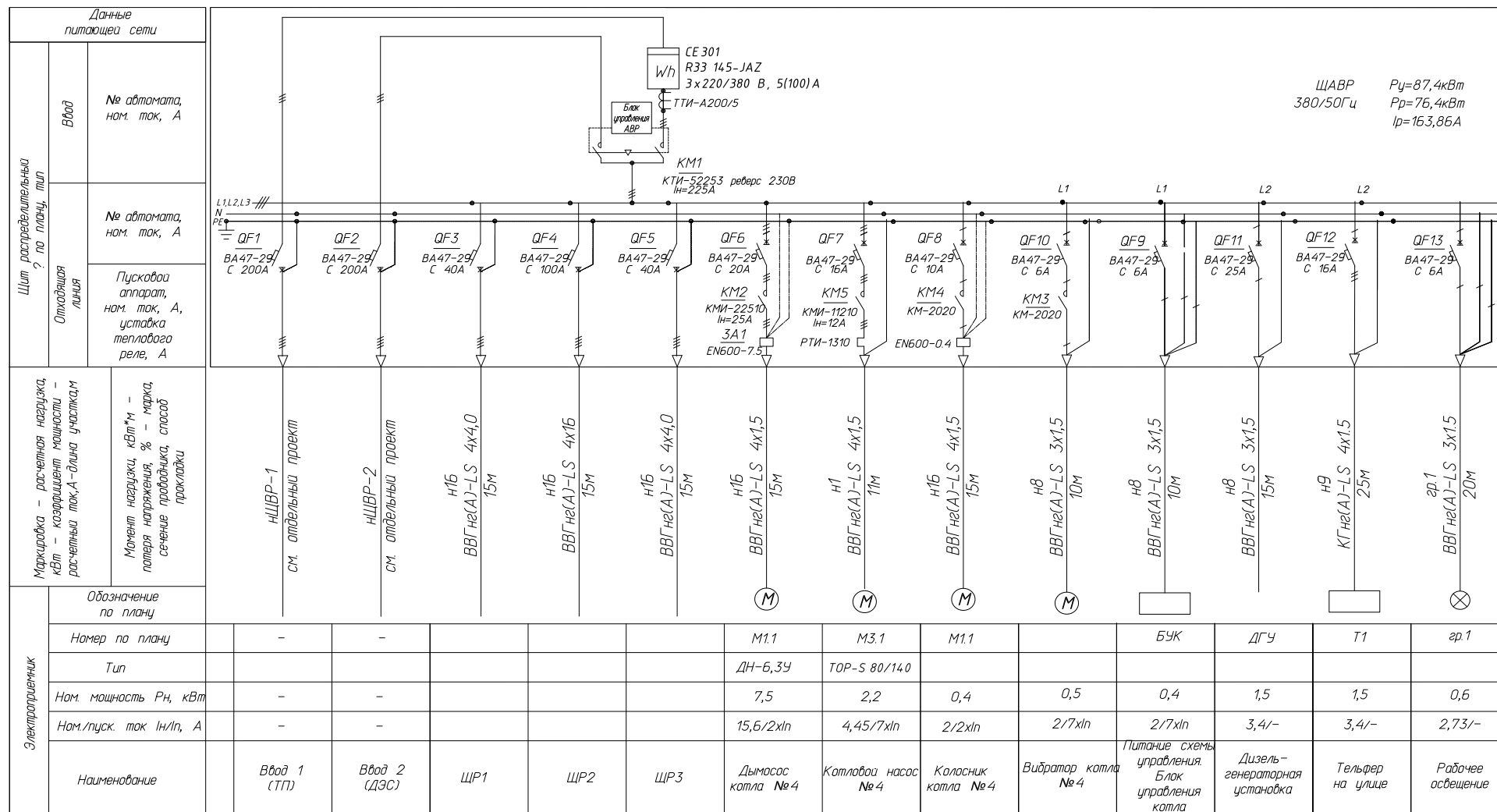
Рисунок 4.2. Однолинейная схема ЩАВР
