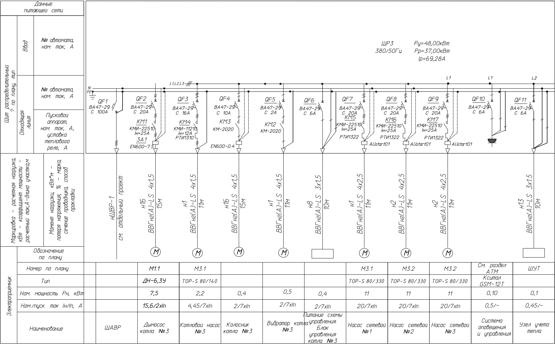
Рисунок 4.5. Однолинейная схема ЩРЗ
