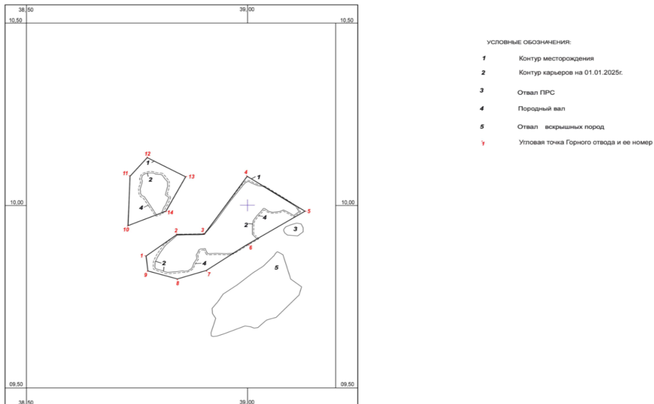
Рис.6. Ситуационный план карьера после проведения ликвидационно-рекультивационных работ. Масштаб 1:5 000
