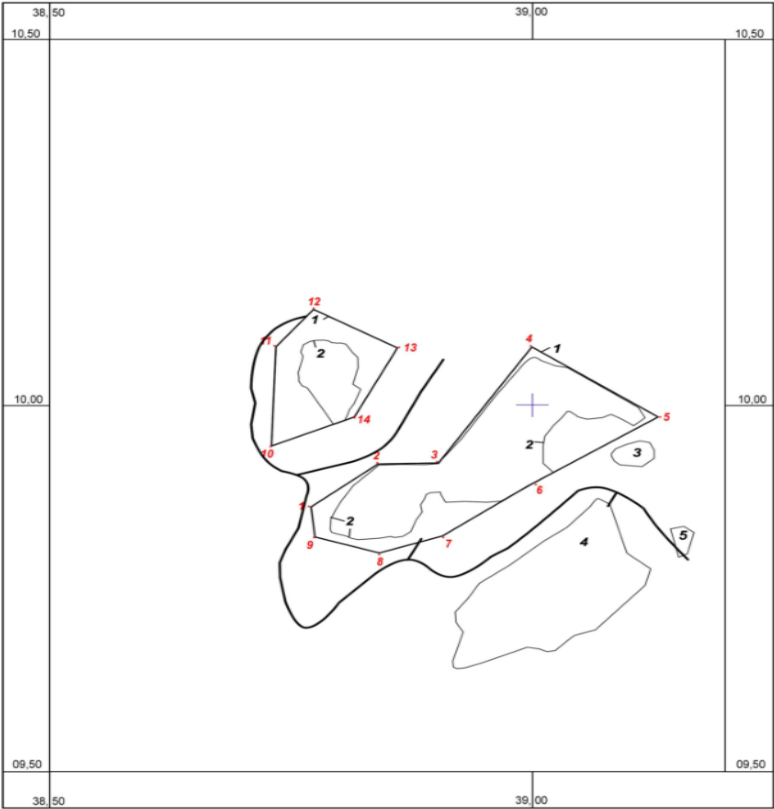
Рис.5. Ситуационный план карьера на 01.01.2025г. Масштаб 1:5 000
