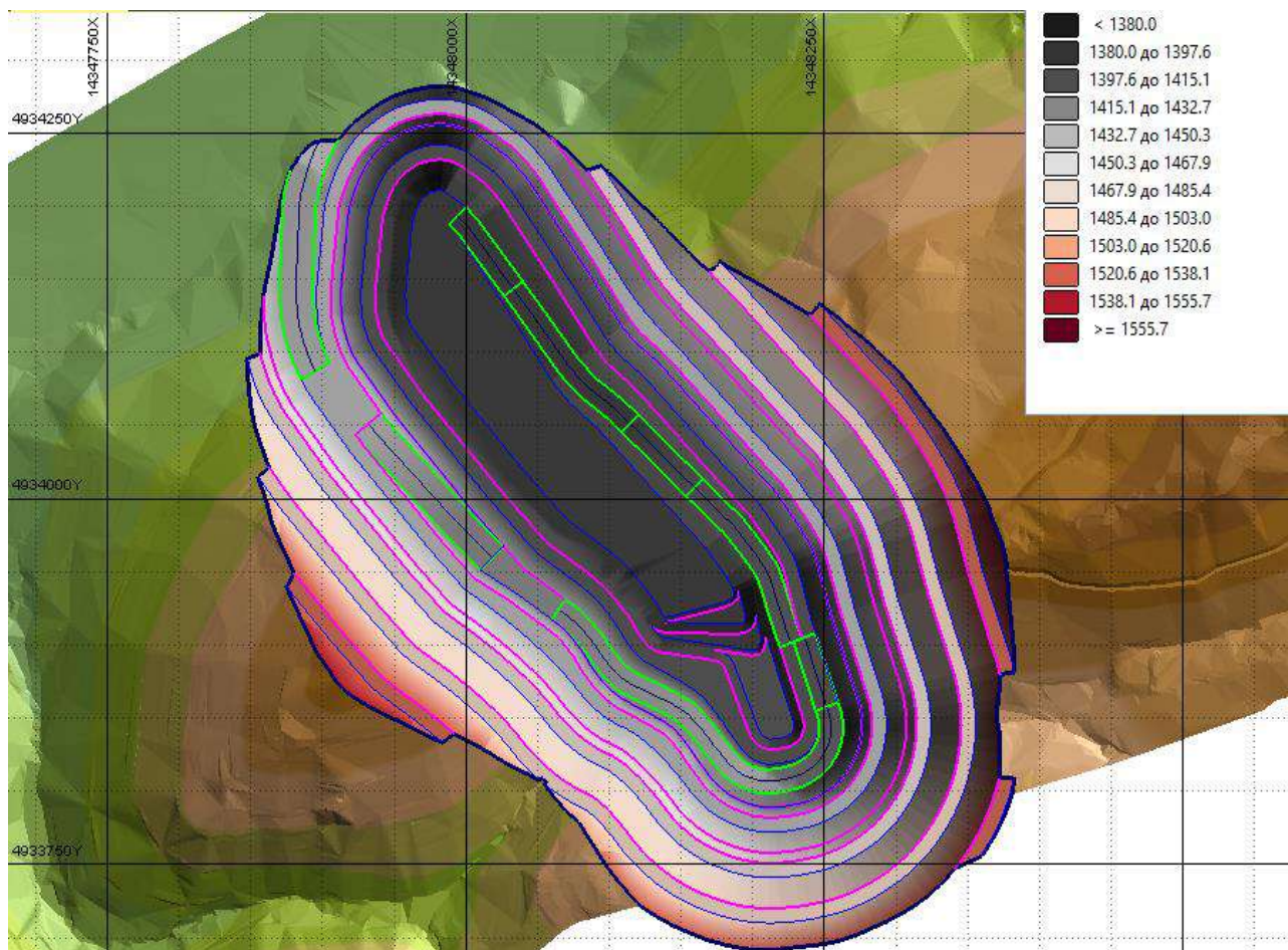
Рис. 1.8 – План Карьера на конец отработки
