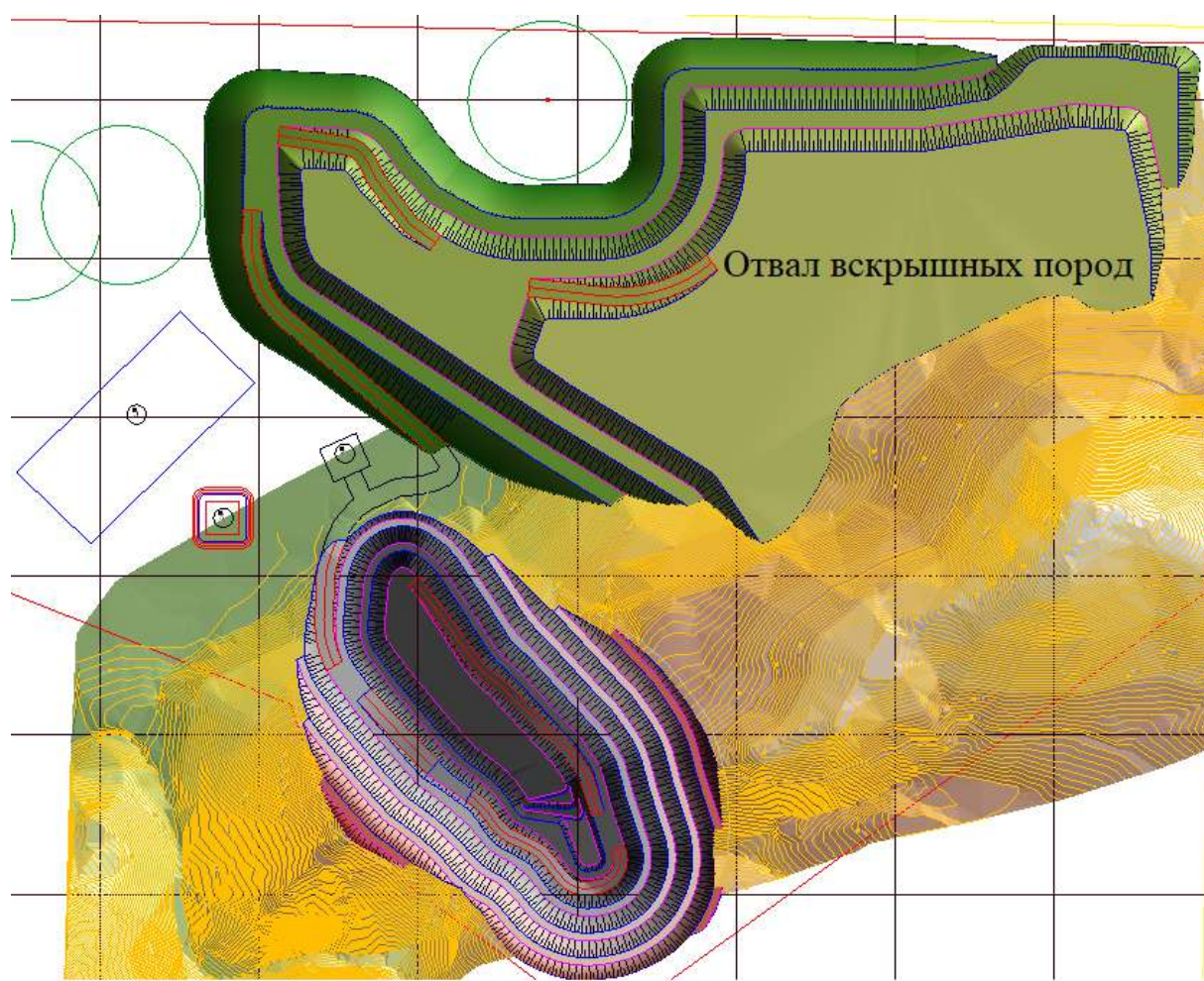
Рис. 1.9 – Проектный контур Отвала вскрышных пород
