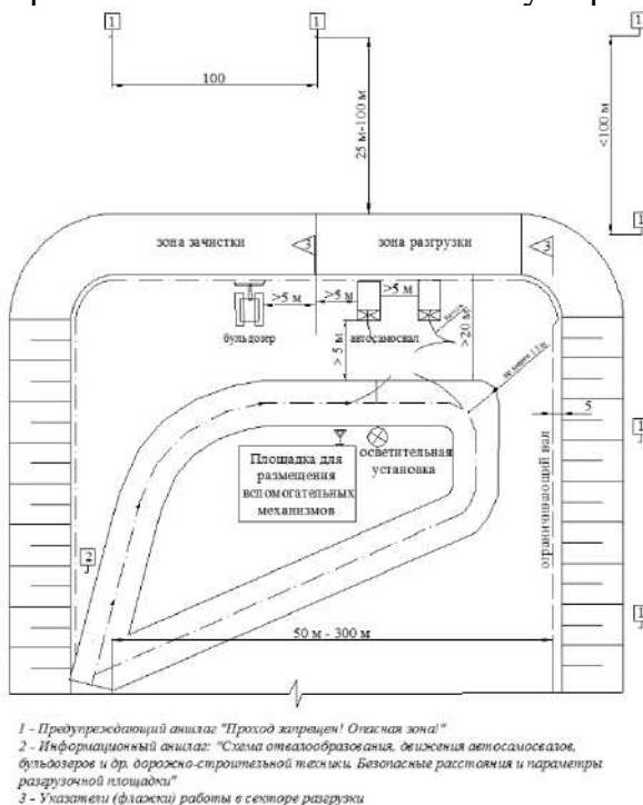
Рис. 1.10. – Схема бульдозерного отвалобразования
