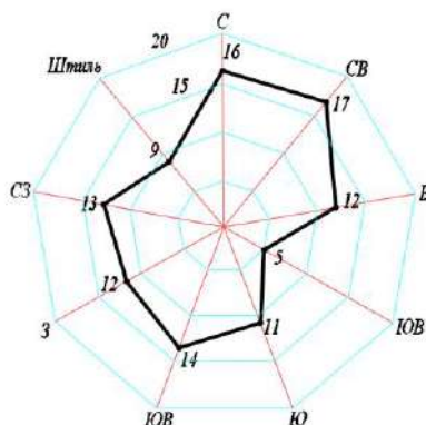
Рис. 1.7 – Роза ветров
