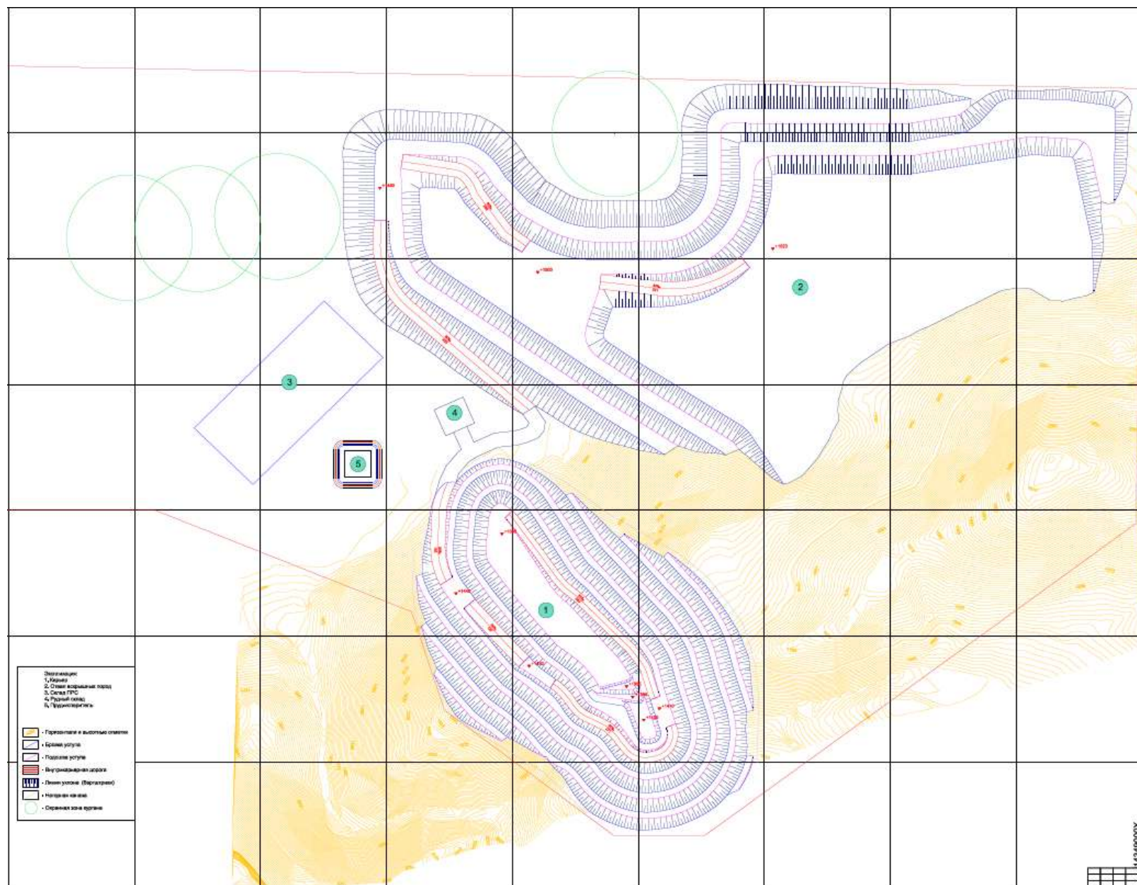
Рис. 1.4 – Генеральный план месторождения
