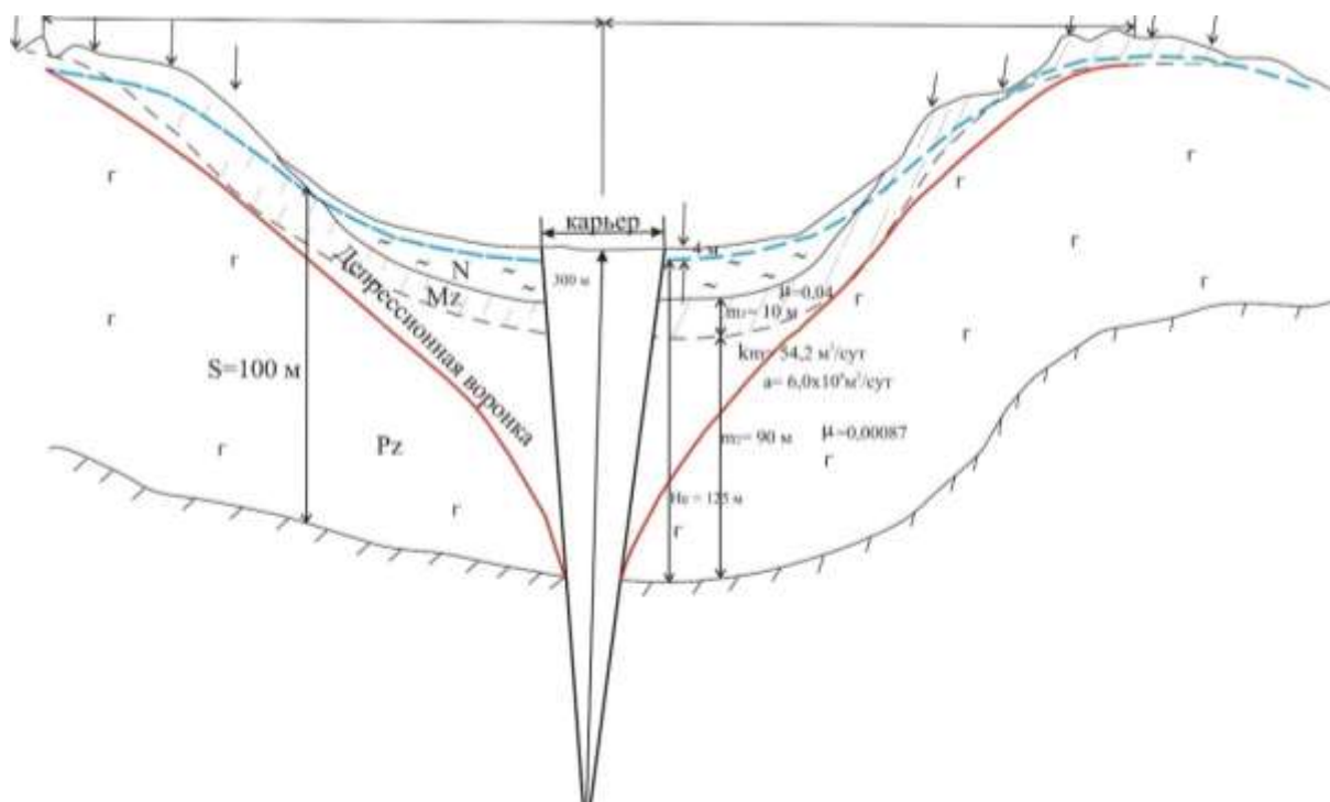
Схематический разрез к расчету водопритоков
