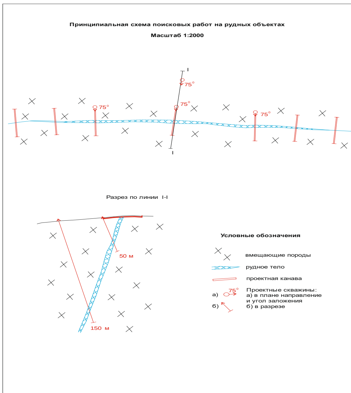
Рисунок 4 – Принципиальная схема работ на рудном объекте
