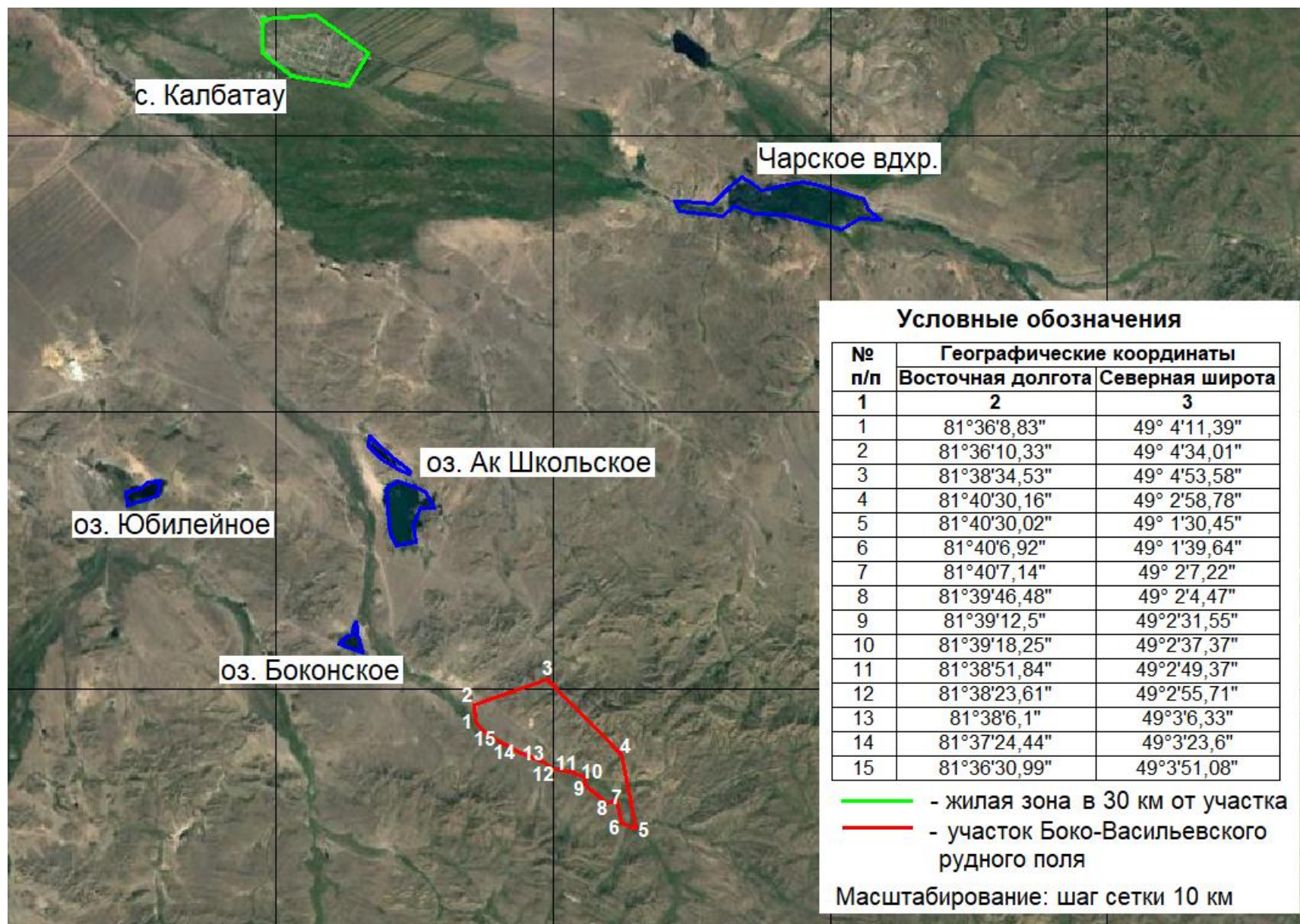
Рисунок 10 – Ситуационная карта-схема рассматриваемого объекта
