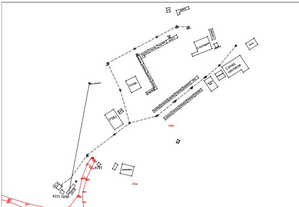
Рисунок 7 – Схема размещения на участке разведки РМЦ, склада инвентаря, столовой и кернорезки
