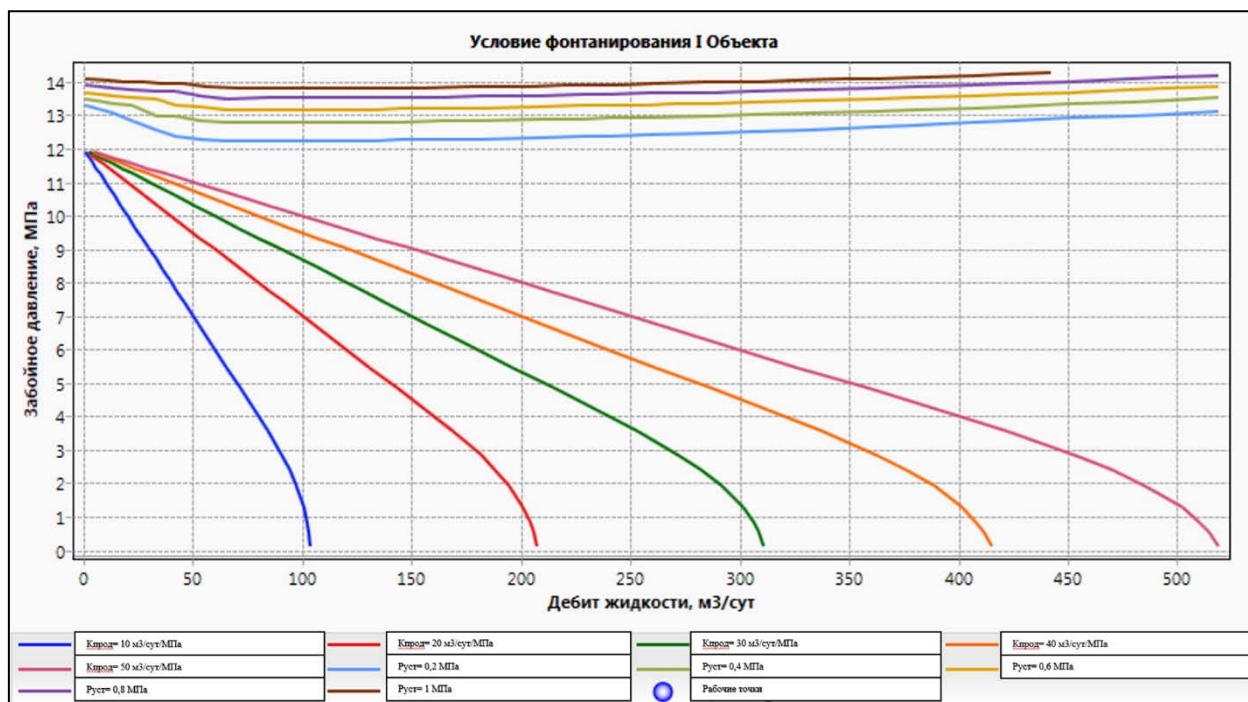
Рисунок 6.1.1 – Согласование работы I Объекта и подъемника с внутренним диаметром 62 мм
