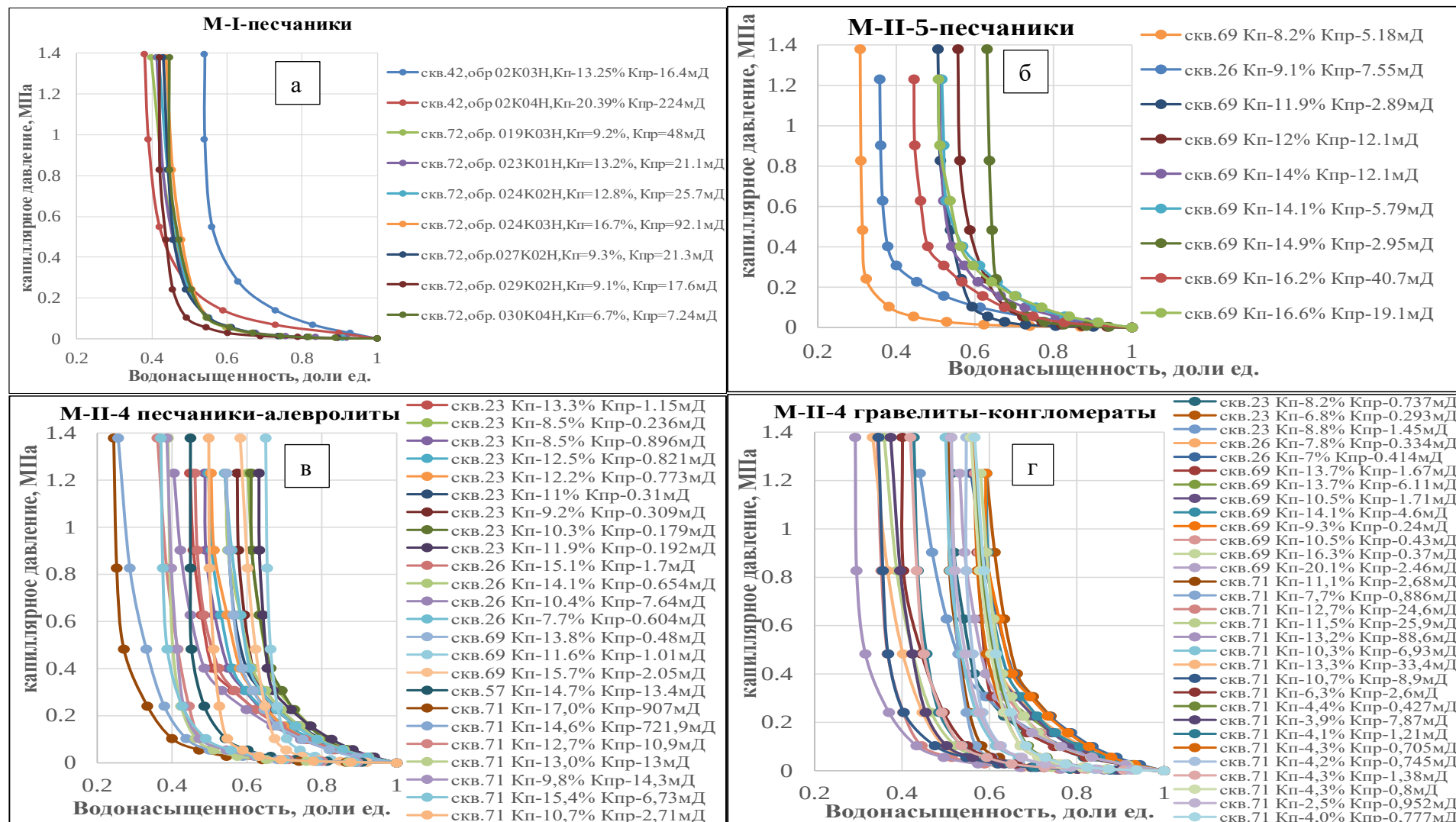
Рисунок 2.4.1 - Кривые капиллярного давления по горизонтам: а) М-I; б) М-II-5; в) М-II-4 для песчаников и алевролитов; г) М-II-4 для гравелитов и конгломератов
