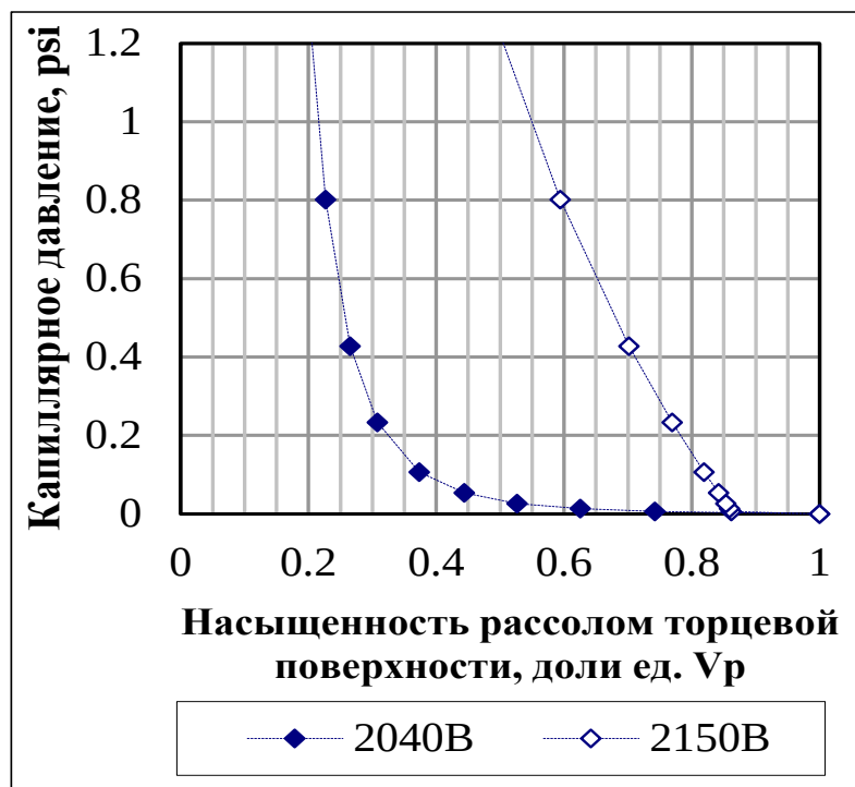
Рисунок 2.4.2 - Кривые капиллярного давления, скв. №23, горизонт М-II-4, песчаники
