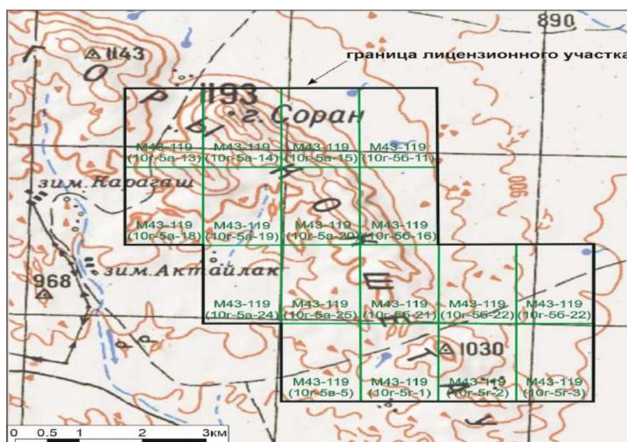
Рисунок 4. Схема участка Саран на топографической основе
