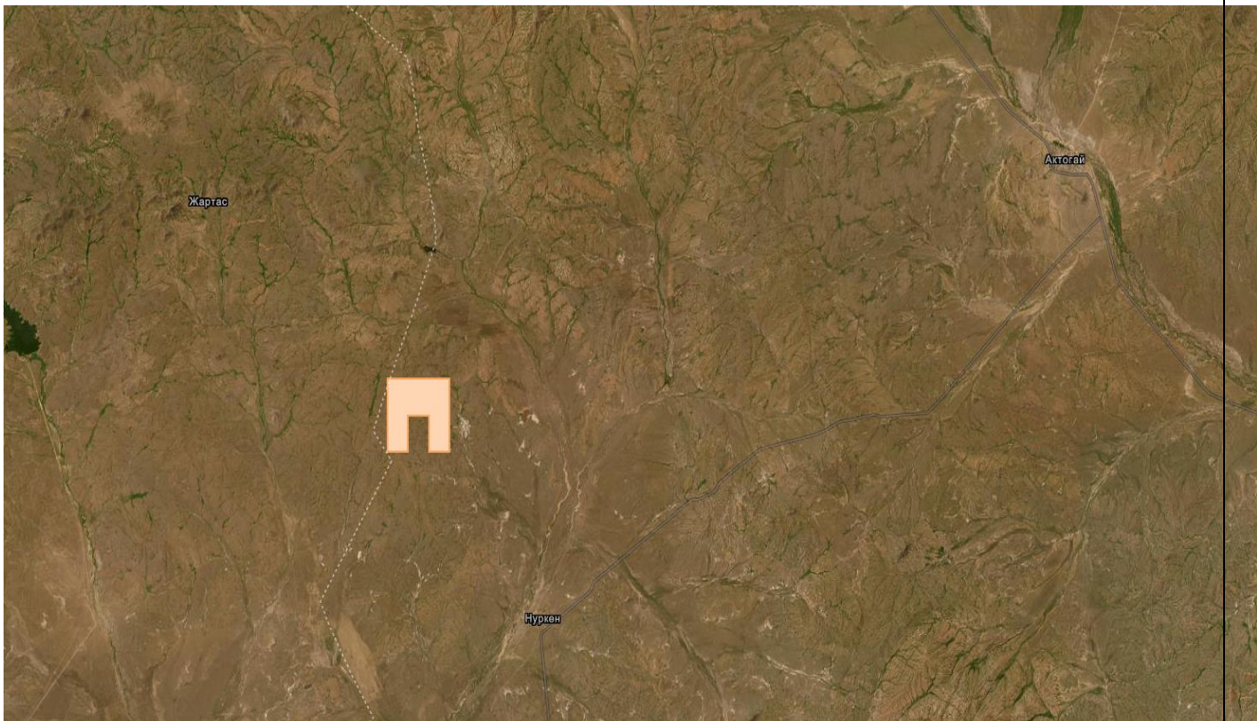
Рис 1.2 Космоснимок участка
