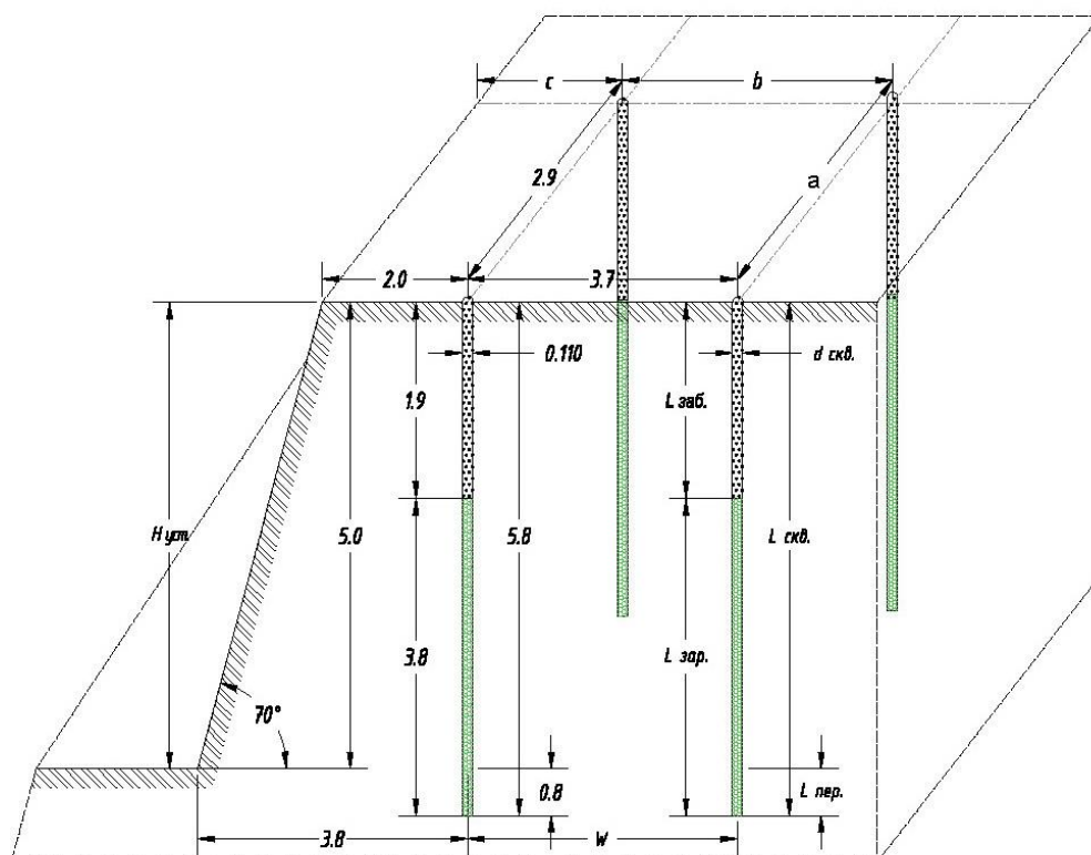
Рисунок 3-6 - Параметры конструкции скважинного заряда на рудных уступах
