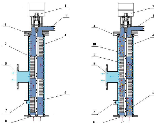
Рисунок 4-2-Процесс очистки в фильтрах ССФ
