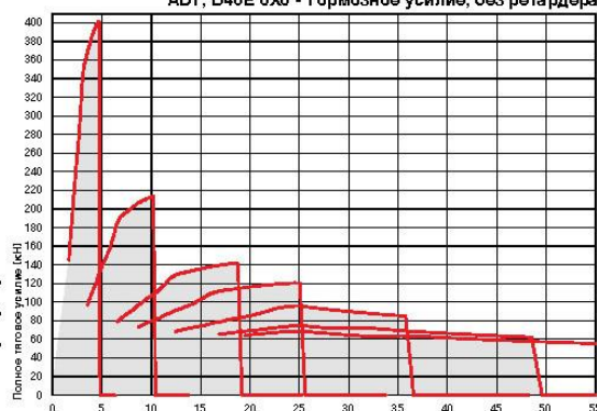
ADT, B40E 6X6 - Тормозное усилие, без ретардера
