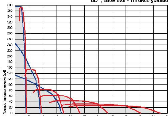
ADT, B40E 6X6 - Тяговое усилие
