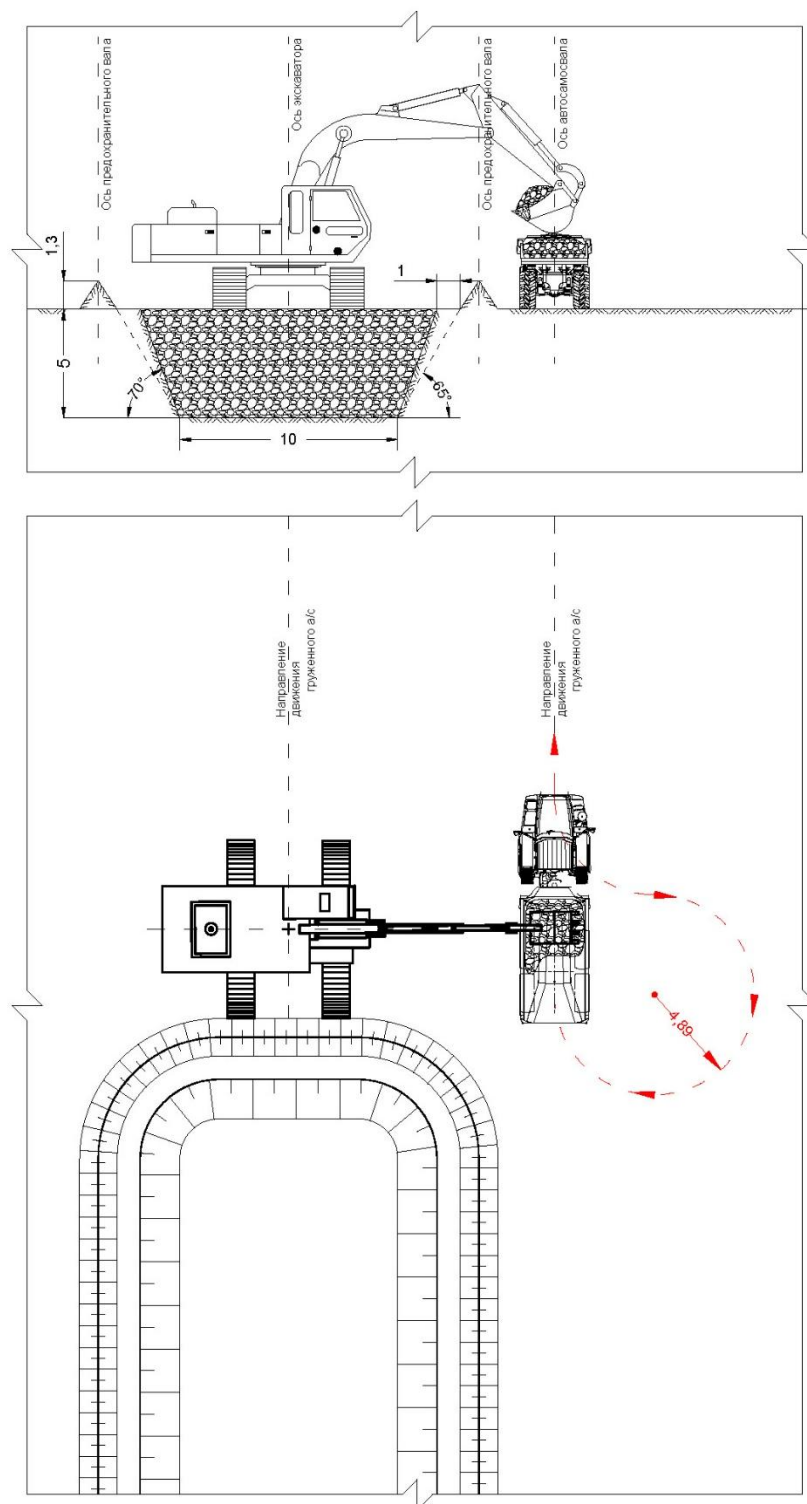
Рисунок 3-3 - Схема проходки траншеи (сезда) гидравлическим экскаватором (обратная лопата) с нижним черпанием и погрузкой в автосамосвалы на уровне стояния экскаватора, с петлевым разворотом
