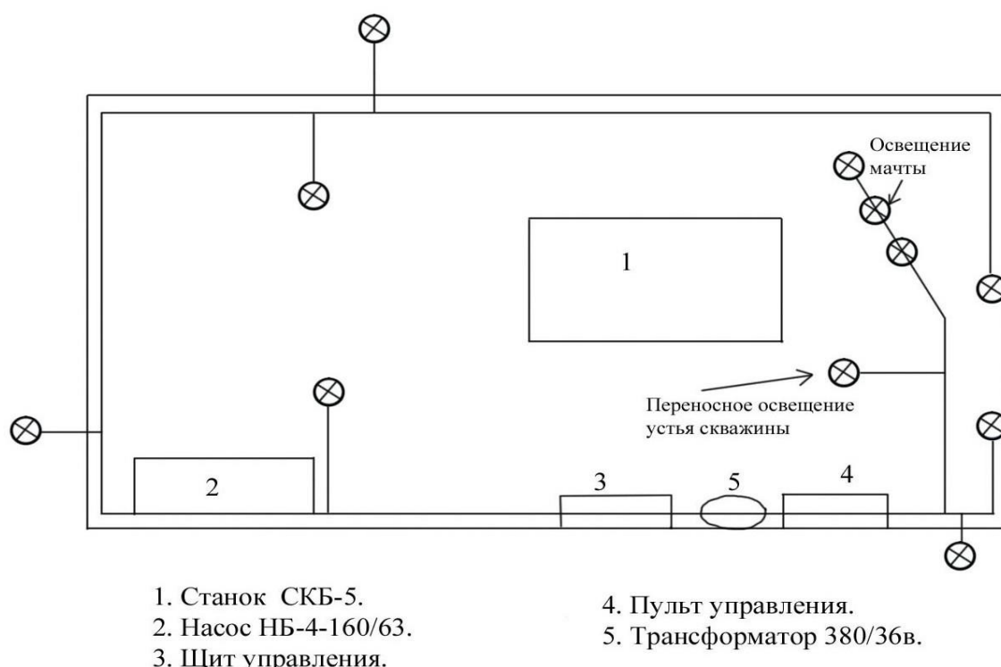
Схема освещения бурового агрегата
