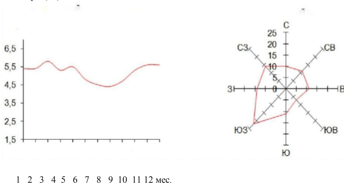
Рис. 2-2. Характеристика ветра по метеостанциям
