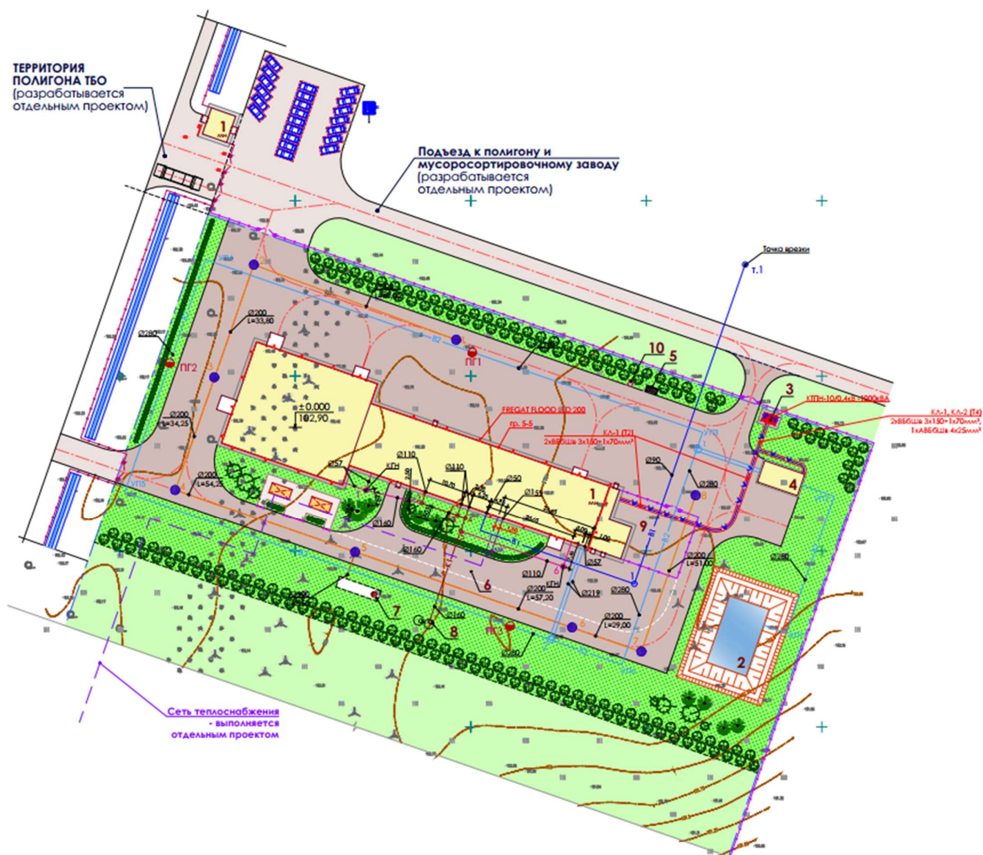
Рис. 1.5.1.2 Карта-схема объекта с указанием границ существующих объектов и указанием проектируемых зданий, сооружений
