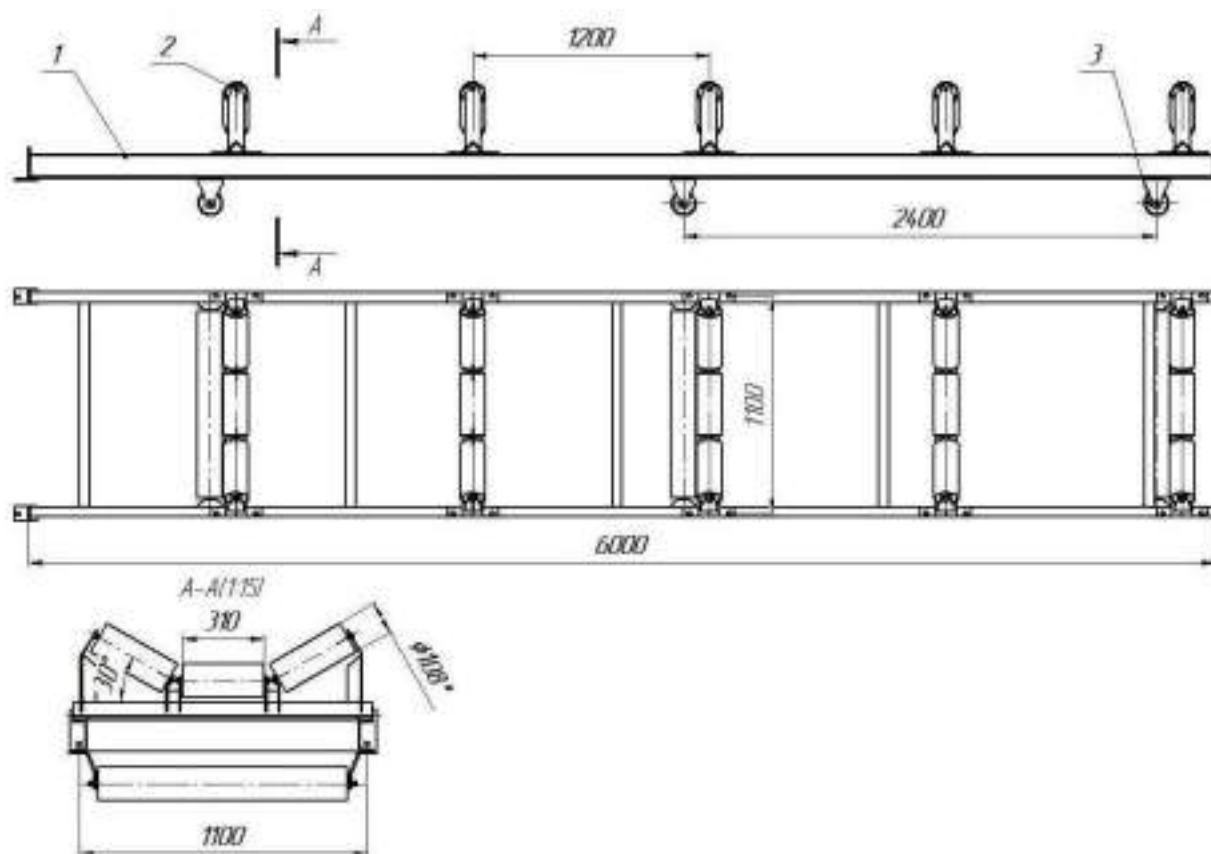
Рис. 5 КЛ800.50.17.03.00.00.000-01 СБ Линейная секция
