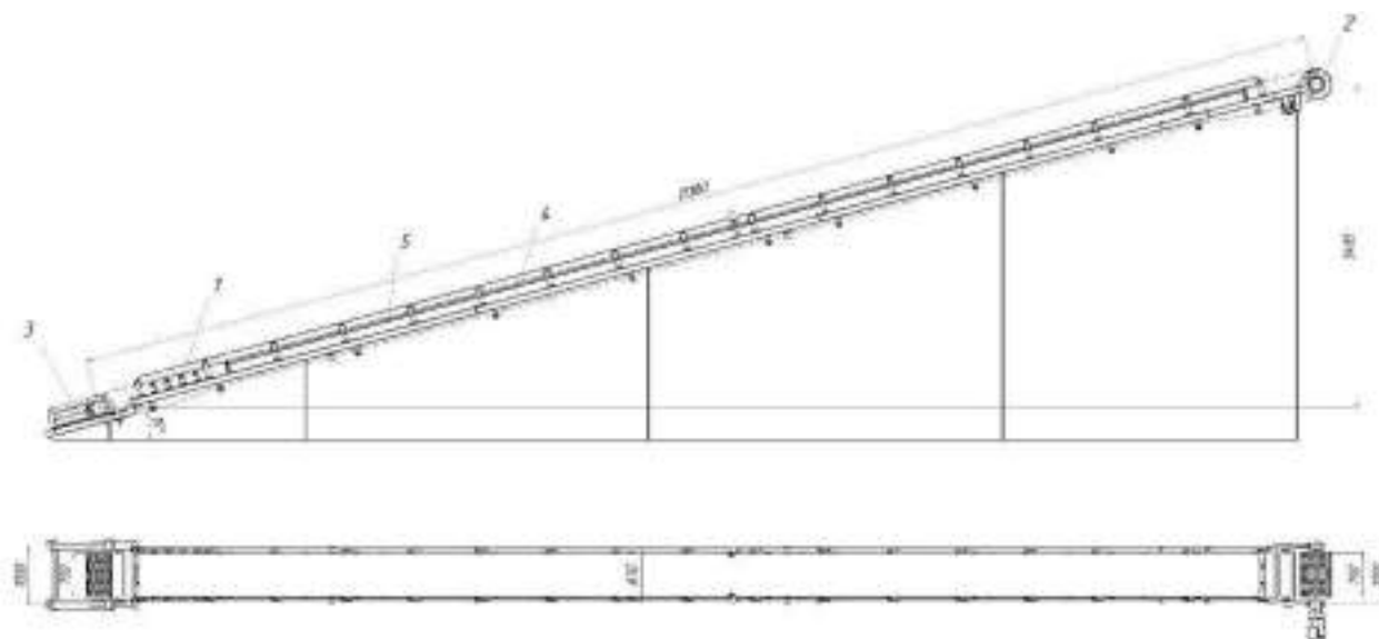
Рис.1 КЛ650.21,38.00.00.00.000 СБ Ленточный конвейер
