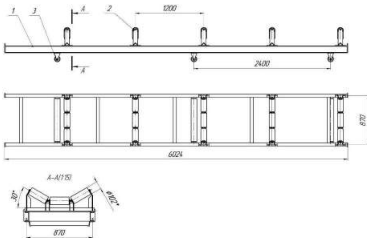
Рис. 5 КЛ650.20.03.00.00.000-01 СБ Линейная секция
