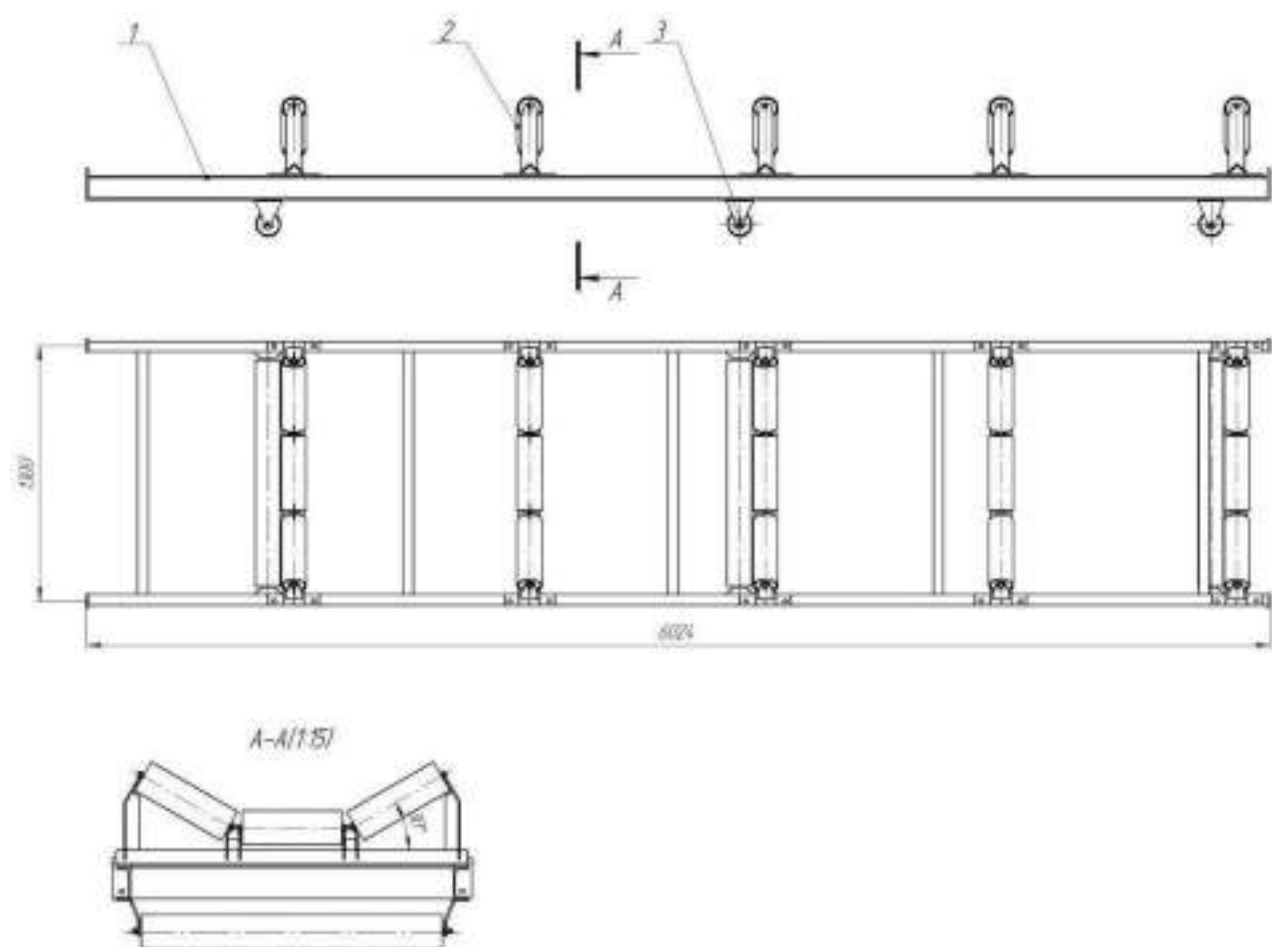
Рис. 5 КЛ1000.41,2.03.00.00.000-01 СБ Линейная секция
