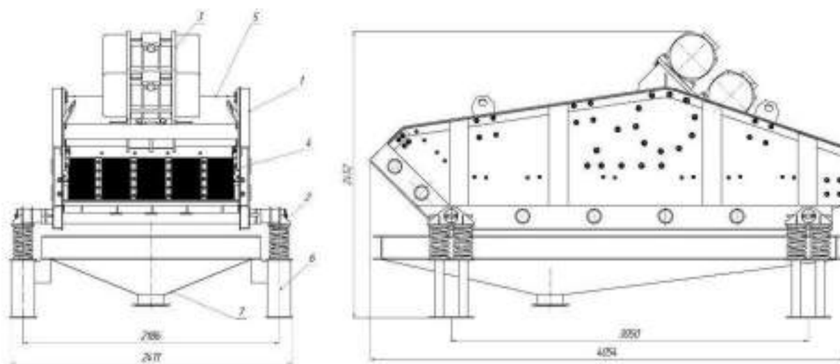
Рис.1 1 Корпус; 2 Опора; 3 Вибратор; 4 Гайка; 5 Под-вибраторная балка 6 Опора пружинная; 7 Вибрационная тарелка
