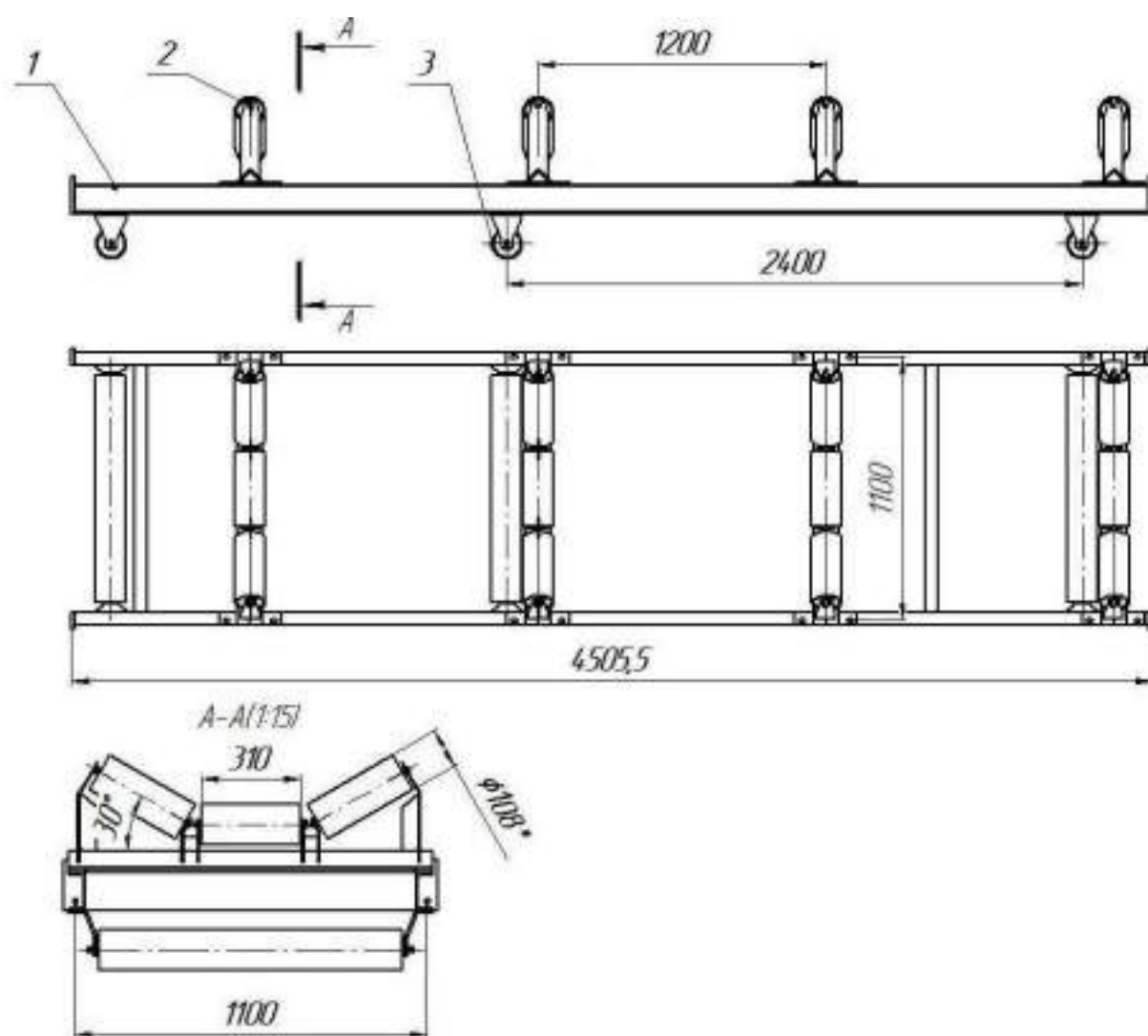
Рис.6 КЛ800.50.17.03.00.00.000-08 СБ Линейная секция
