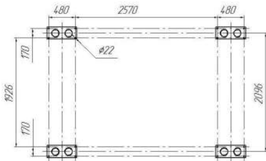
Расположения отверстий под монтажные болты
