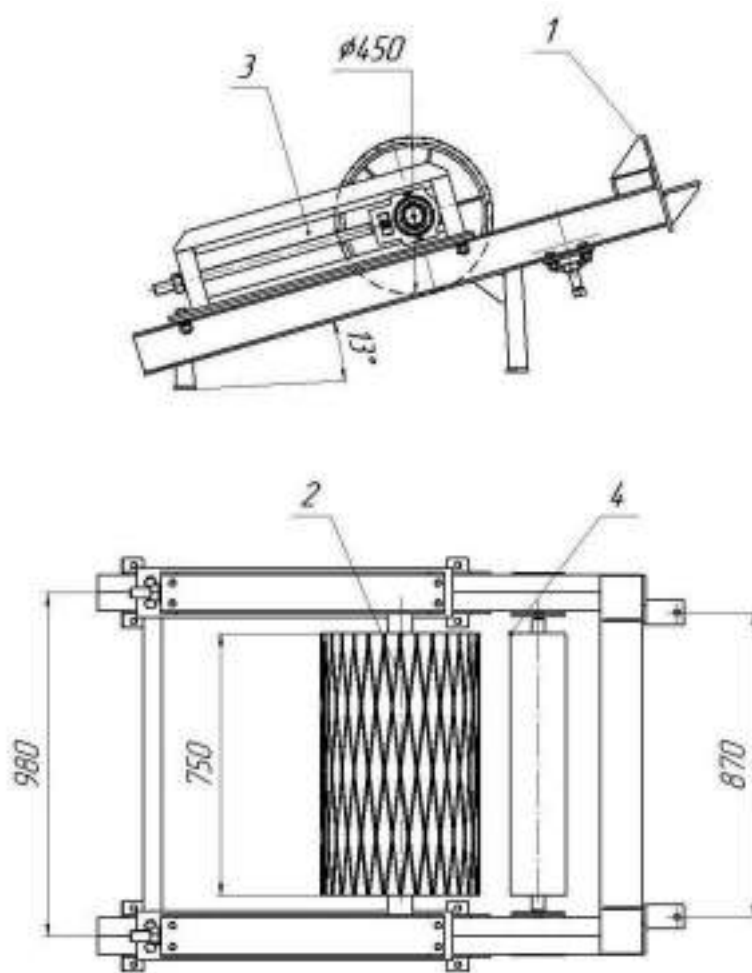
Рис.3 КЛ650.22,42.02.00.00.000 СБ Натяжной барабан
