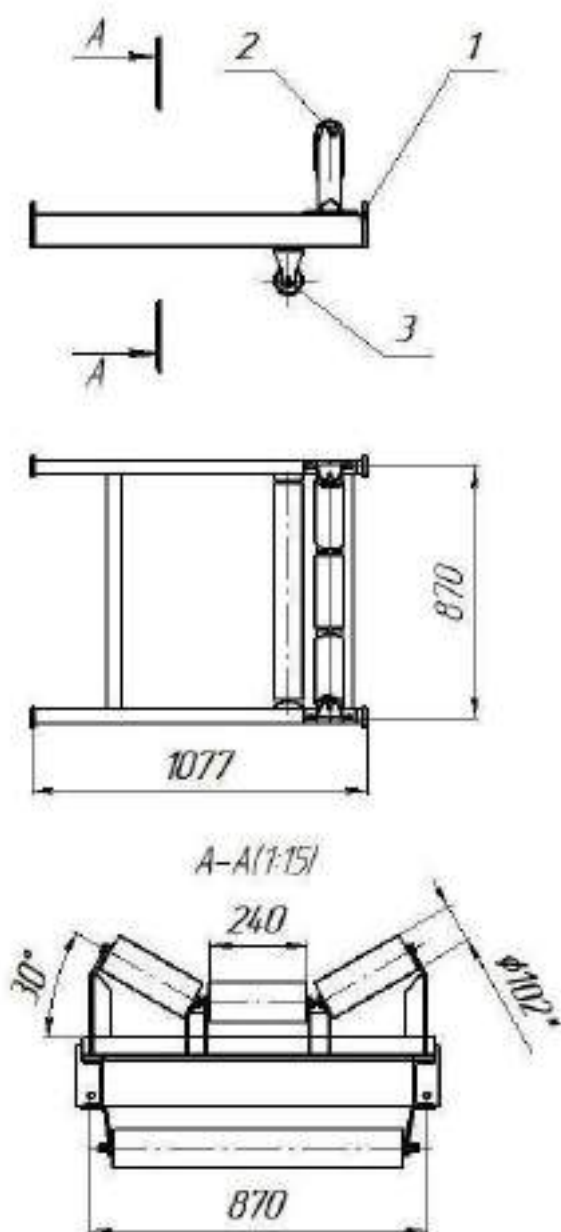
Рис. 5 КЛ650.9,68.03.00.00.000-02 СБ Линейная секция
