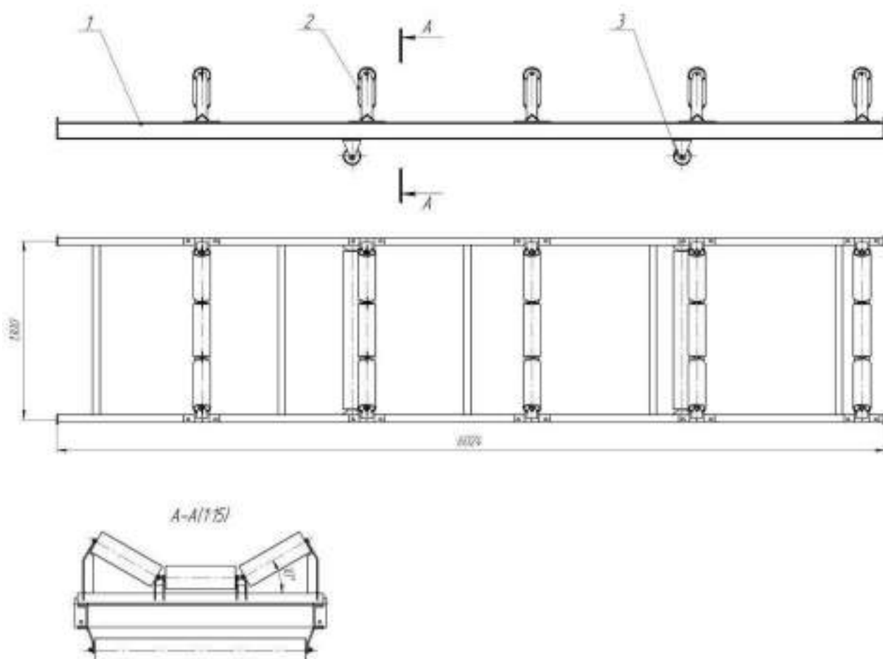
Рис.7 КЛ1000.41,2.03.00.00.000-03 СБ Линейная секция
