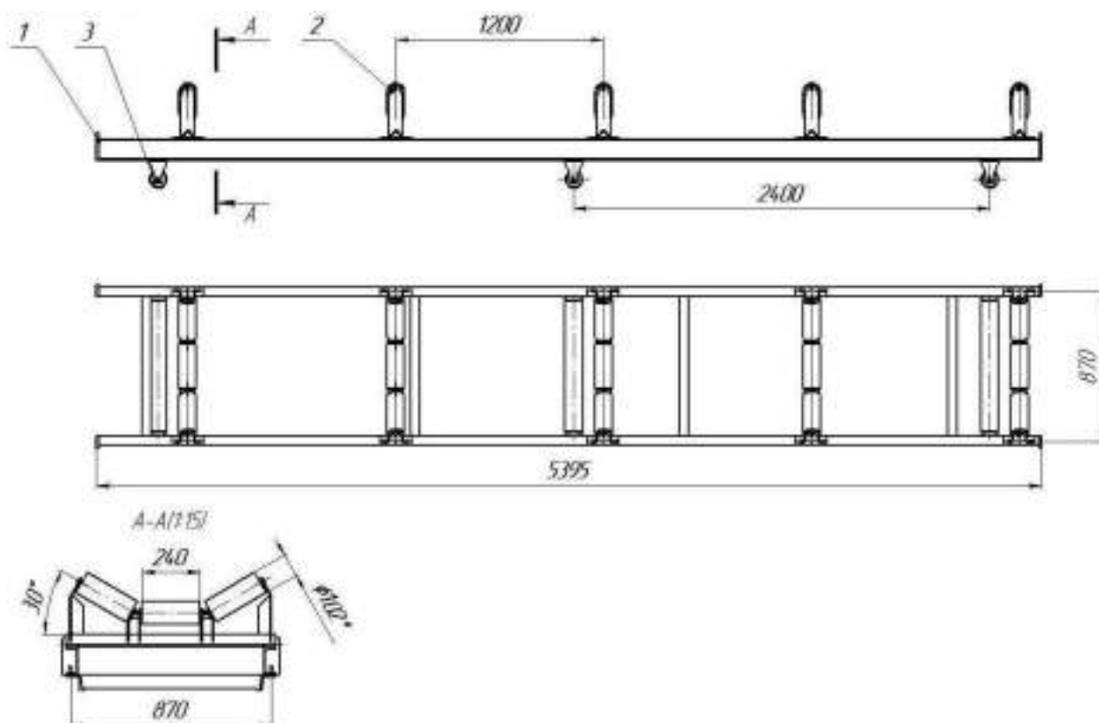
Рис.6 КЛ650.20.03.00.00.000-02 СБ Линейная секция
