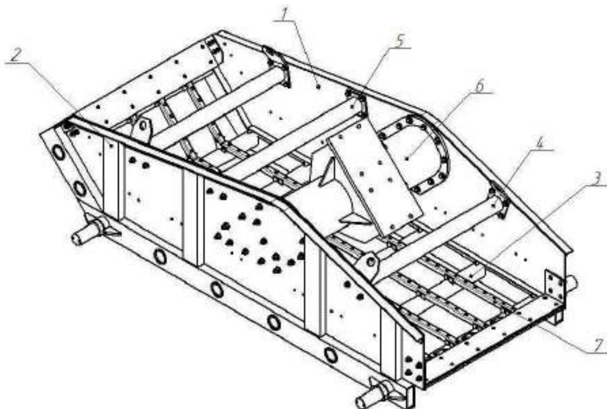
Рис.3 Короб 1,2 - ГВЧ 500.01.00.00.00.001 Боковина 3- Труба; 4- Связь балки; 5- Связь балки 6- Под-вибраторная балка; 7- Подситники
