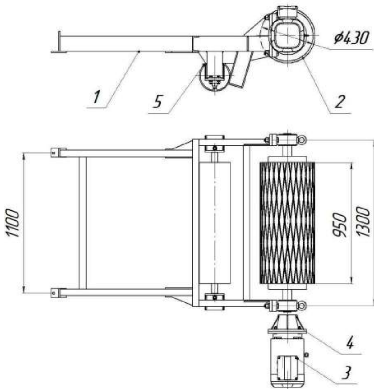
Рис. 2 КЛ800.23,94.01.00.00.000 СБ Приводной барабан
