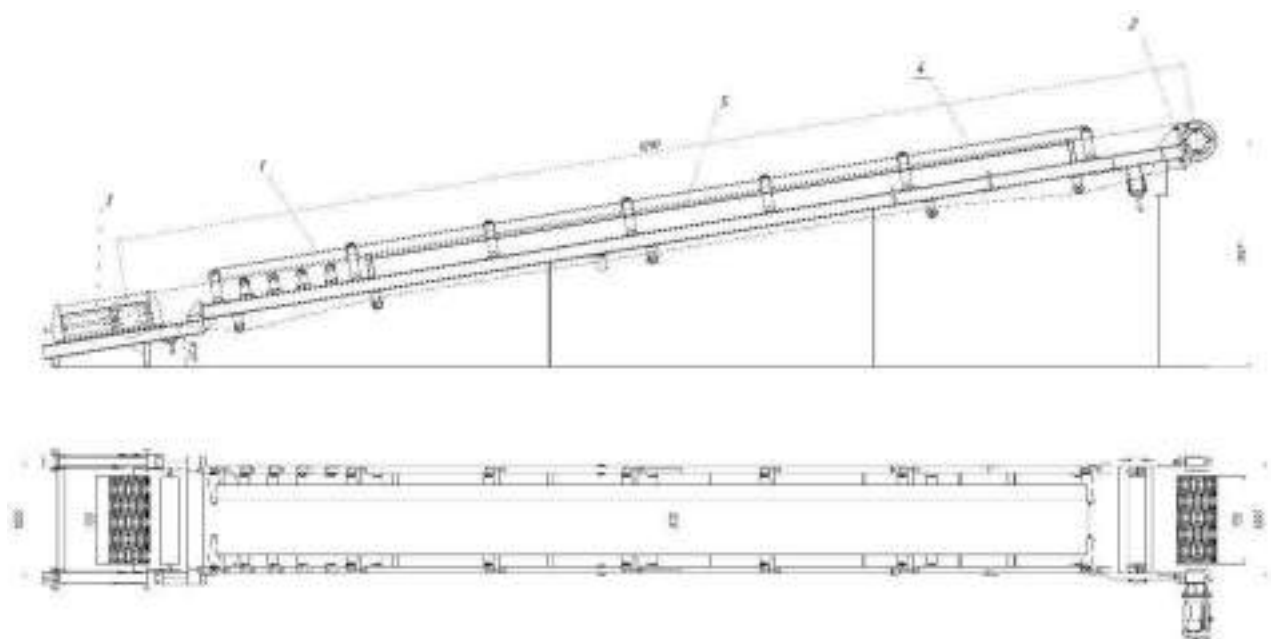
Рис.1 КЛ650.9,29.00.00.00.000 СБ Ленточный конвейер
