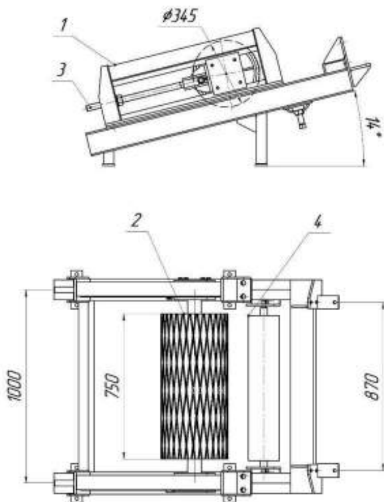
Рис.3 КЛ650.12,6.02.00.00.000 СБ Натяжной барабан
