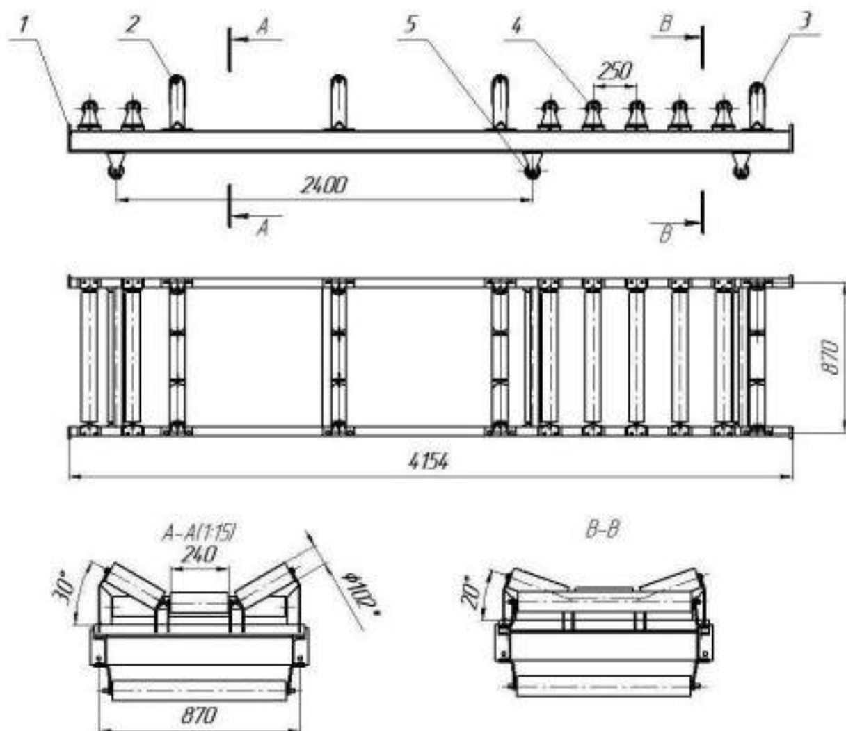
Рис. 4 КЛ650.6,6.03.00.00.000 СБ Линейная секция
