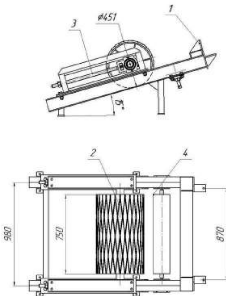
Рис.3 КЛ650.21,38.02.00.00.000 СБ Натяжной барабан
