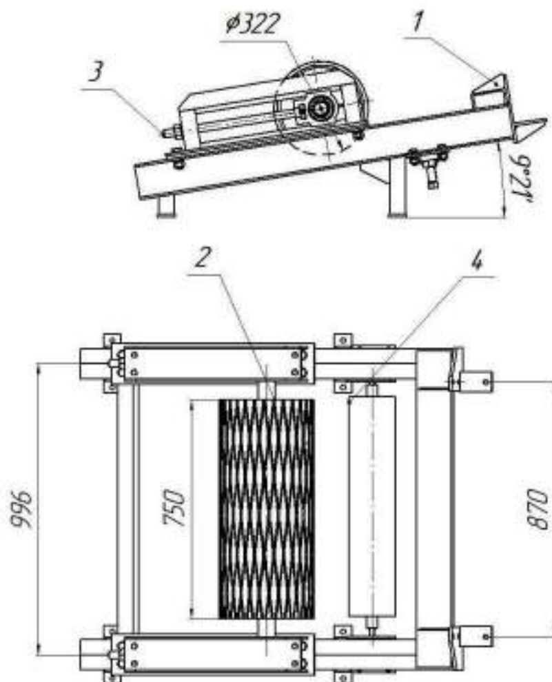
Рис.3 КЛ650.9,68.02.00.00.000 СБ Натяжной барабан
