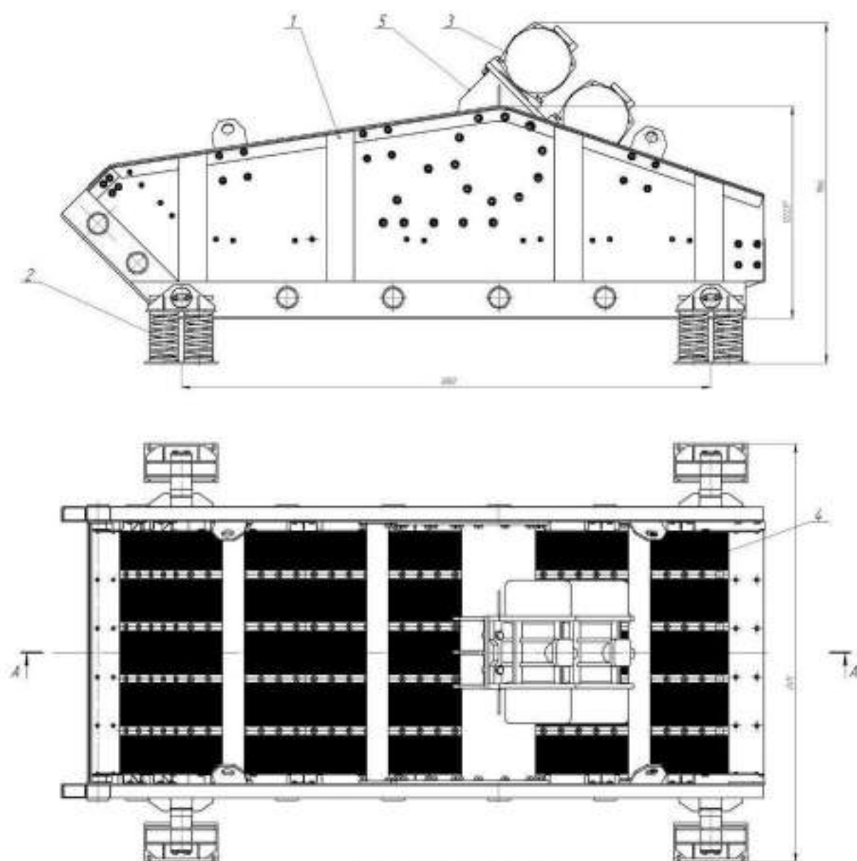
Рисунок 1. Общий вид грохота 1- корпус, 2-опора, 3-вибратор 4- Сито, 5- Подвижная рама
