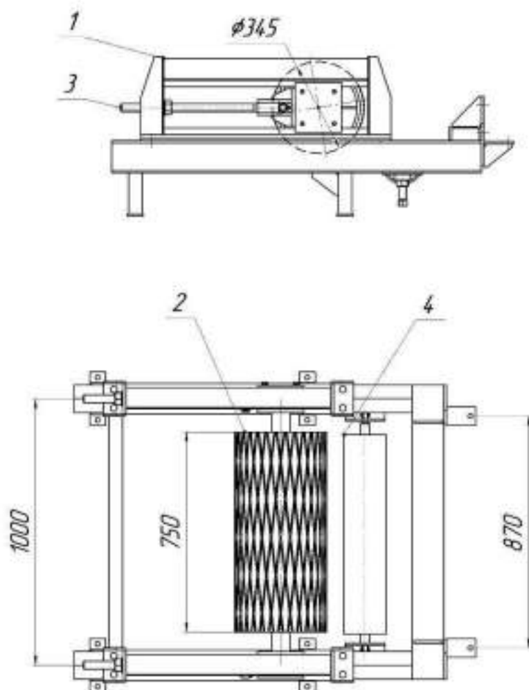
Рис.3 КЛ650.9,68.02.00.00.000 СБ Натяжной барабан
