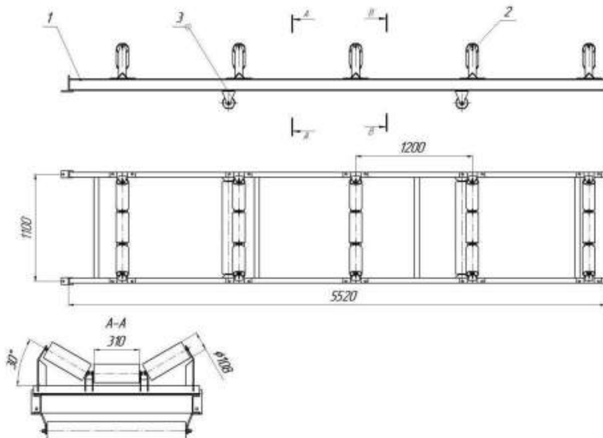
Рис.6 КЛ800.23,94.03.00.00.000-02 СБ Линейная секция
