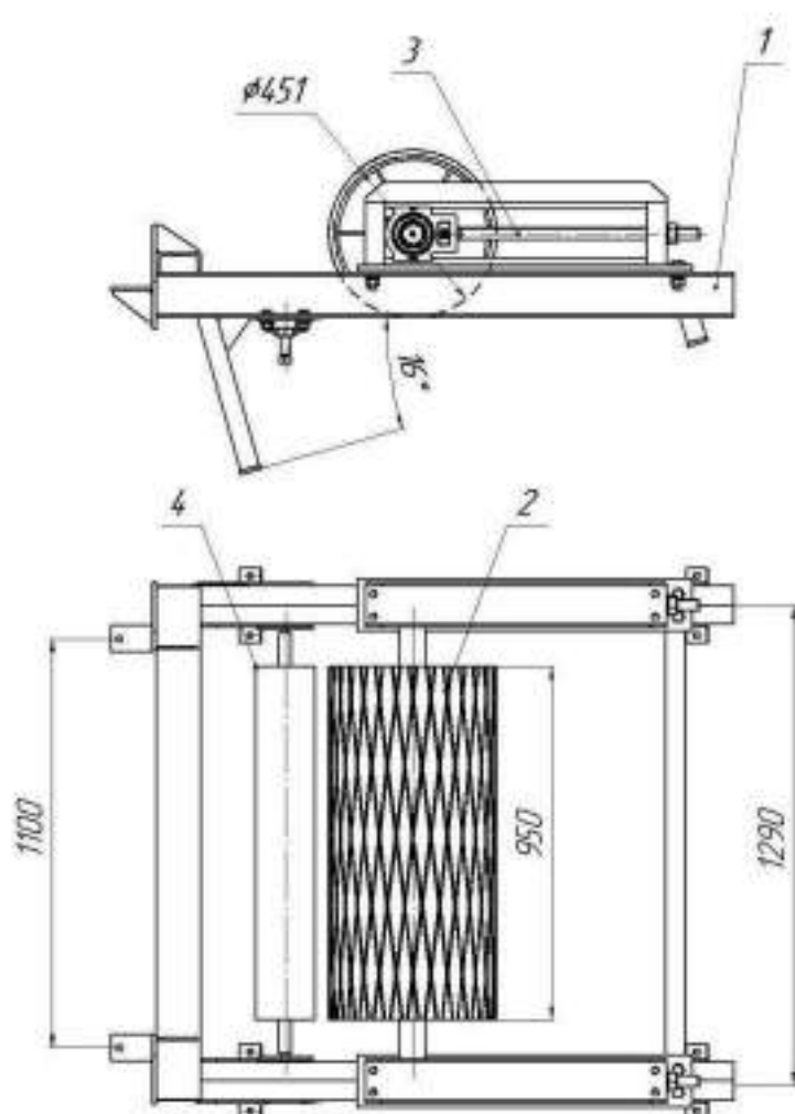
Рис.3 КЛ800.23,94.02.00.00.000 СБ Натяжной барабан
