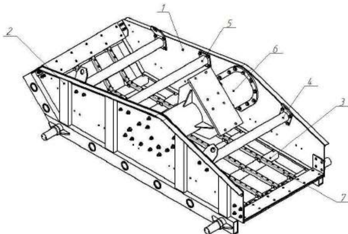
Рис.3 Короб 1,2 - ГВЧ 500.01.00.00.00.001 Боковина 3- Труба; 4- Связь балка; 5- Связь балка 6- Под-вибраторная балка; 7- Подситники
