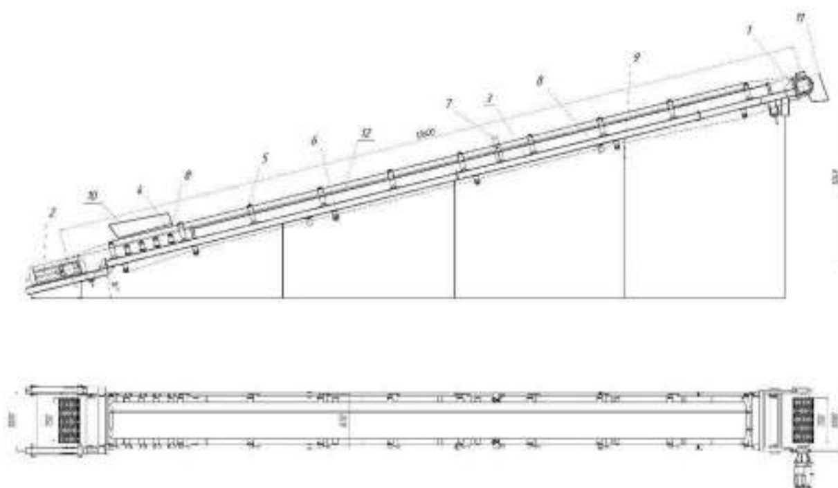
Рис.1 КЛ650.12,6.00.00.000 СБ Ленточный конвейер
