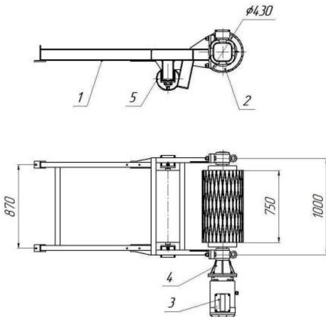
Рис. 2 КЛ650.15,73.01.00.00.000 СБ Приводной барабан
