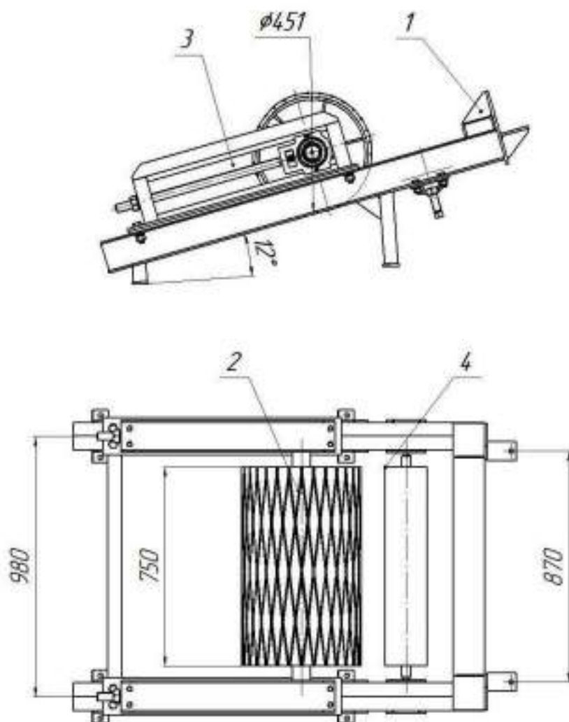
Рис.3 КЛ650.20.02.00.00.000 СБ Натяжной барабан
