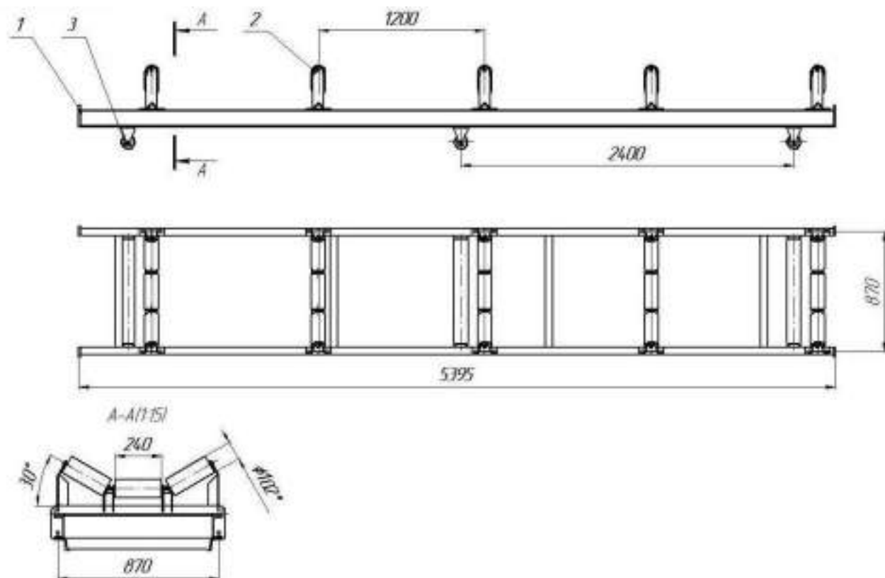
Рис.6 КЛ650.20.03.00.00.000-02 СБ Линейная секция
