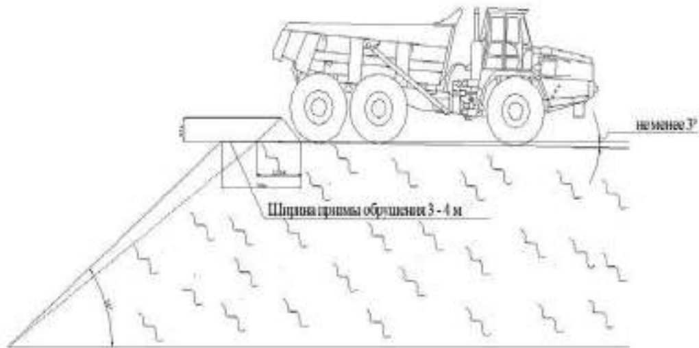
рисунки 6: Схема бульдозерного отвалообразования
