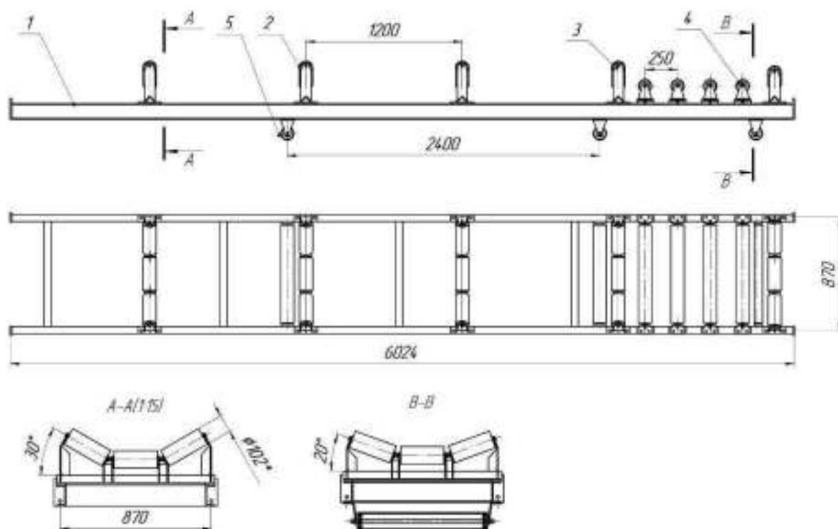
Рис. 4 КЛ650.20.03.00.00.000 СБ Линейная секция
