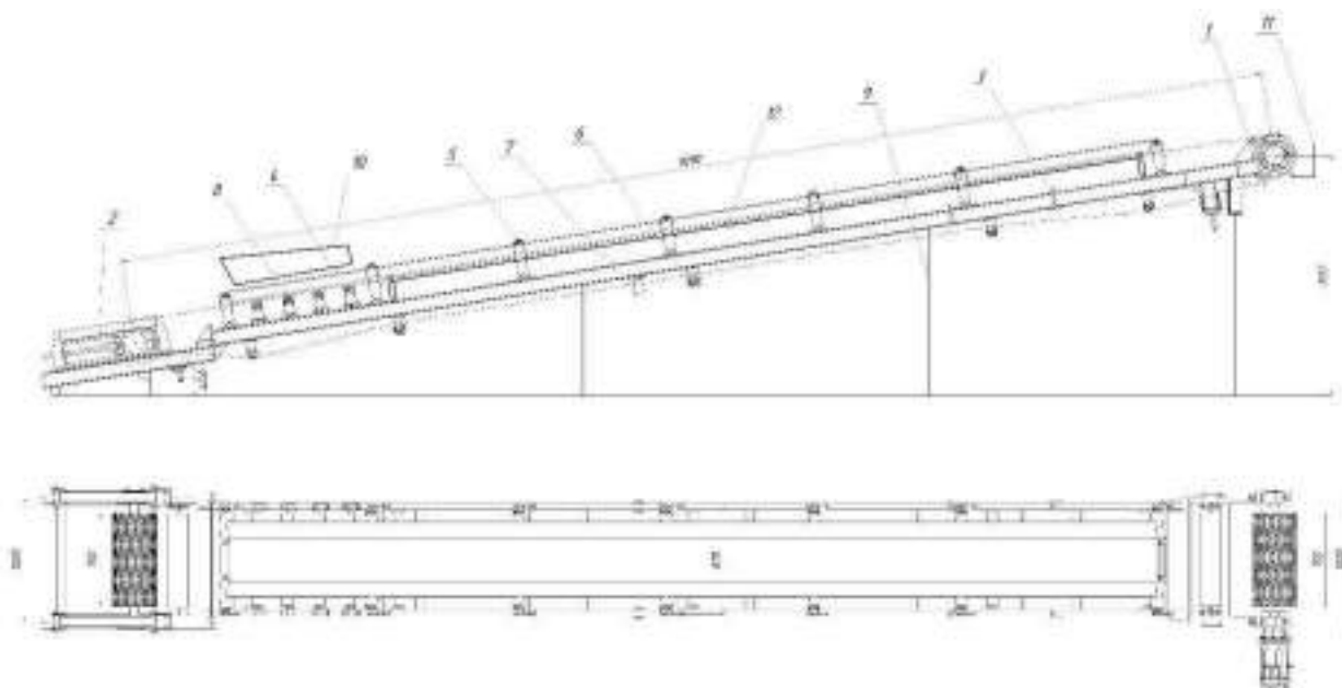
Рис.1 КЛ650.9,29.00.00.000 СБ Ленточный конвейер
