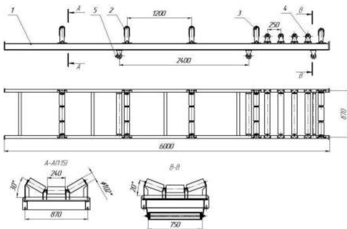
Рис. 4 КЛ650.12,6.03.00.00.000 СБ Линейная секция
