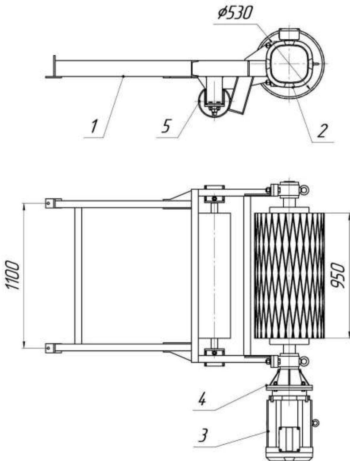
Рис. 2 КЛ800.50.17.01.00.00.000 СБ Приводной барабан
