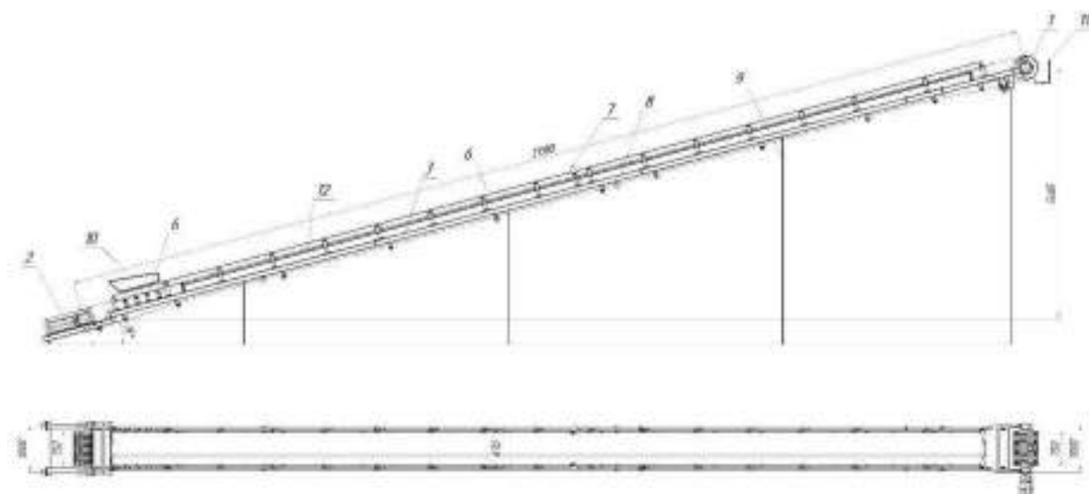
Рис.1 КЛ650.21,38.00.00.000 СБ Ленточный конвейер
