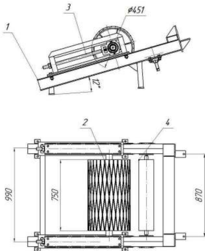
Рис.3 КЛ650.20.02.00.00.000 СБ Натяжной барабан
