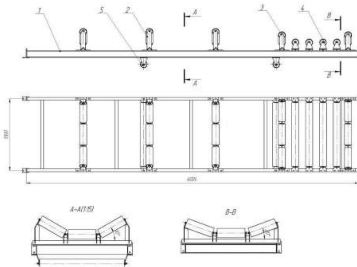
Рис. 4 КЛ1000.41,2.03.00.00.000 СБ Линейная секция
