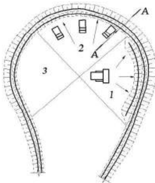
рисунки 6: Схема бульдозерного отвалообразования
