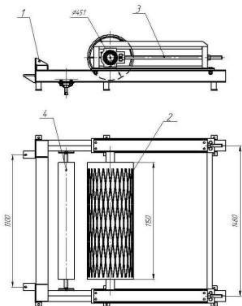
Рис.3 КЛ1000.41,2.02.00.00.000 СБ Натяжной барабан
