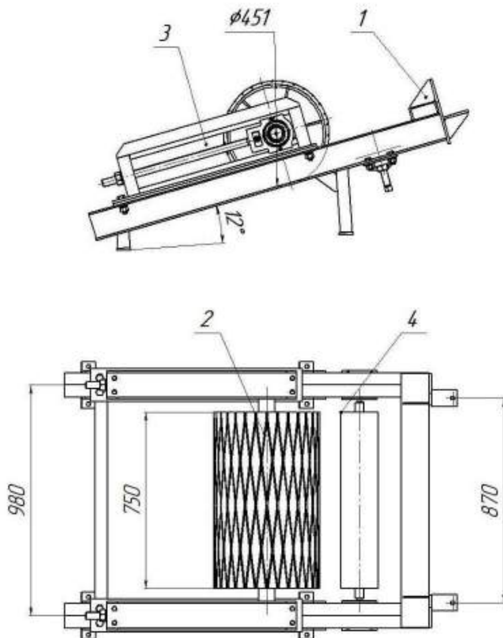
Рис. 3 КЛ650.20.02.00.00.000 СБ Натяжной барабан
