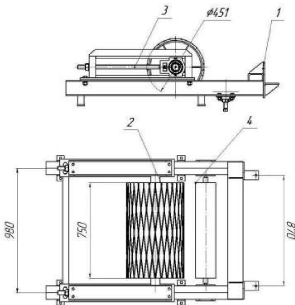
Рис.3 КЛ650.15,73.02.00.00.000 СБ Натяжной барабан
