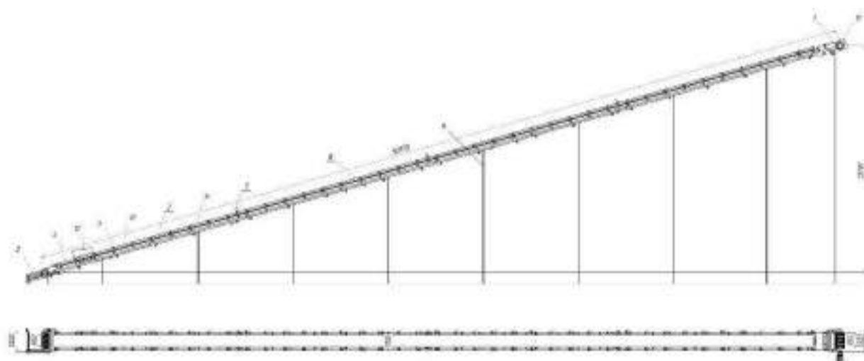
Рис.1 КЛ800.15.17.00.00.000 СБ Ленточный конвейер
