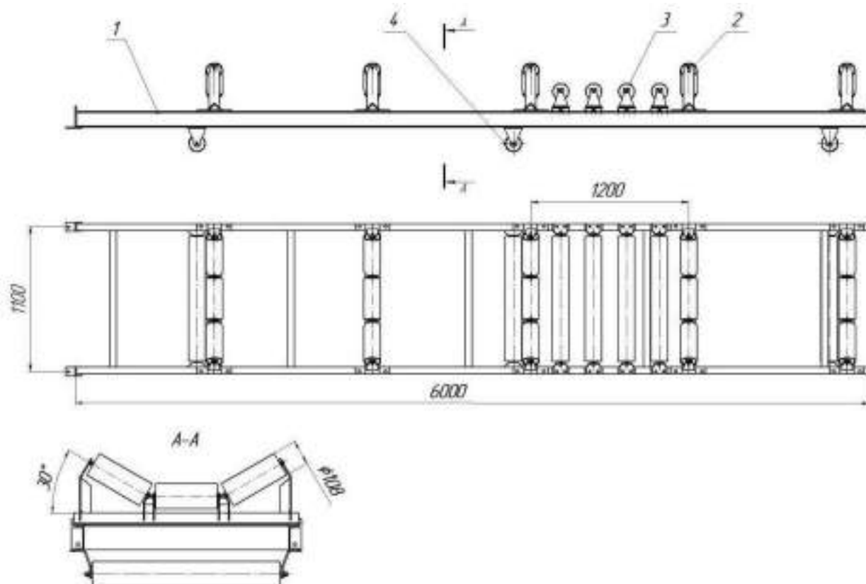
Рис. 5 КЛ800.23,94.03.00.00.000-01 СБ Линейная секция
