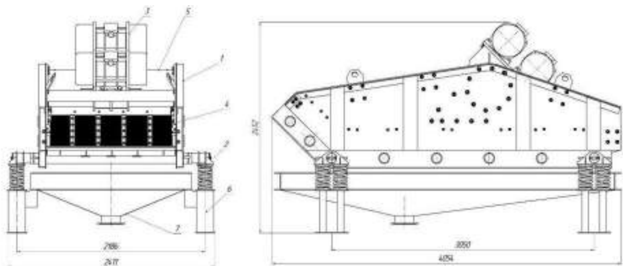
Рис.1 1 Короб; 2 Опора; 3 Вибратор; 4 Сито; 5 Под-вибраторная балка 6 Опора грохота; 7 Выгрузная воронка
