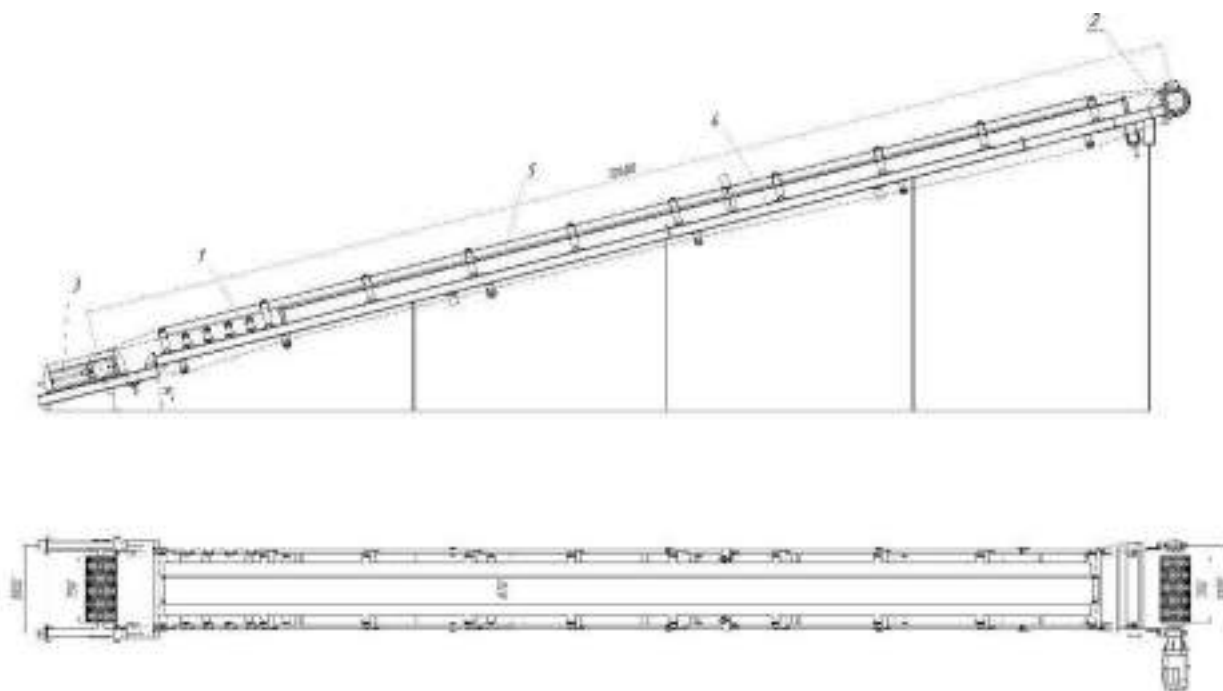
Рис.1 КЛ650.12,6.00.00.00.000 СБ Ленточный конвейер
