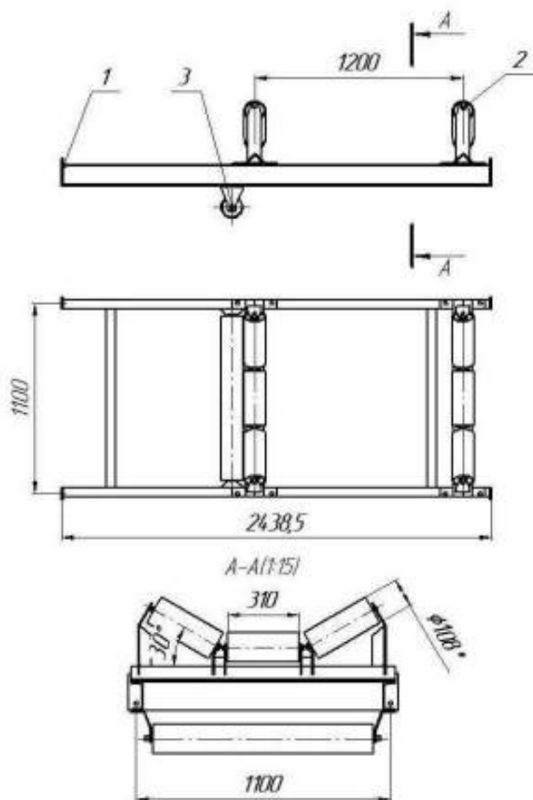
Рис.6 КЛ800.46,94.03.00.00.000-02 СБ Линейная секция
