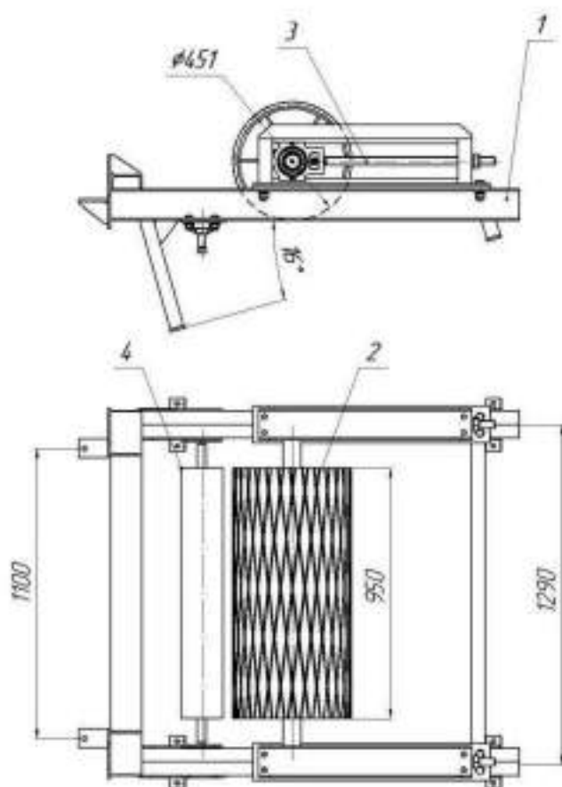
Рис.3 КЛ800.50.17.02.00.00.000 СБ Натяжной барабан
