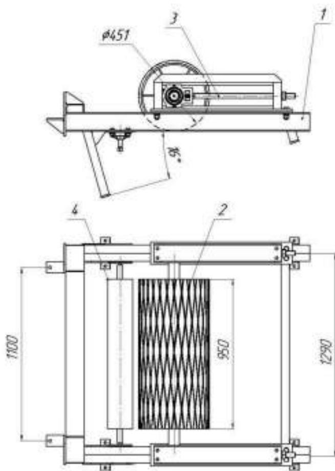
Рис.3 КЛ800.50.17.02.00.00.000 СБ Натяжной барабан
