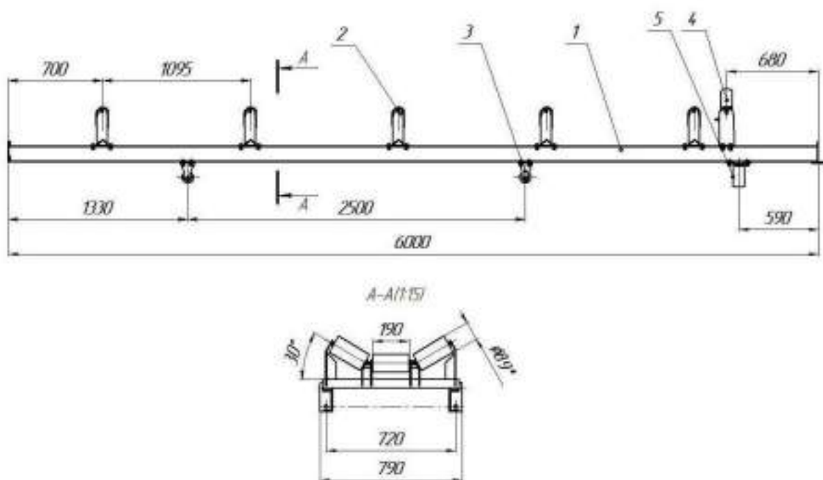
Рис.6 КЛ500.25.03.00.00.000-02 СБ Линейная секция
