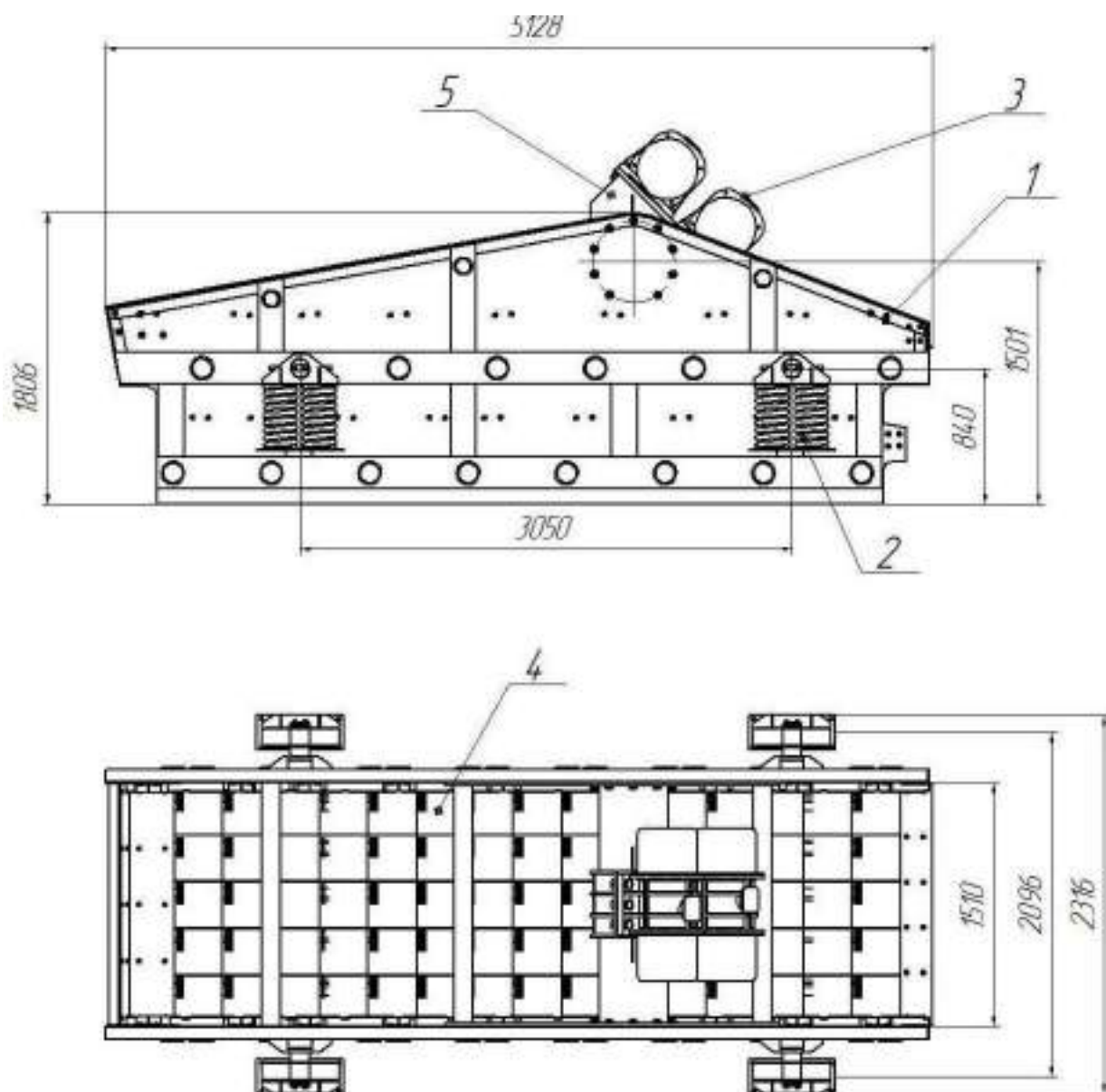
Рисунок 1. Общий вид грохота 1- карод; 2-опора; 3-вибратор 4- Сита; 5- Подвижная балка
