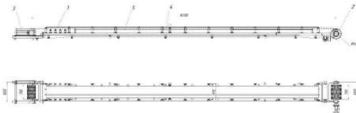
Рис.1 КЛ650.15,73.00.00.00.000 СБ Ленточный конвейер
