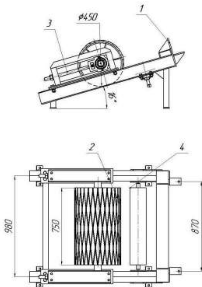
Рис.3 КЛ650.9,68.02.00.00.000 СБ Натяжной барабан
