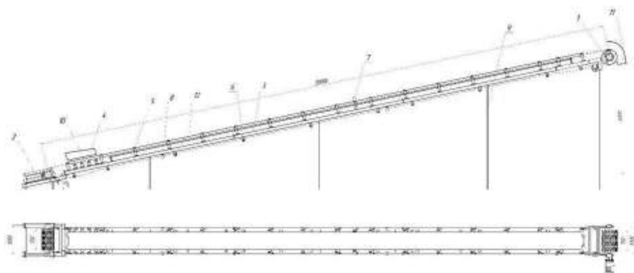
Рис.1 КЛ650.20.00.00.000 СБ Ленточный конвейер
