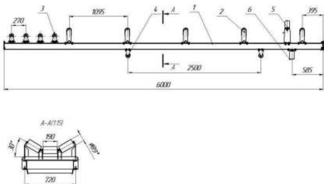
Рис. 5 КЛ500.25.03.00.00.000-01 СБ Линейная секция
