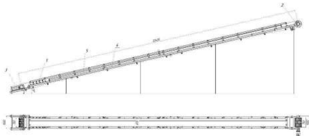
Рис.1 КЛ650.22,42.00.00.00.000 СБ Ленточный конвейер
