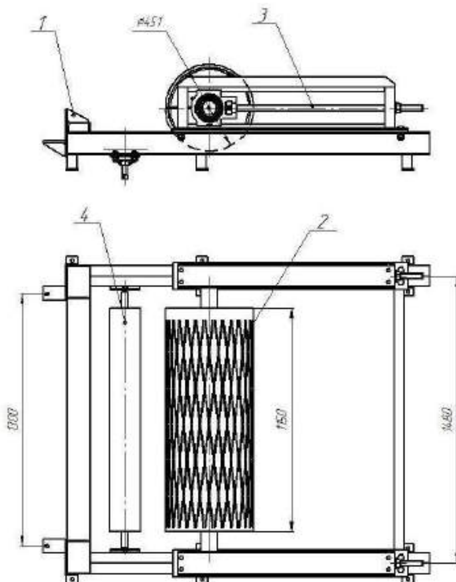
Рис. 3 КЛ1000.41,2.02.00.00.000 СБ Натяжной барабан
