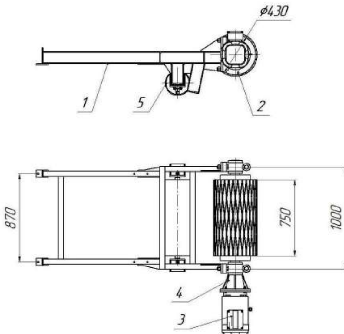
Рис. 2 КЛ650.22,42.01.00.00.000 СБ Приводной барабан
