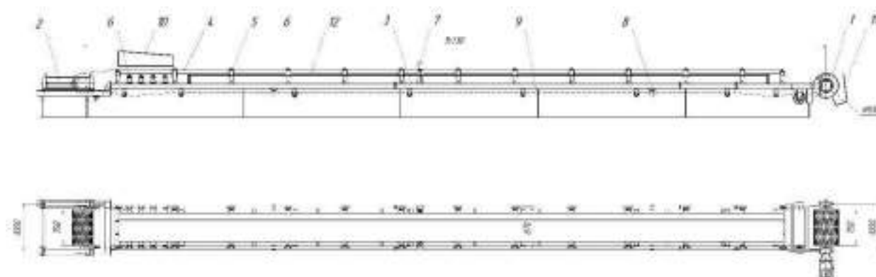
Рис.1 КЛ650.15,73.00.00.000 СБ Ленточный конвейер
