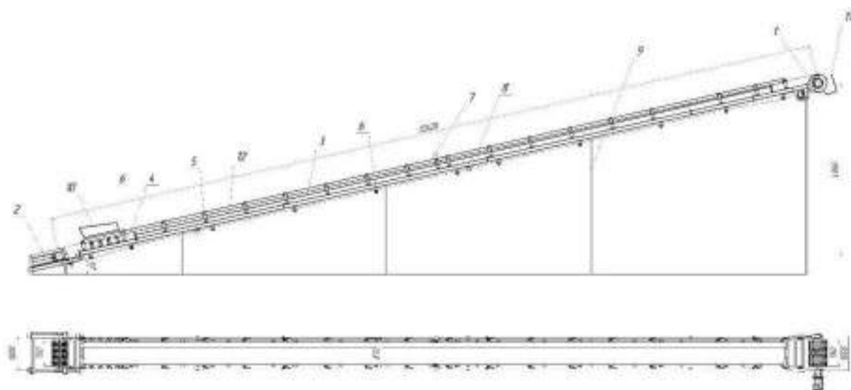
Рис.1 КЛ650.22,42.00.00.000 СБ Ленточный конвейер
