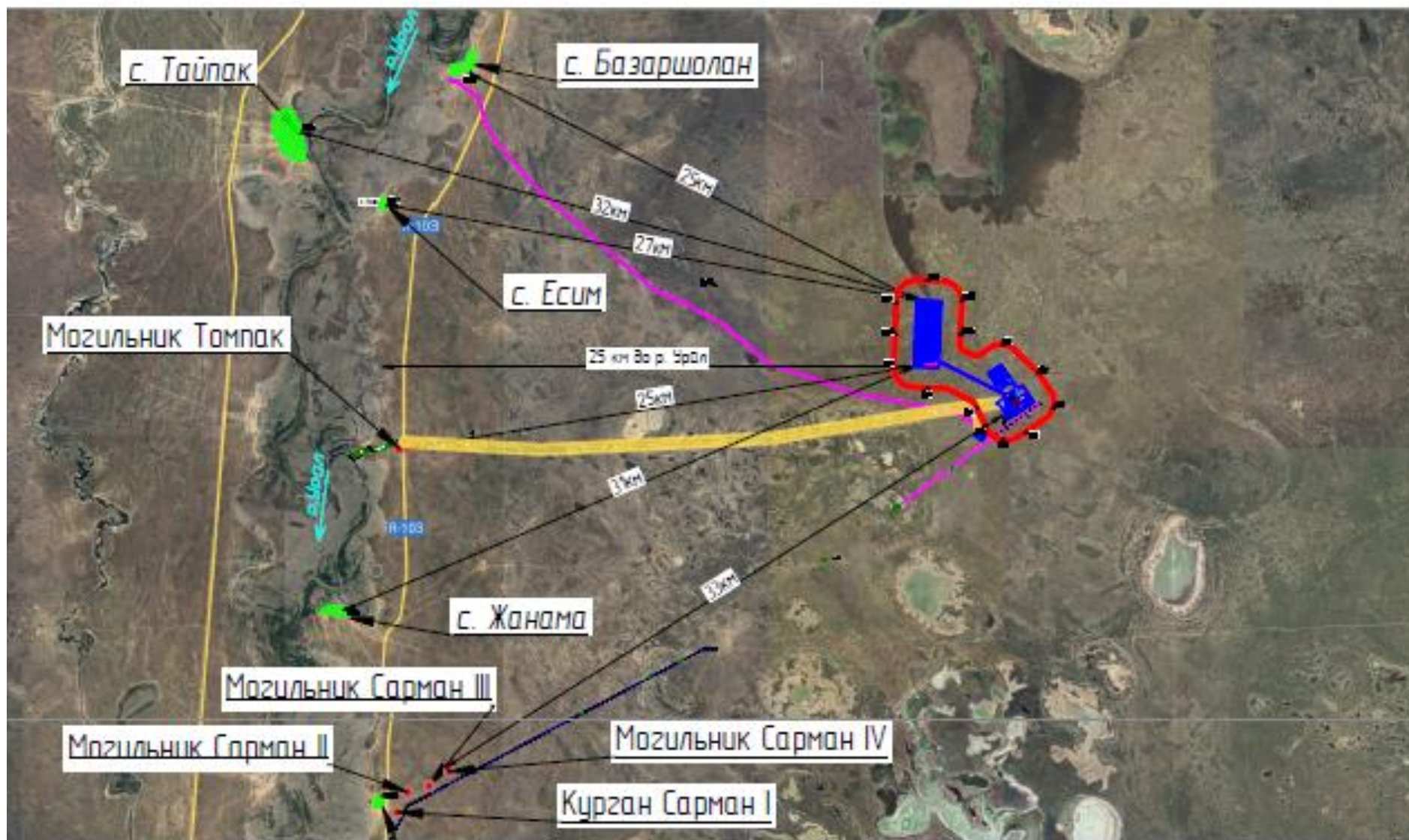
Рисунок 1.2 – Карта-схема района расположения ГОКа месторождения Сатимолы
