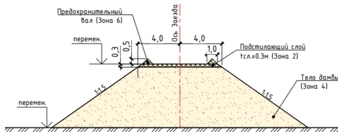
Рисунок 1.9 Типовая конструкция заезда на дамбу.
