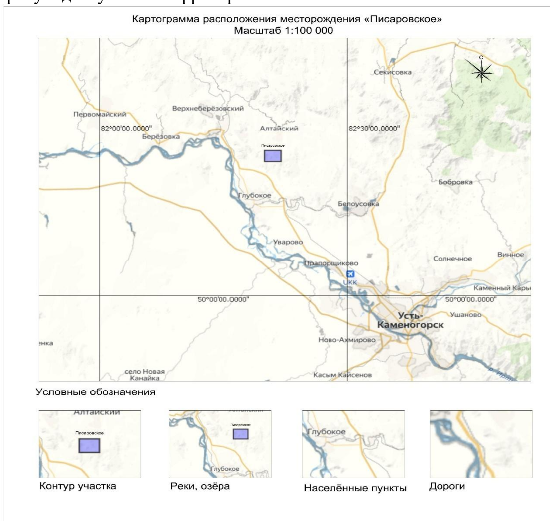
Рисунок 2.1.1. Обзорная карта участка «Писаревский».
