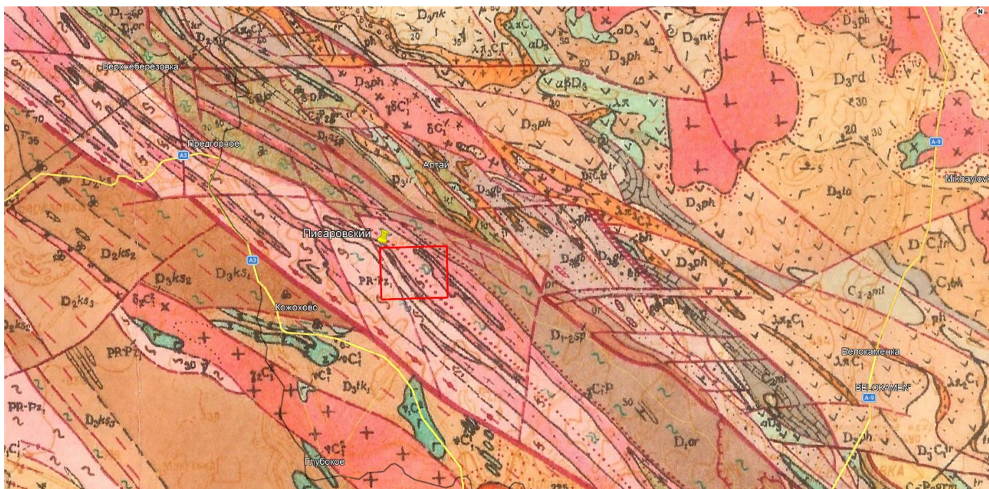
Рисунок 3.1. Геологическая карта м-ба 1:200 000
