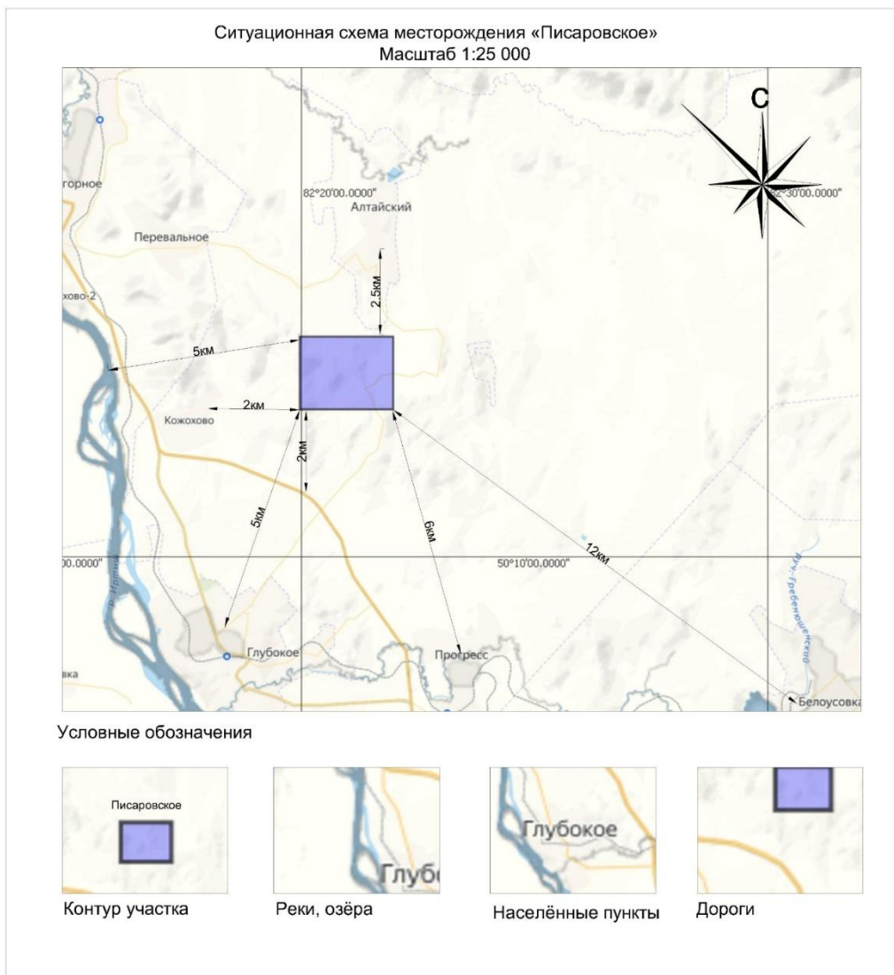
Рисунок 2.1.2. Ситуационная карта-схема расположения участка «Писаревский»
