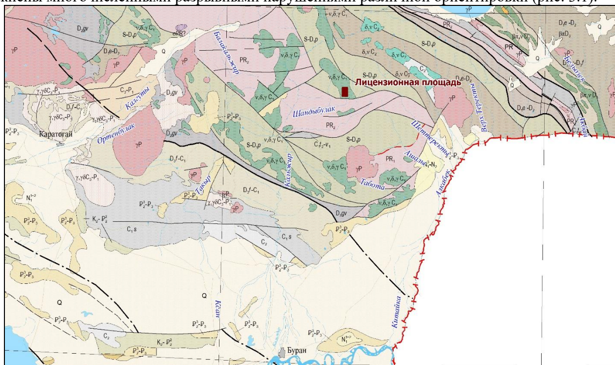
Рис.4 Геологическая карта района
