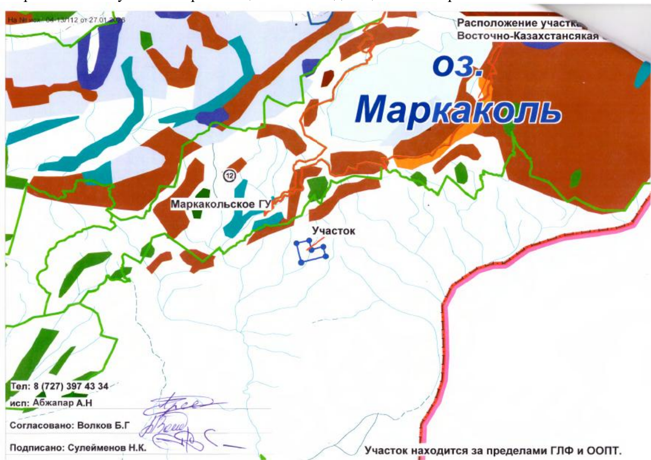
Рисунок 3. Картограмма расположения участка «Южно-Алтайская площадь»
