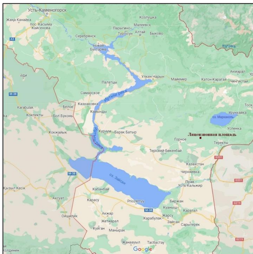
Рисунок 1. Обзорная карта участка «Южно-Алтайская площадь»
