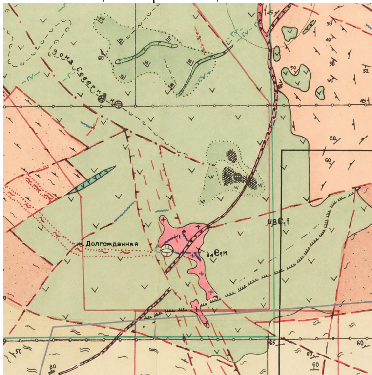
Рис. 5 Геологическая карта участка
