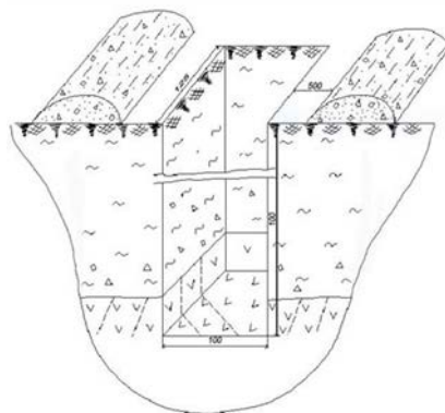
Рис. 1.8 Паспорт проходки шурфов глубиной до 3,0 м.
