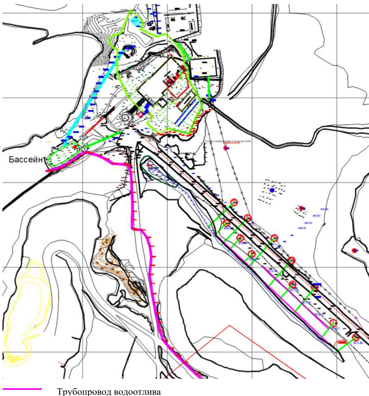
Рисунок 6.2 – Схема водоотлива карьерных вод месторождения Коктасжал (продолжение)
