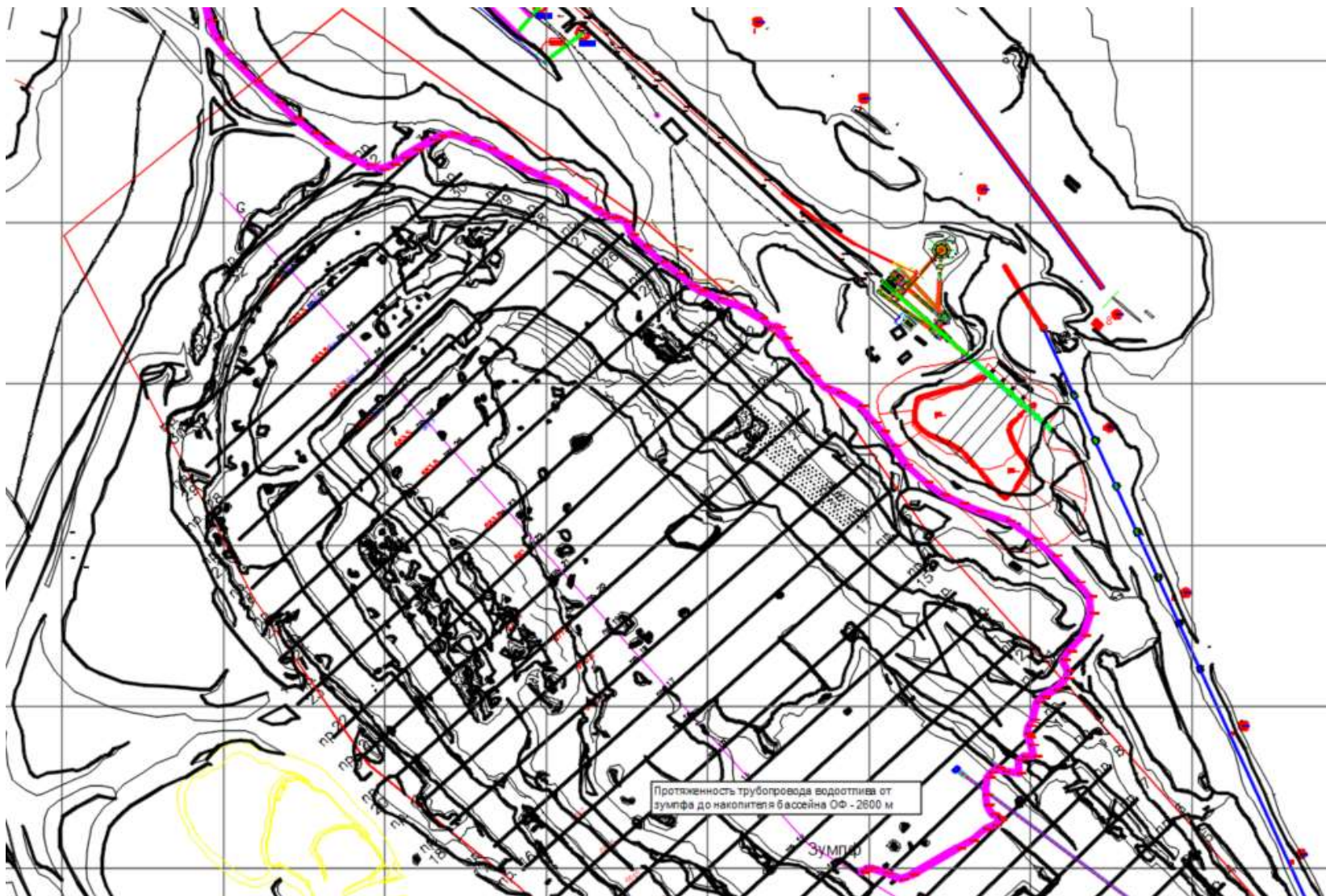
Рисунок 6.1 – Схема водоотлива карьерных вод месторождения Коктасжал
