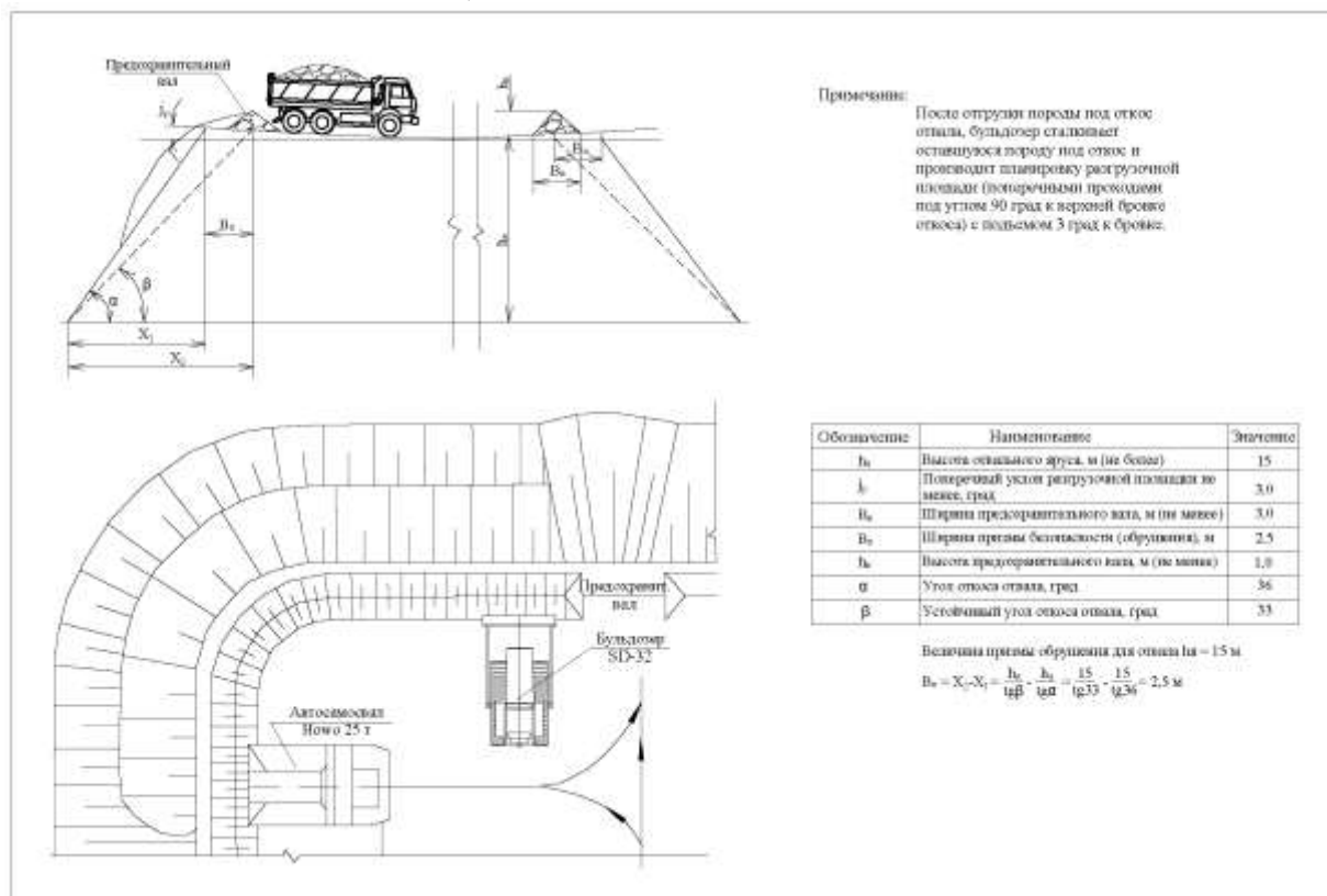
Рисунок 1.5.10.1 Технологическая схема отвалообразования
