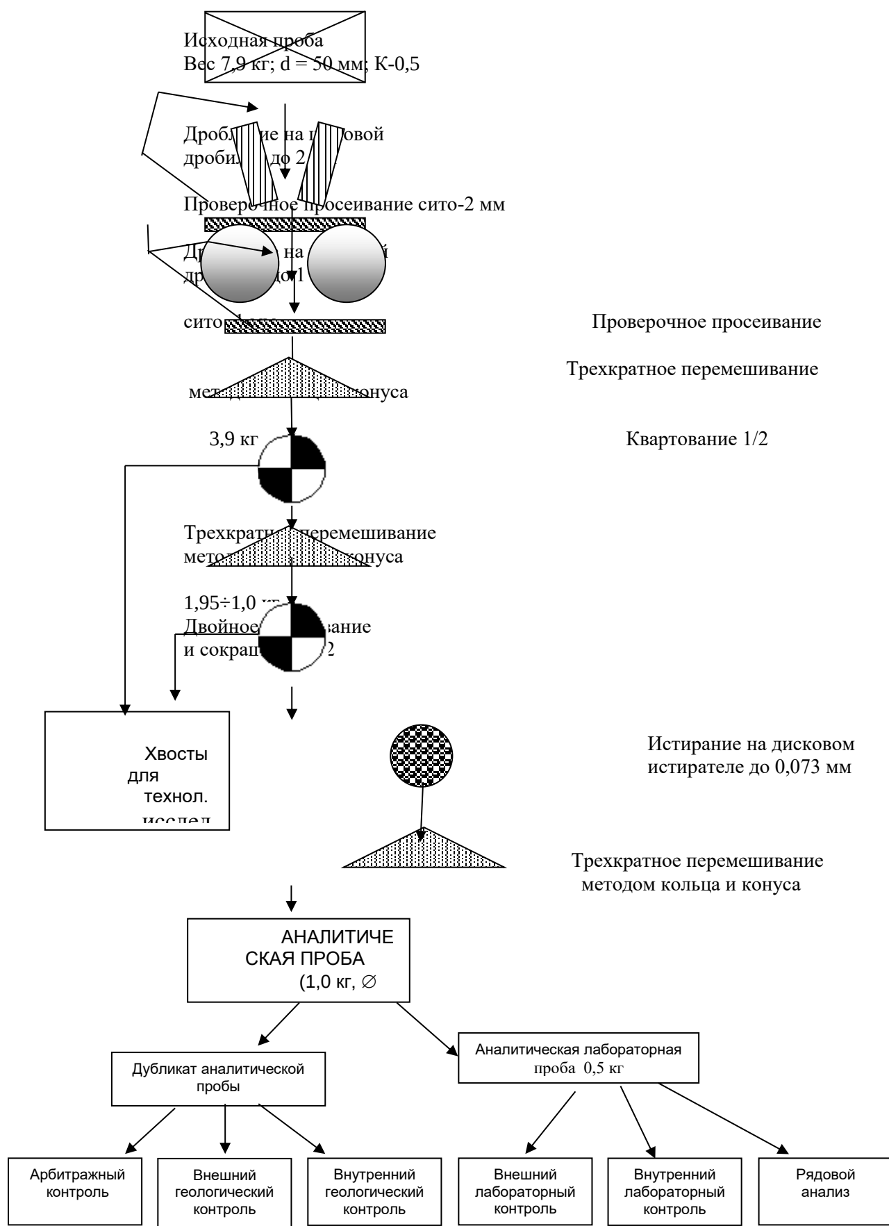
Рисунок 1.5.14.1 - Схема обработки бороздовых проб Аналитические работы
