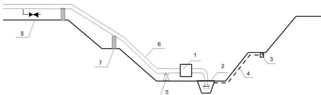
Рисунок 1.8.2.2.1- Схема карьерного водоотлива
