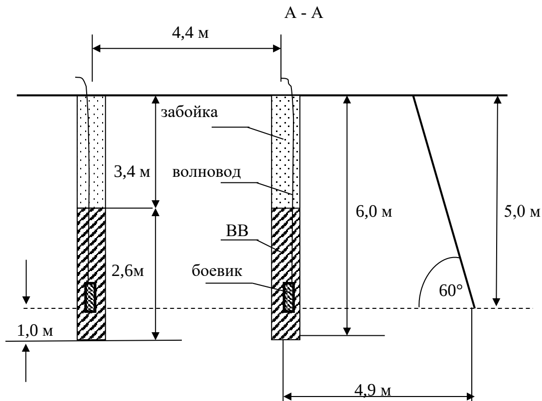
Рисунок 1.5.4 1-Конструкция заряда
