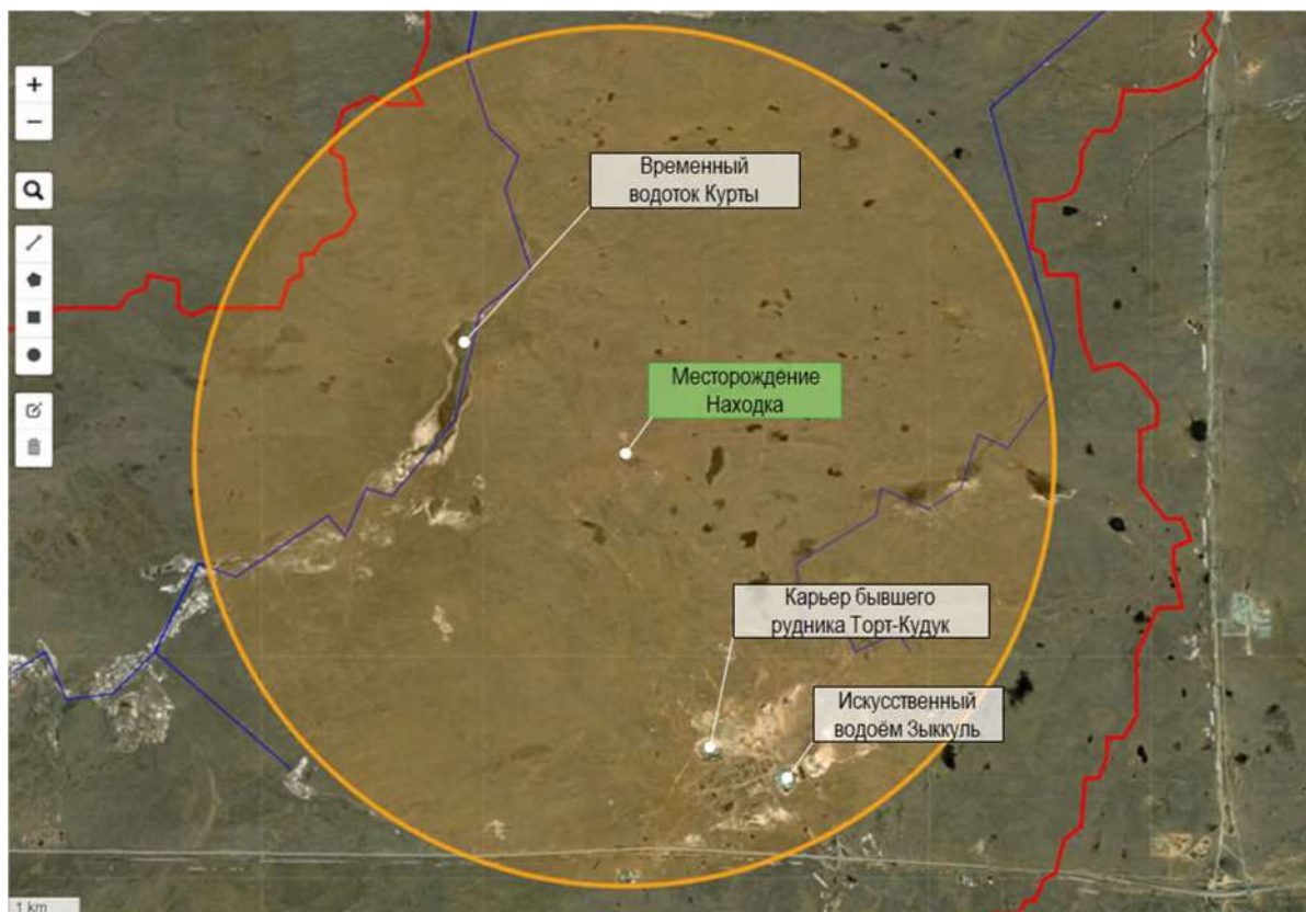
Рисунок 3-13 Поверхностные водные объекты в районе месторождения
