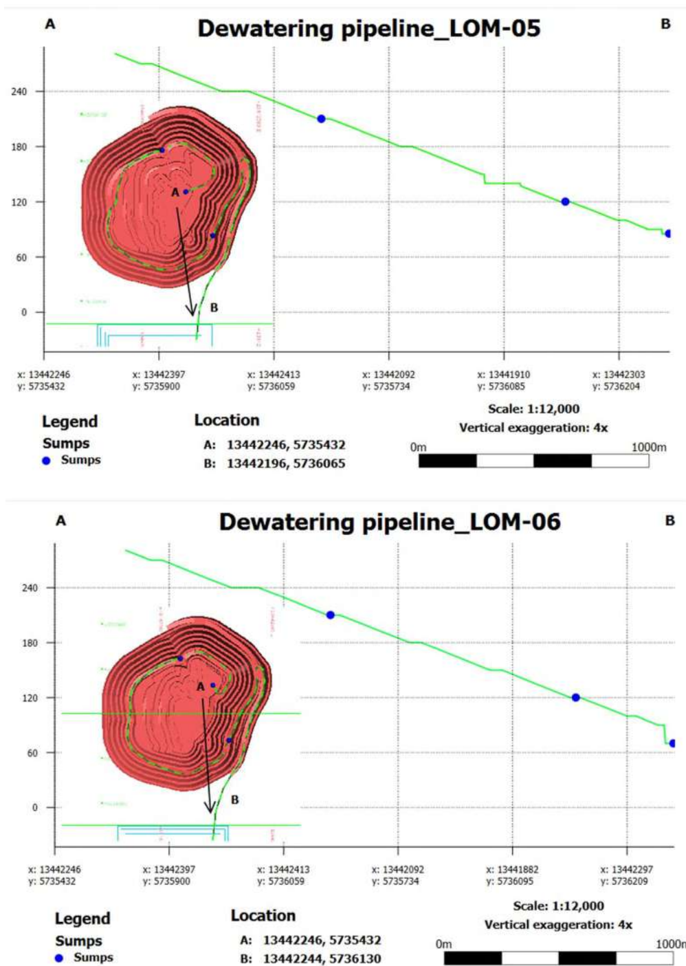
Рисунок 5-14 Разрез линии трубопроводов на дизайн 5 и 6 года
