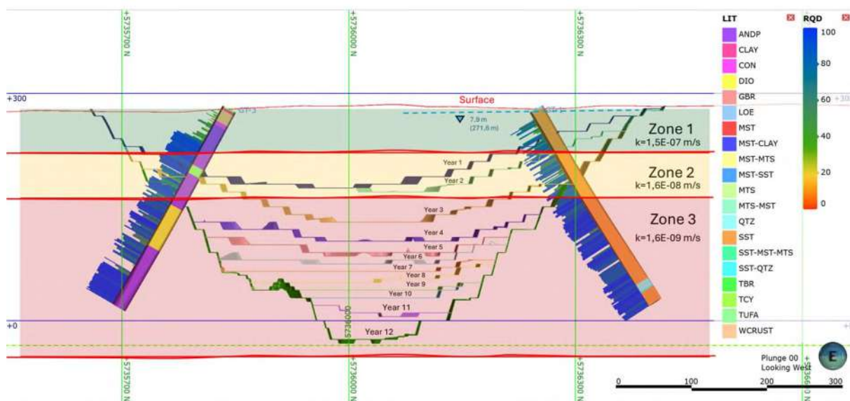
Рисунок 5-9 – Гидрогеологическая концептуальная модель, используемая для расчета притока
