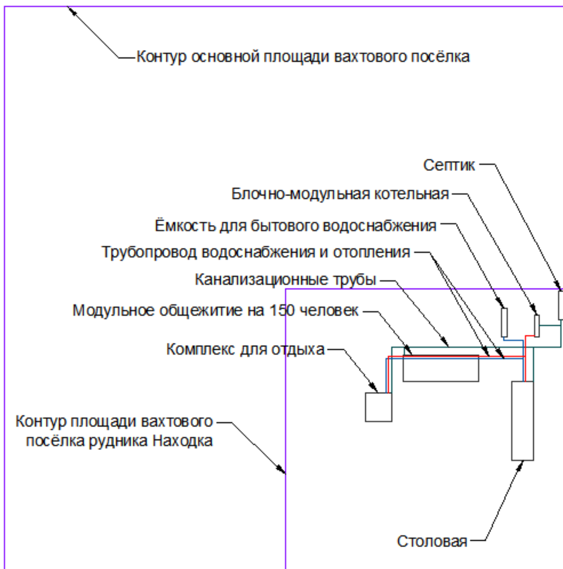
Рисунок 5.4 Схема вахтового посёлка
