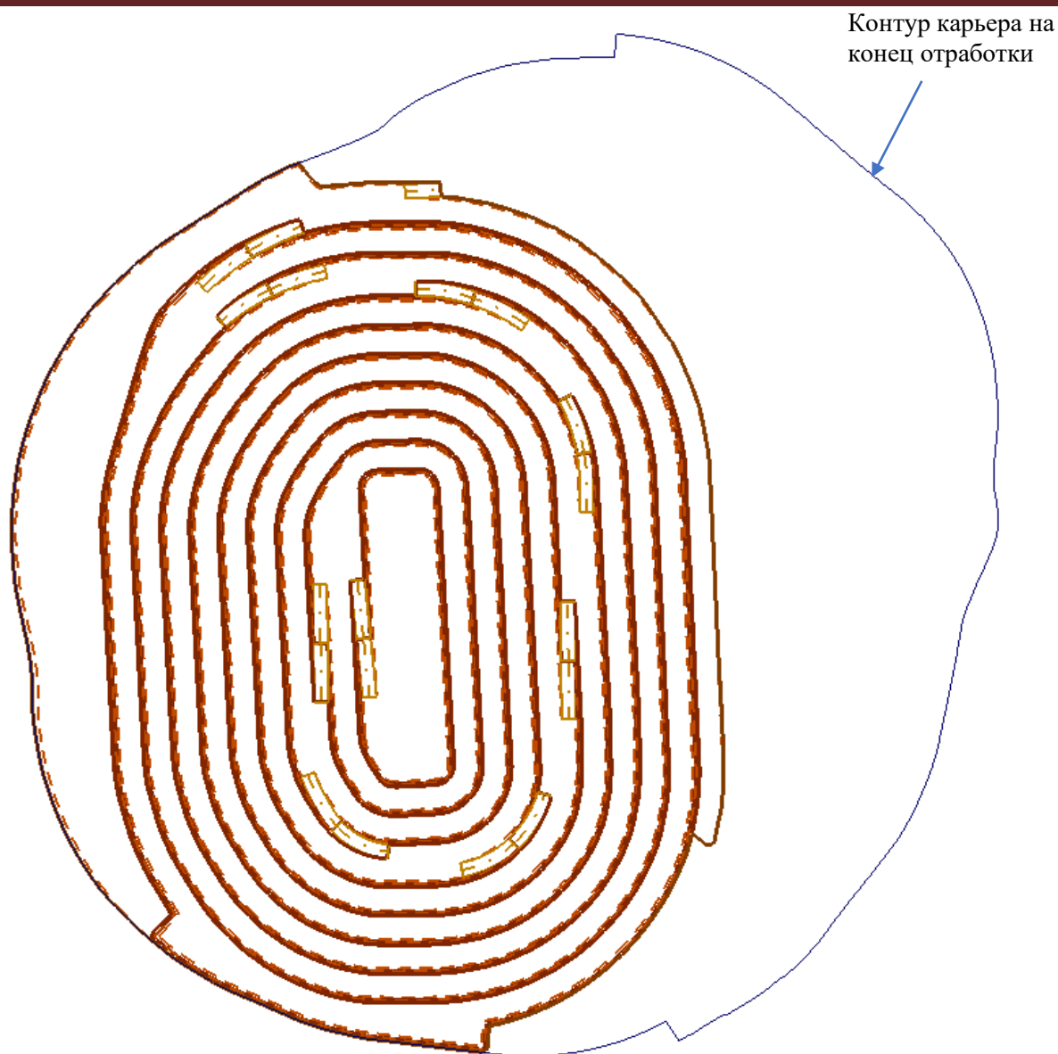
Рисунок 5.1. План карьера на момент вскрытия.
