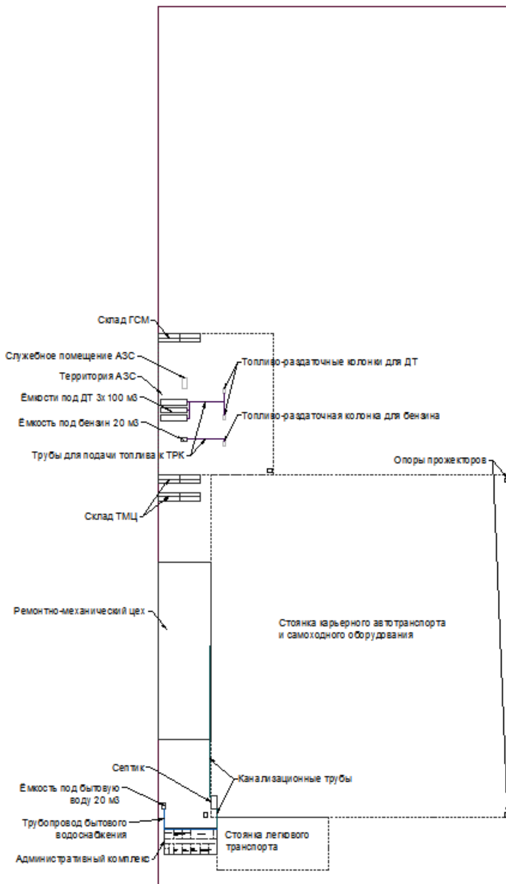
Рисунок 5.5 Схема промышленной площадки
