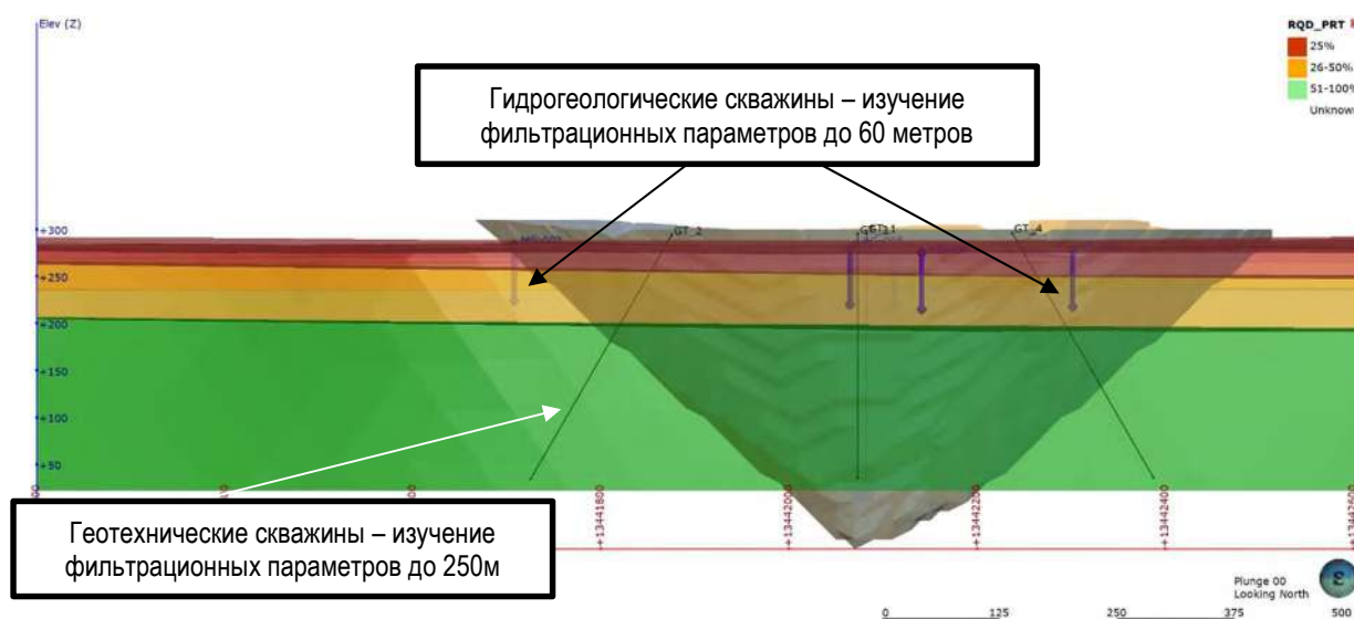
Рисунок 4-1 Схема изучения параметров с глубиной
