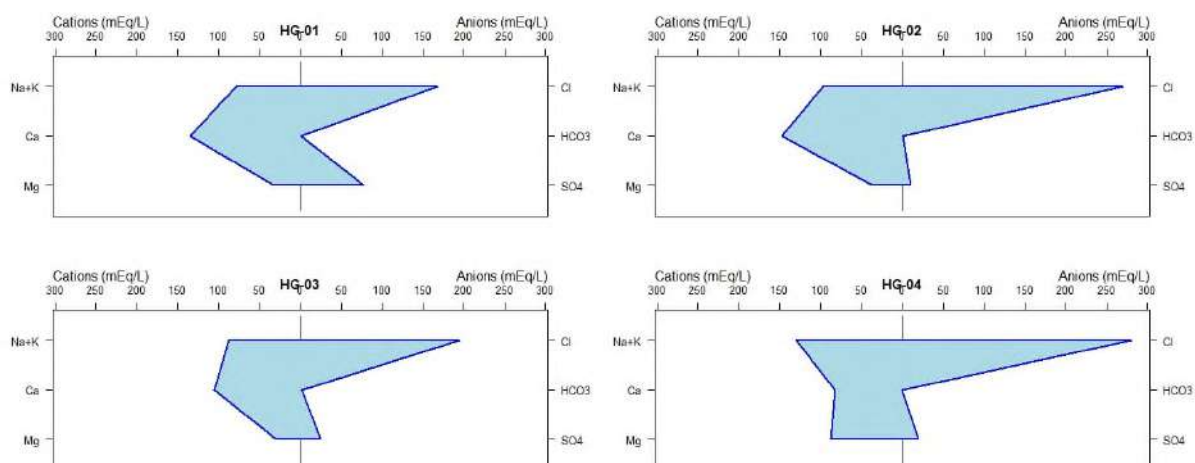
Рисунок 4-8 Диаграммы Stiff для образцов подземных вод (HG 01–HG 04), с катионами слева и анионами справа в ме/л. Полигоны демонстрируют выраженную асимметрию в сторону \text{Cl}^- и значительный вклад \text{Na}^+ и \text{Ca}^{2+} . HG 01 и HG 02 характеризуются фациями Ca–Cl, HG 03 показывает смешанный профиль Ca–Na–Cl, а HG 04 смещается к фации Na–Cl, что отражает прогрессивное геохимическое созревание воды
