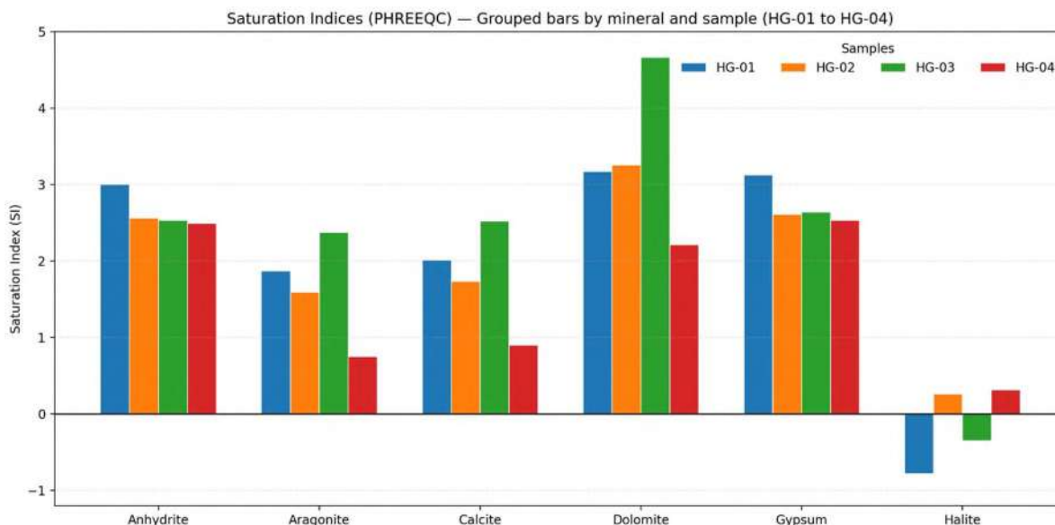
Рисунок 4-9 Индексы насыщения (PHREEQC) — сгруппированные столбцы по минералам и образцам (HG-01–HG-04)
