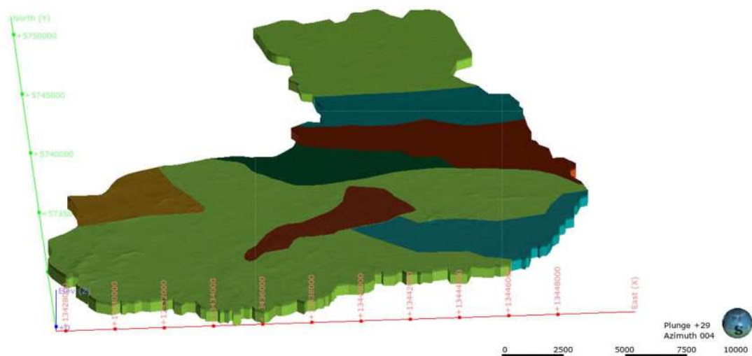
Рисунок 5-6 – Окончательная геолого-гидрогеологическая концептуальная модель
