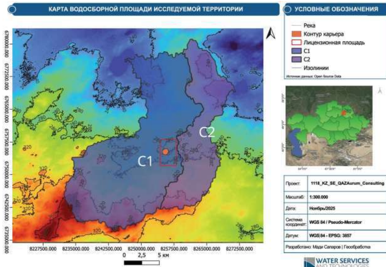
Рис. 2.4 - Водосборные площади в районе месторождения Находка
