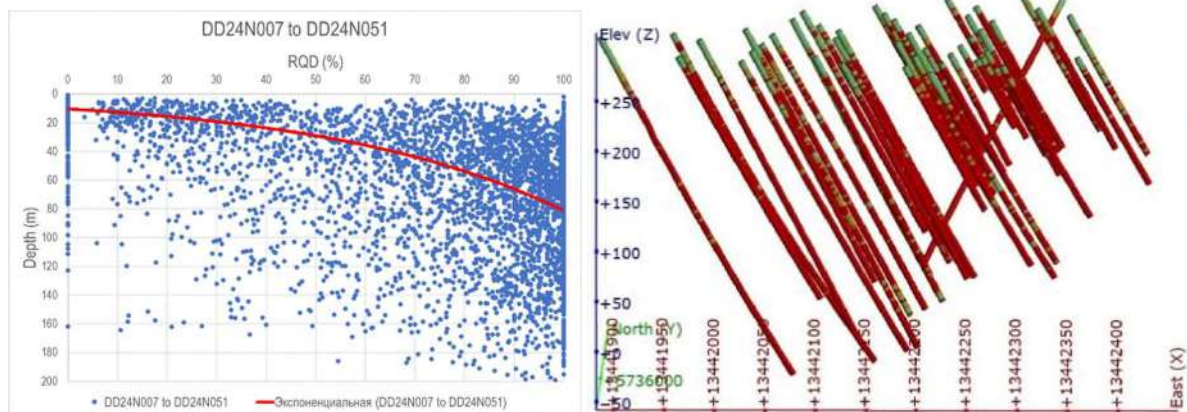
Рисунок 3-16313 Индекс качества породы с глубиной
