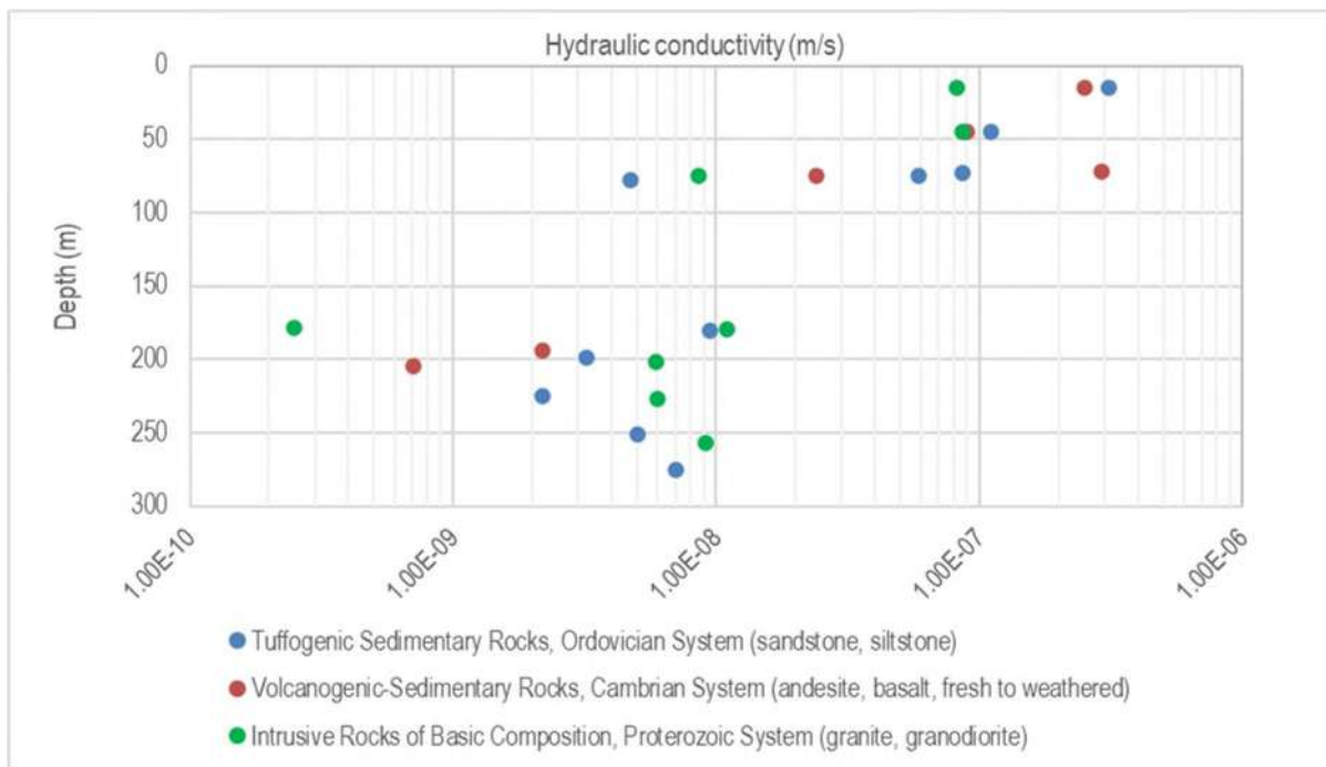
Рисунок 5-1 Зависимость коэффициента фильтрации от глубины для каждой гидрогеологической единицы
