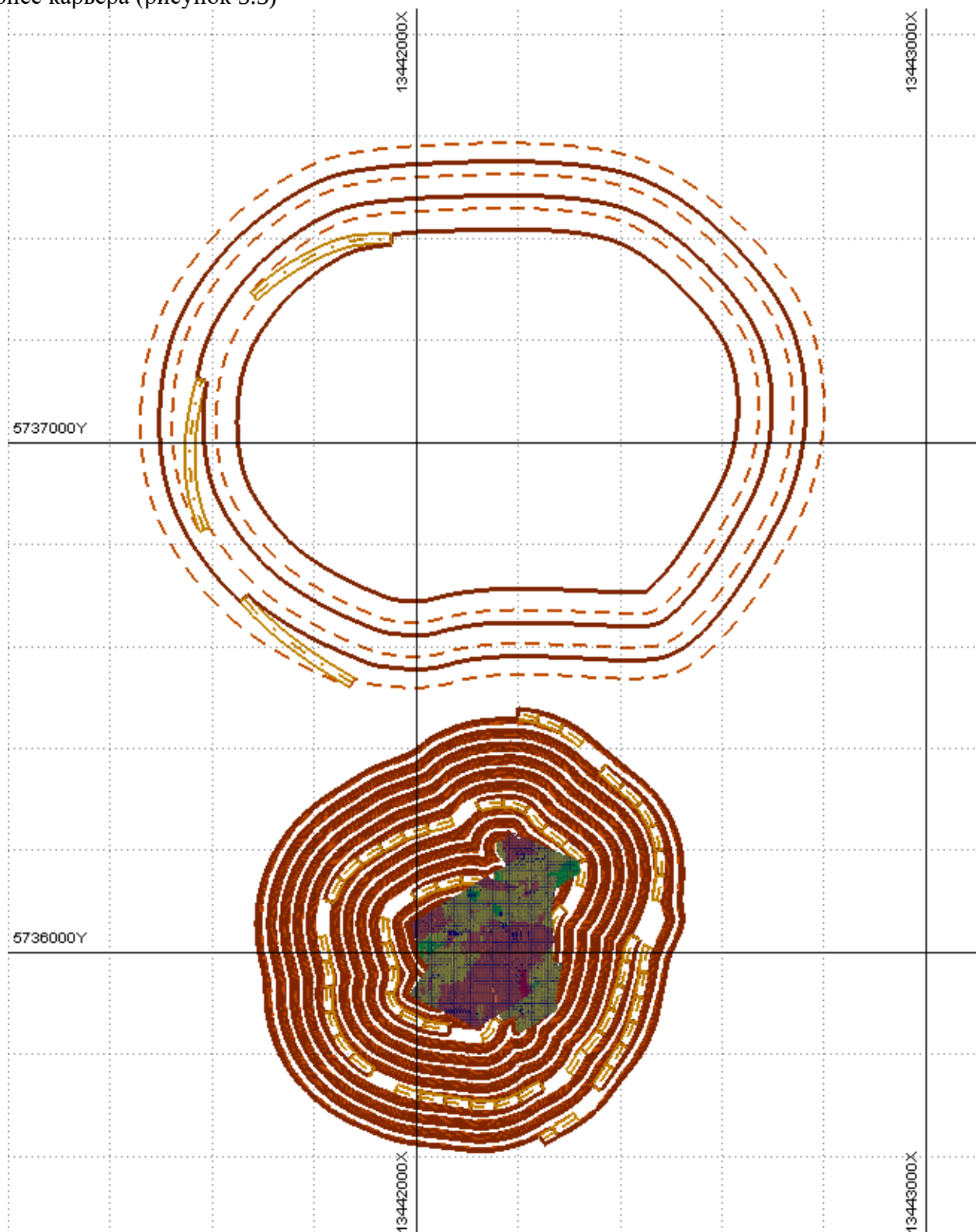
Рисунок 5.3 Схема расположения отвала
