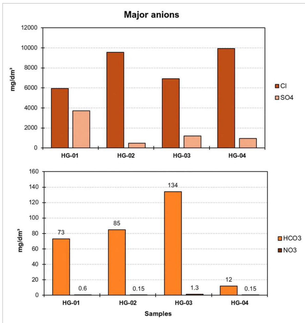
Рисунок 4-6 Распределение основных анионов между четырьмя образцами, отобранными в рамках данного исследования
