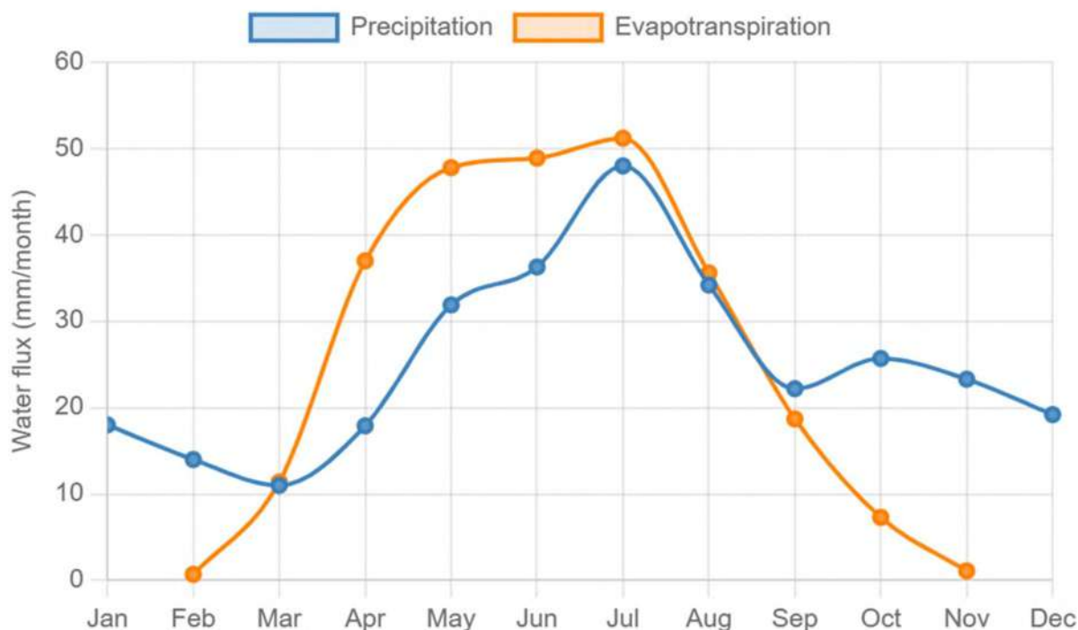
Рисунок 3-10 Климатология водосборного бассейна: среднеемесячное количество осадков и эвапотранспирации на водосборном бассейне
