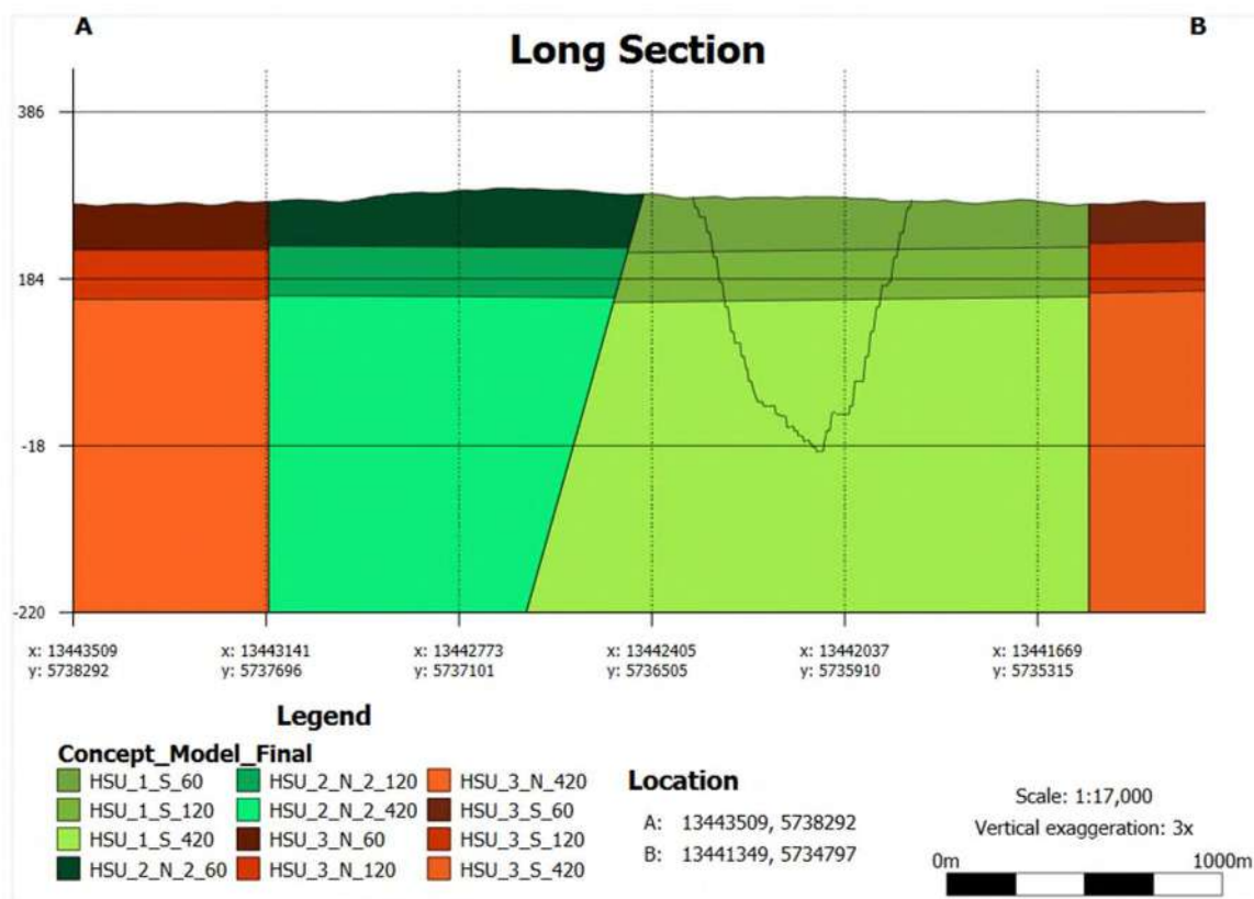
Рисунок 5-7 – Разрез 3D геолого-гидрогеологической модели с указанием финального дизайна карьера
