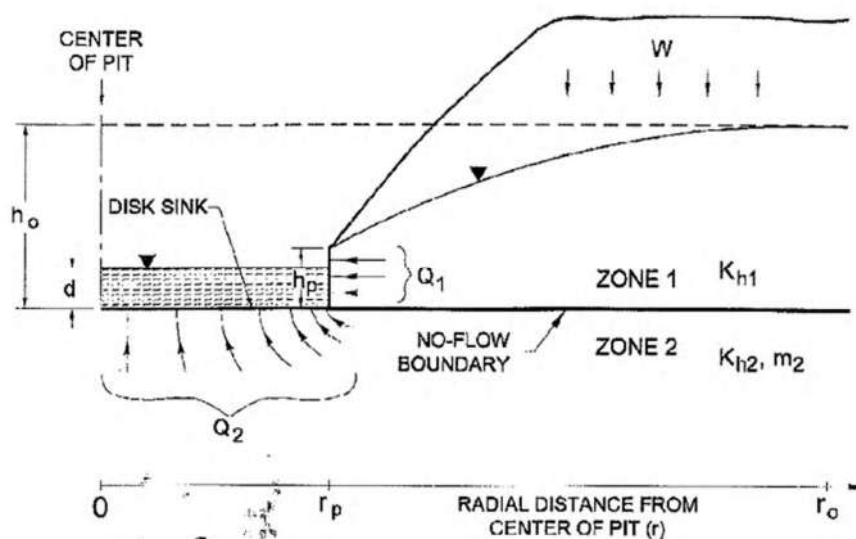
Рисунок 5-8 – Концептуальная модель движения подземных вод для открытого карьера (Marinelli и Nicoli, 2000)
