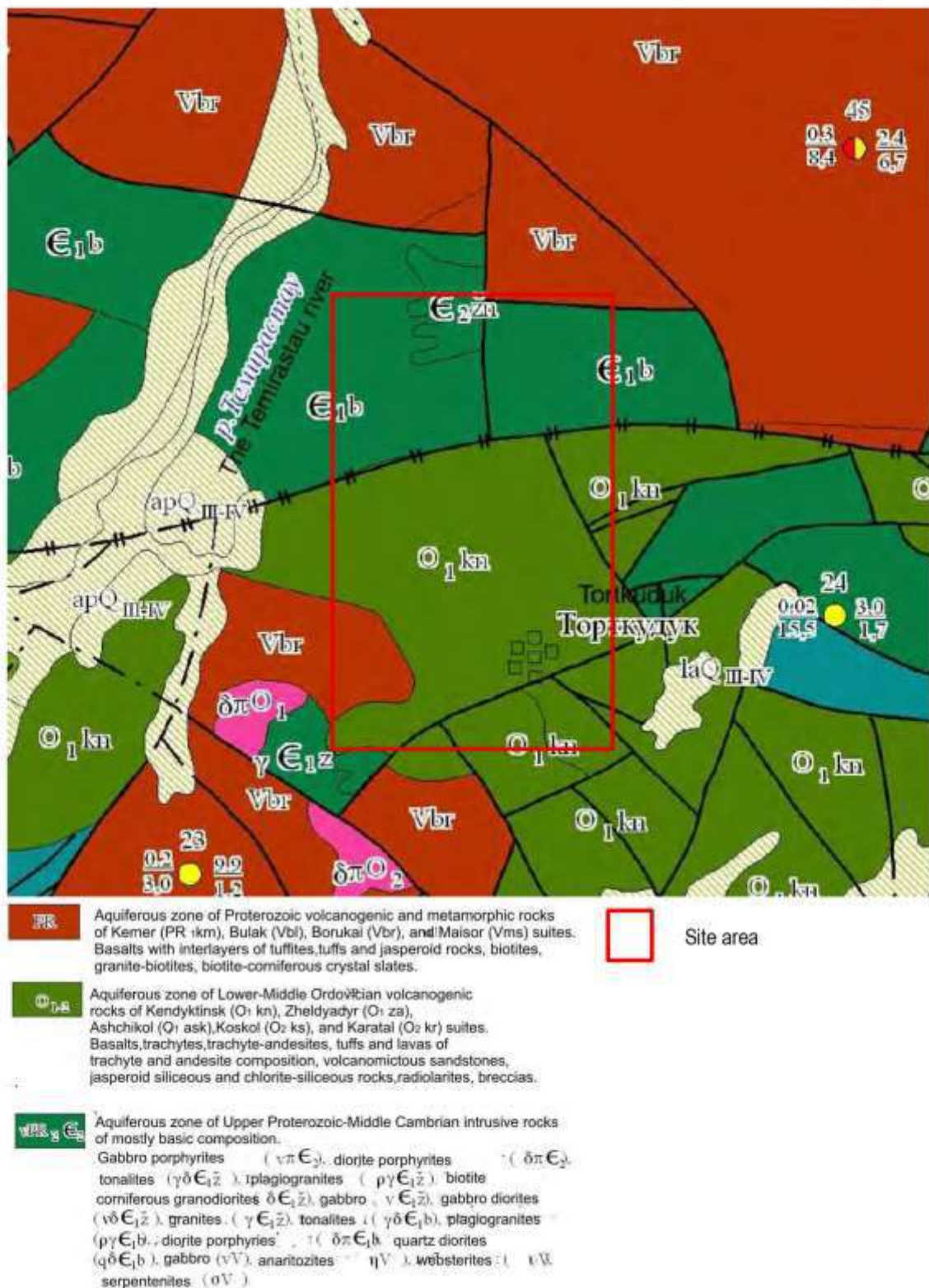
Рис. 2.7 - Геологическая карта участка работ
