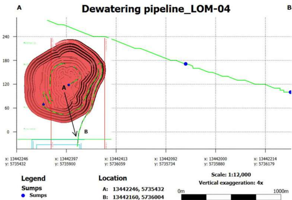
Рисунок 5-13 Разрез линии трубопроводов на дизайн 3 и 4 года
