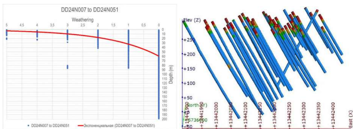
Рисунок 3-15 Интенсивность выветрелости с глубиной
