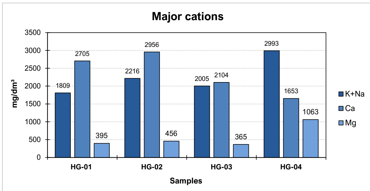
Рисунок 4-5 Распределение основных катионов между четырьмя образцами, отобранными в рамках данного исследования
