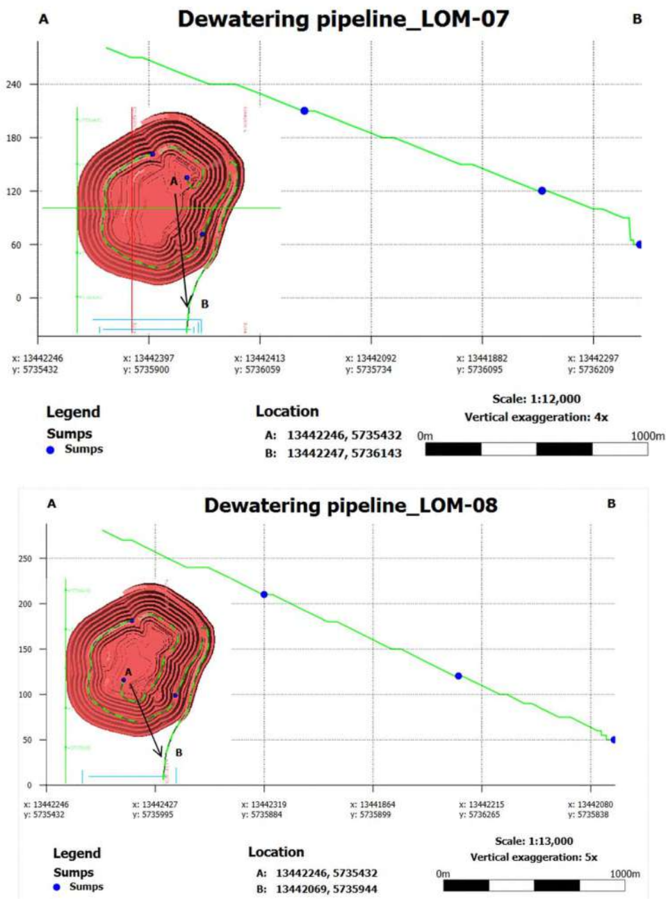
Рисунок 5-15 Разрез линии трубопроводов на дизайн 7 и 8 года
