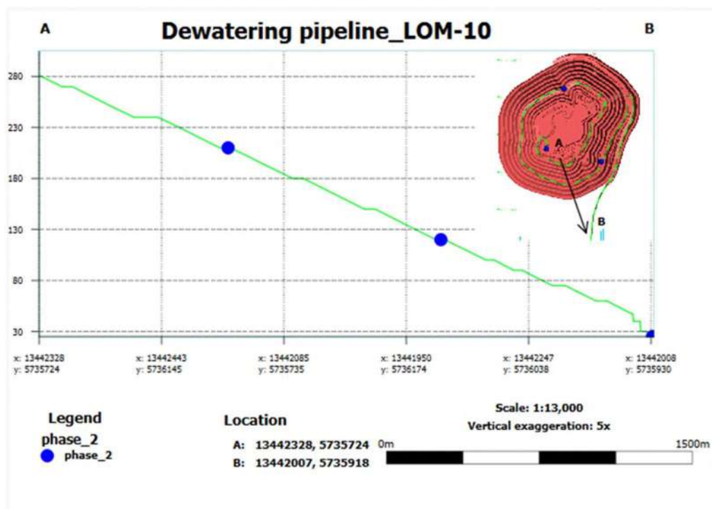
Рисунок 5-16 Разрез линии трубопроводов на дизайн 9 и 10 года
