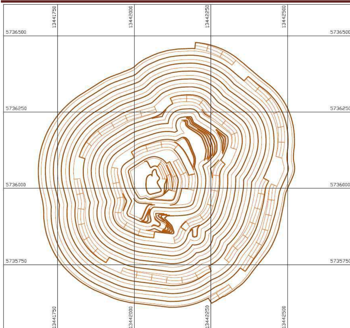
Рисунок 5.2- Контур карьера на конец отработки
