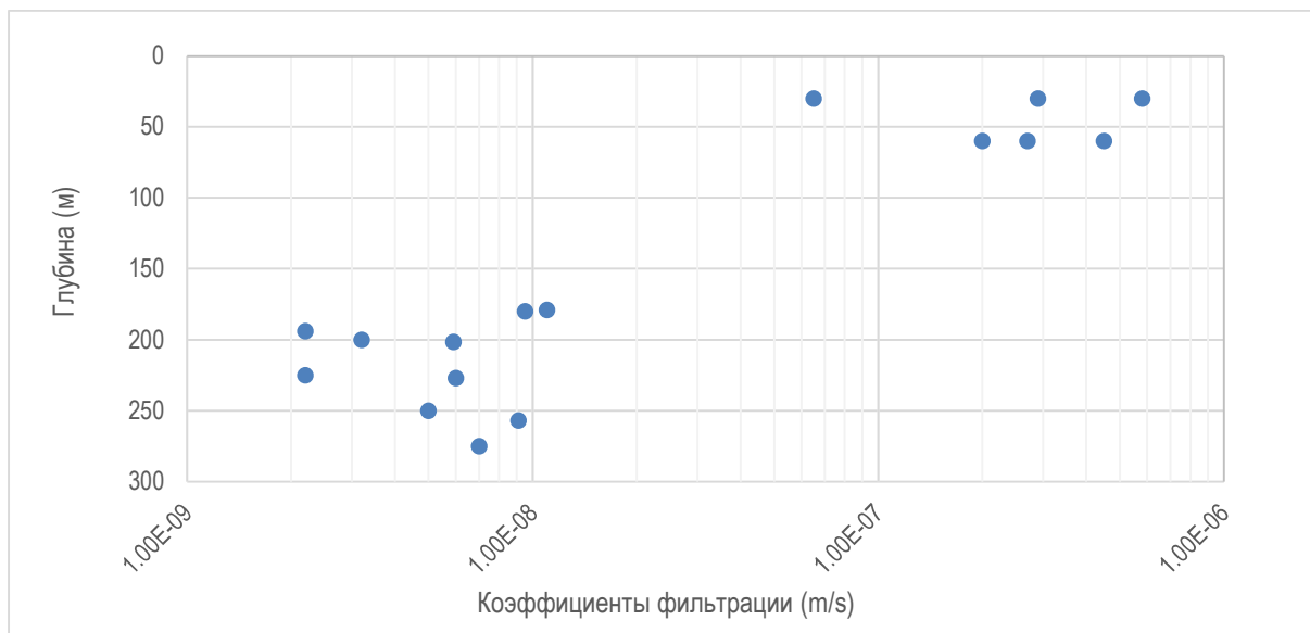
Рисунок 4-3 Зависимость коэффициента фильтрации от глубины для программы испытаний 2025 года
