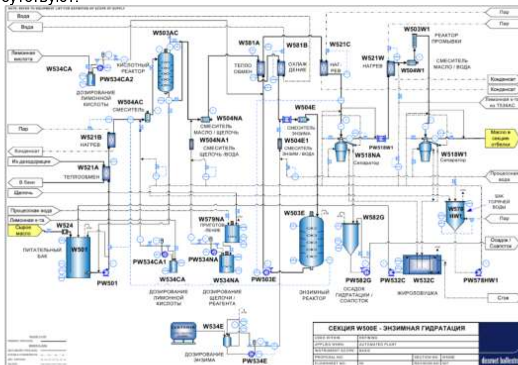
Рисунок 1.8.1 – Технологическая схема отделения гидратации (дегумирования) и нейтрализации
