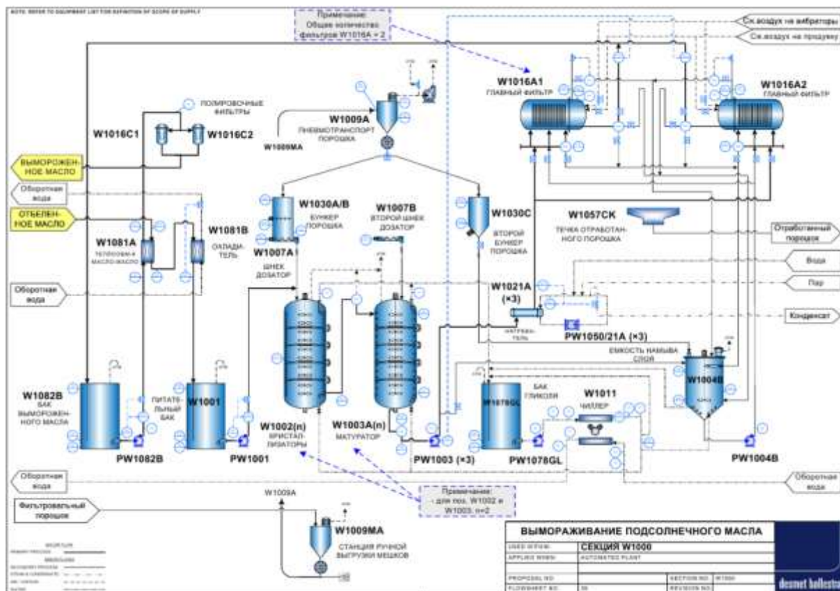
Рисунок 1.8.3 – Технологическая схема отделения винтеризации (вымораживания)
