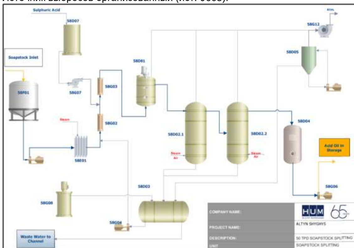
Рисунок 1.8.5 – Технологическая схема отделения разложения соапстока
