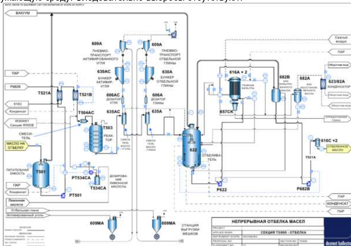
Рисунок 1.8.2 – Технологическая схема отделения отбеливания
