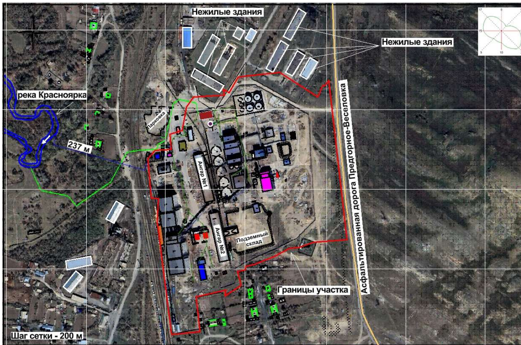
Рисунок 1 – Ситуационная карта-схема рассматриваемого объекта
