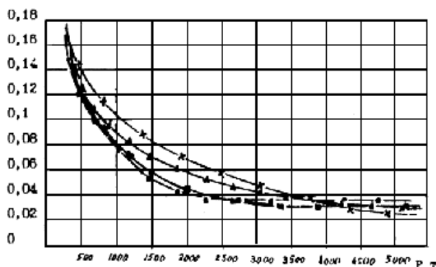
Рисунок 17.3 – Изменение значений удельных выбросов CO грузовыми тепловозами в зависимости от весов перевозимых поездов
