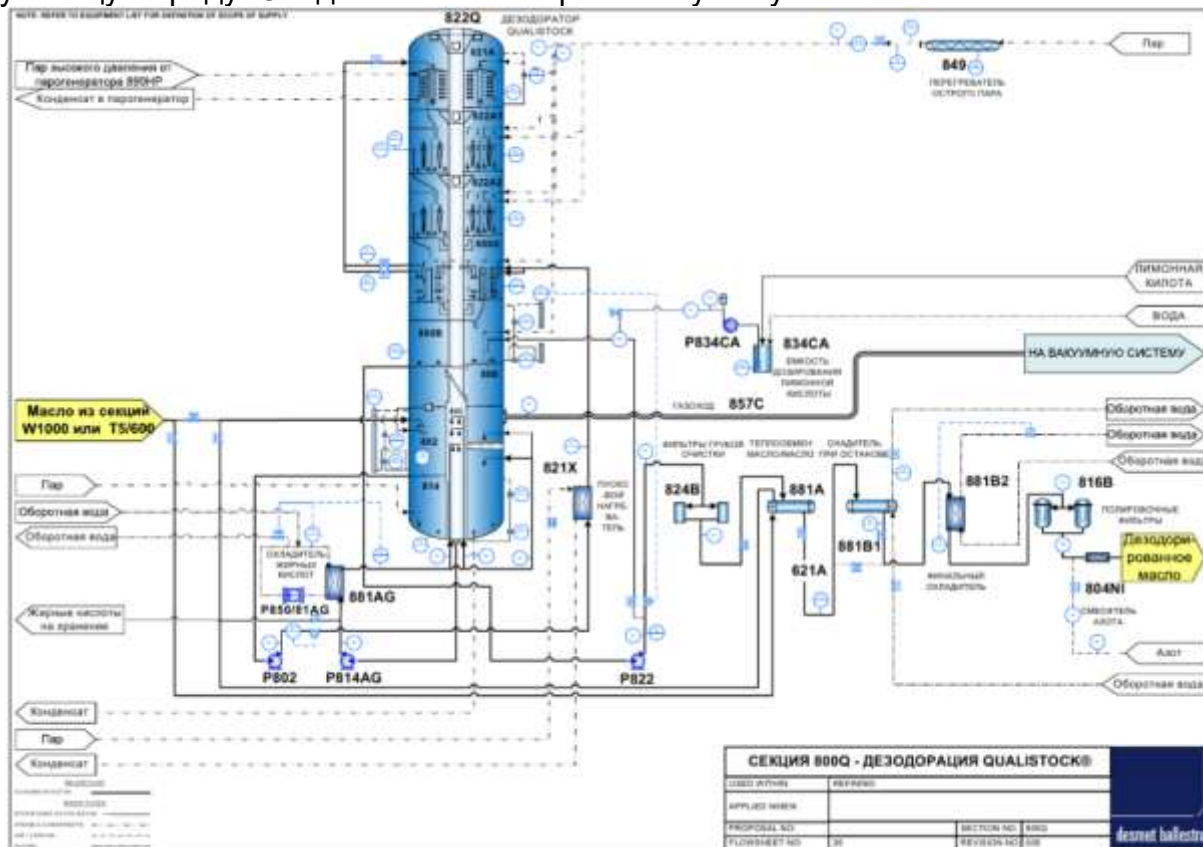
Рисунок 1.8.4 – Технологическая схема отделения дезодорации
