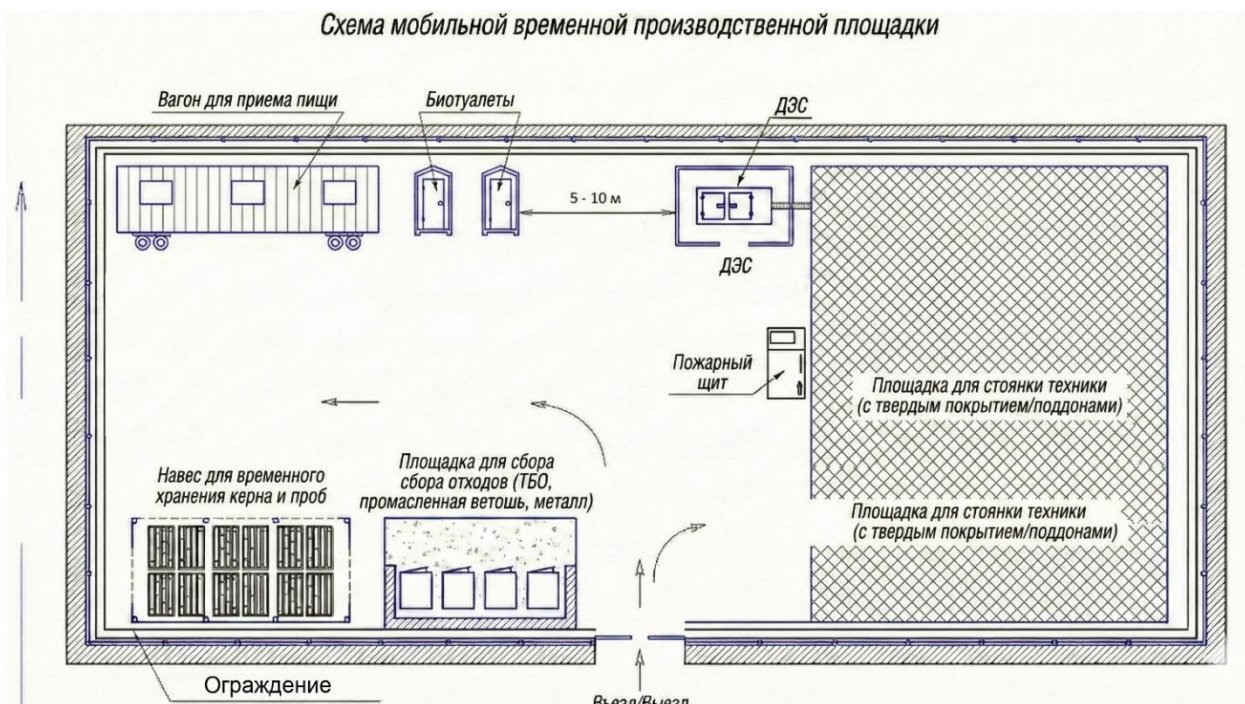
Рисунок 5.3. Схема мобильной временной производственной площадки.
