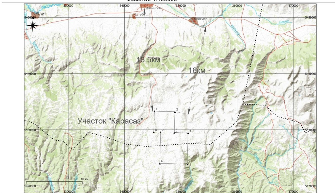
Ситуационная карта-схема расположения участка "Карасаз" масштаб 1:150000
