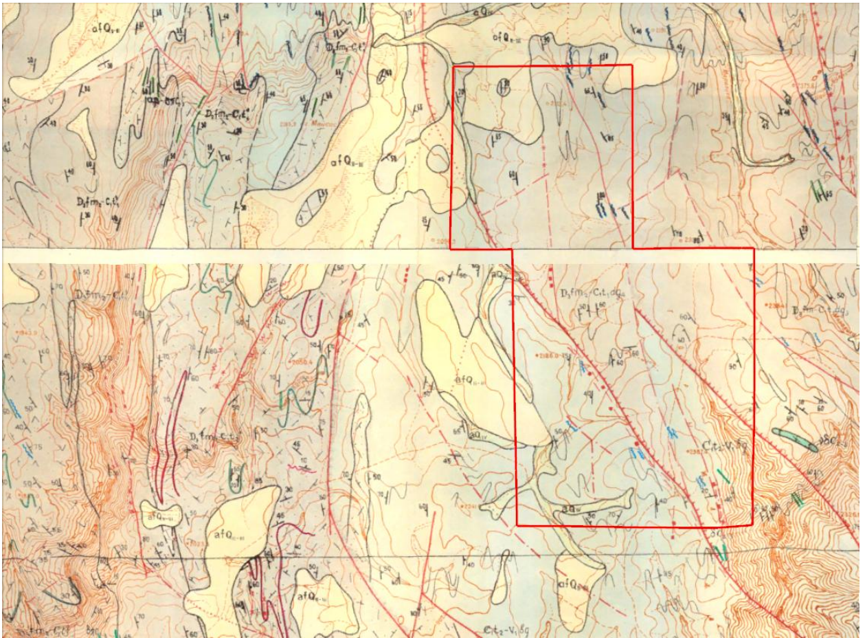
Рис. 3.1 Геологическая карта участка «Карасаз»
