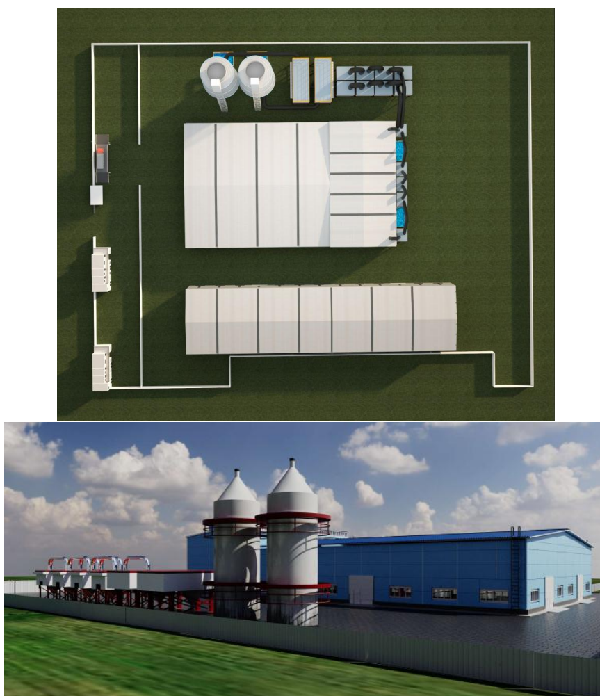
Рисунок 5.1 – Генеральный план расположения объектов
