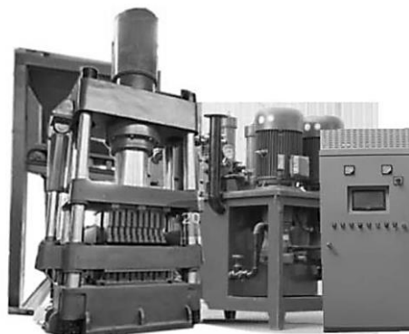
Сурет 1. Кірпіш жасауға арналған баспақ.
