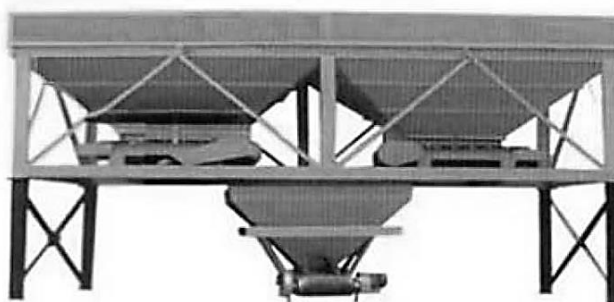
Сурет 3. Мөлшерлегіш.
