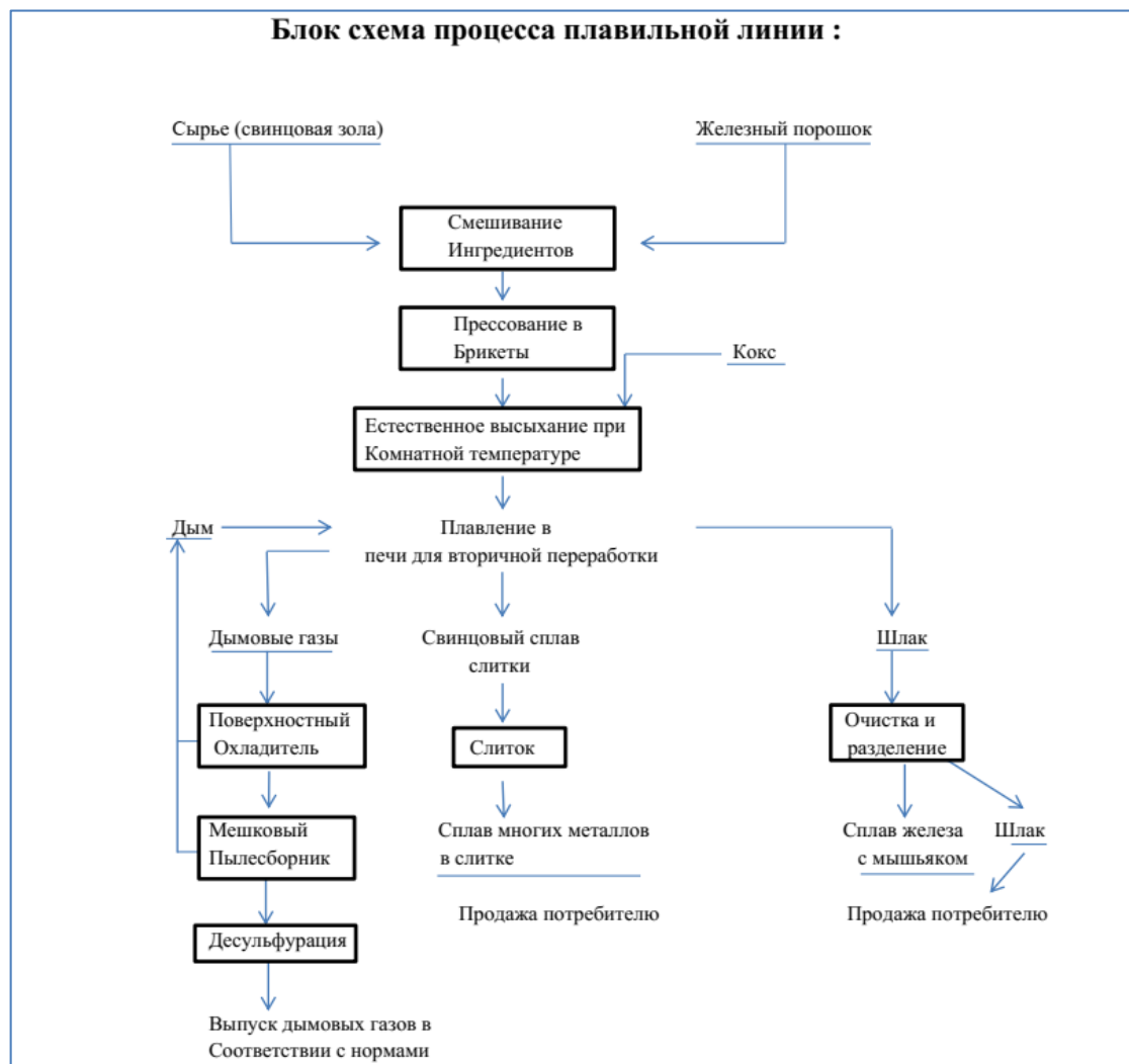
Рисунок 5.3 – Блок-схема технологического оборудования и технологии
