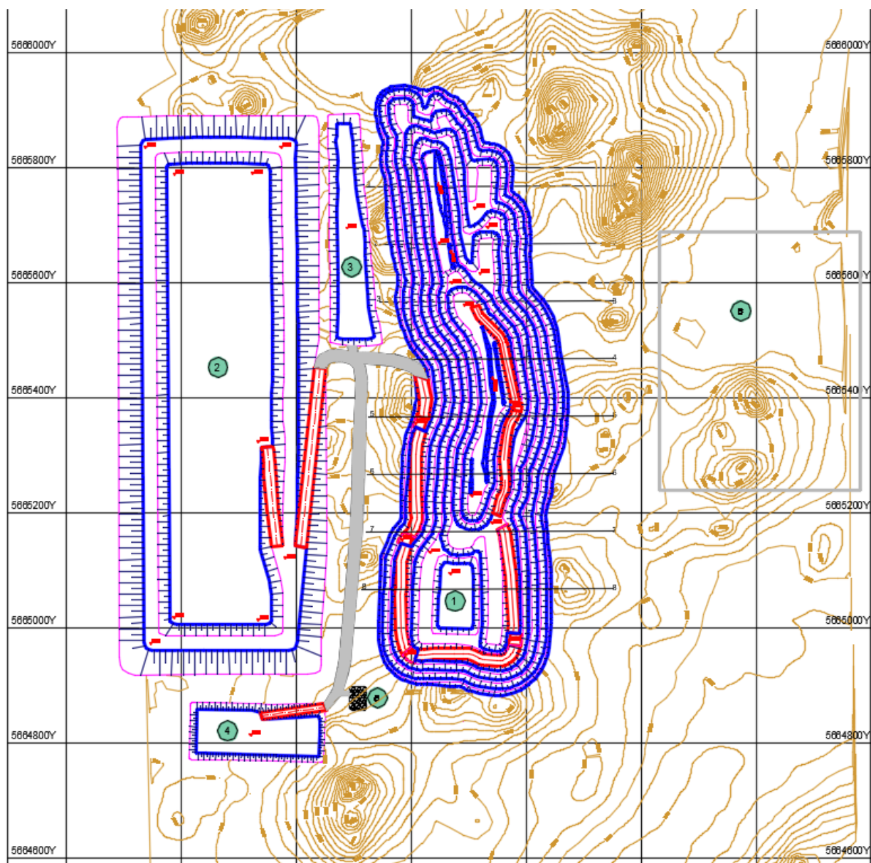
Рис. 1.4 – Генеральный план месторождения
