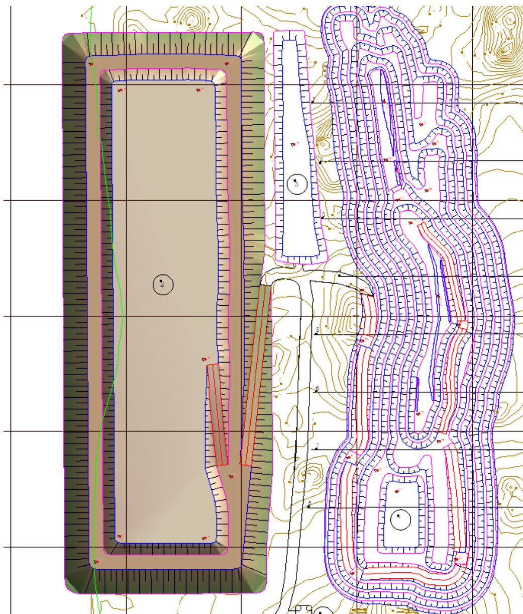
Рис. 1.8 – Проектный контур Отвала вскрышных пород
