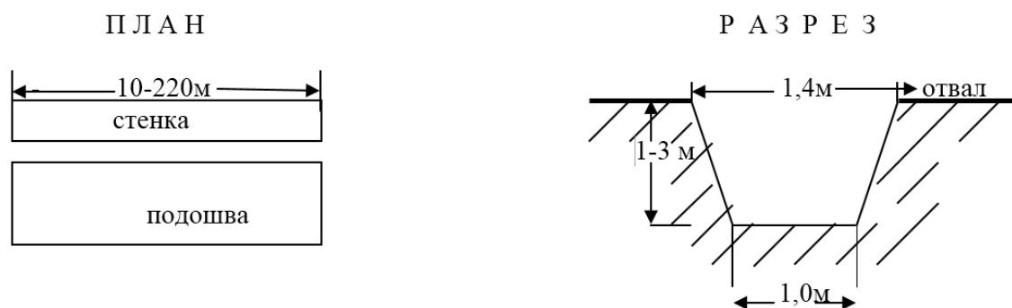
Рисунок. 5.10.2. Паспорт проходки канав
