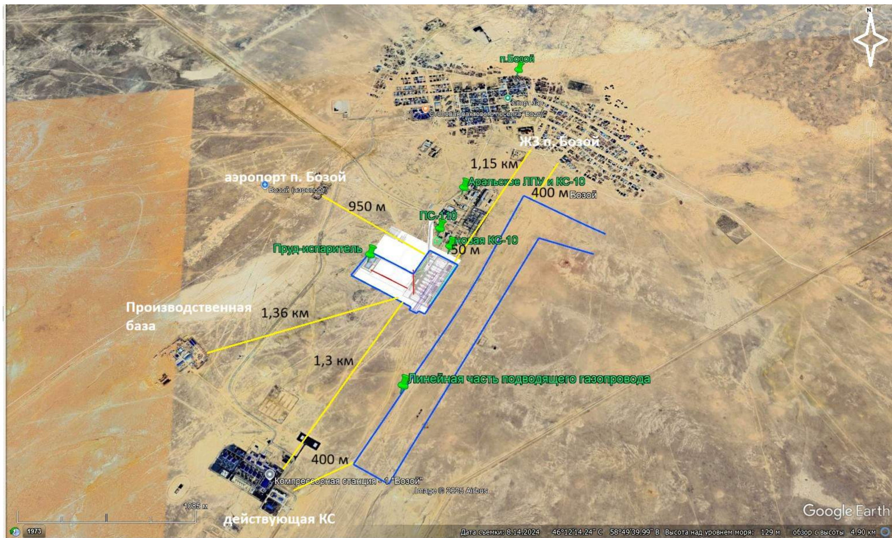
Рис.2 Ситуационная схема расположения проектируемой КС-10 по отношению к окружающим предприятиям и п. Бозой Масштаб 1:271 м
