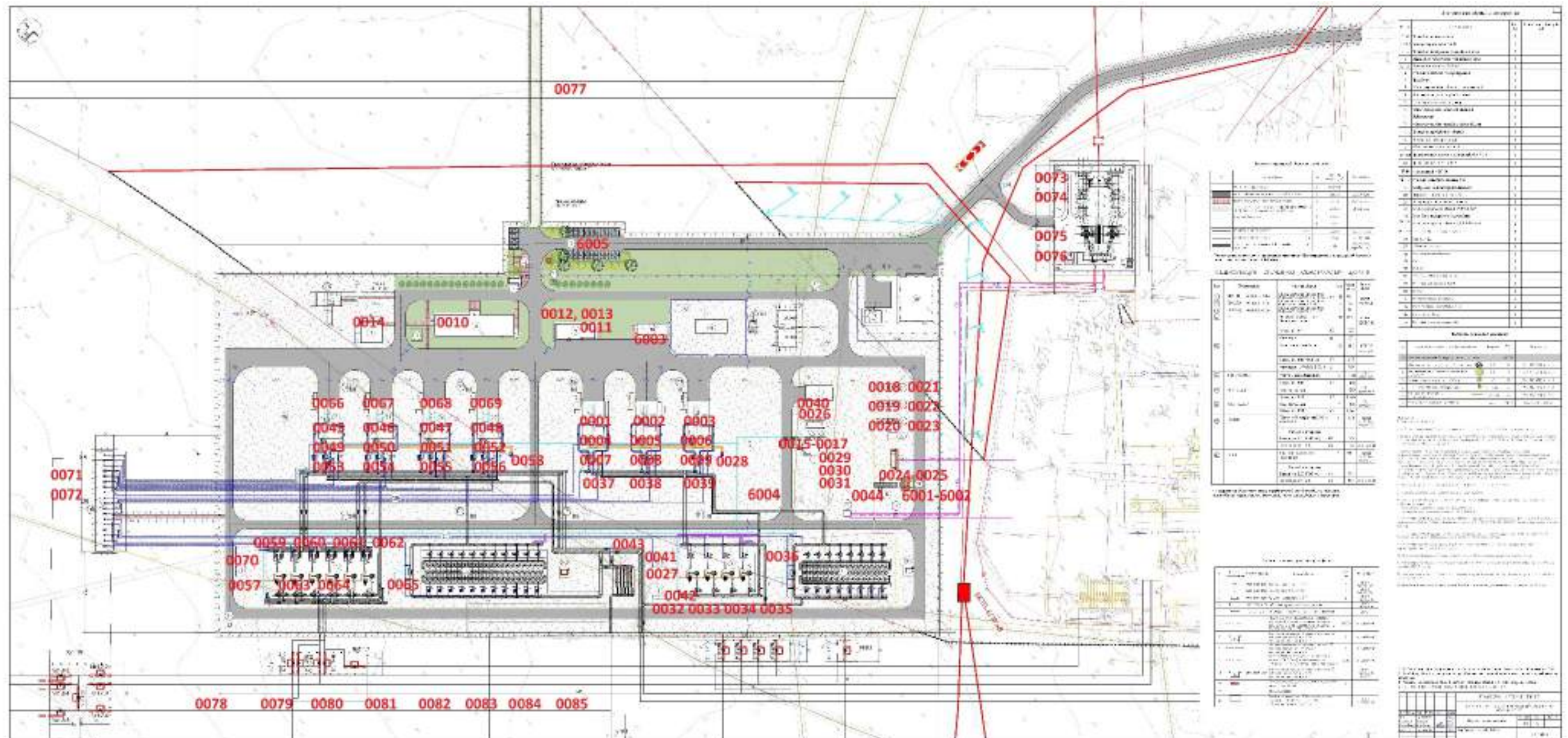
Рис.33 Генплан проектируемых объектов с ИВА
