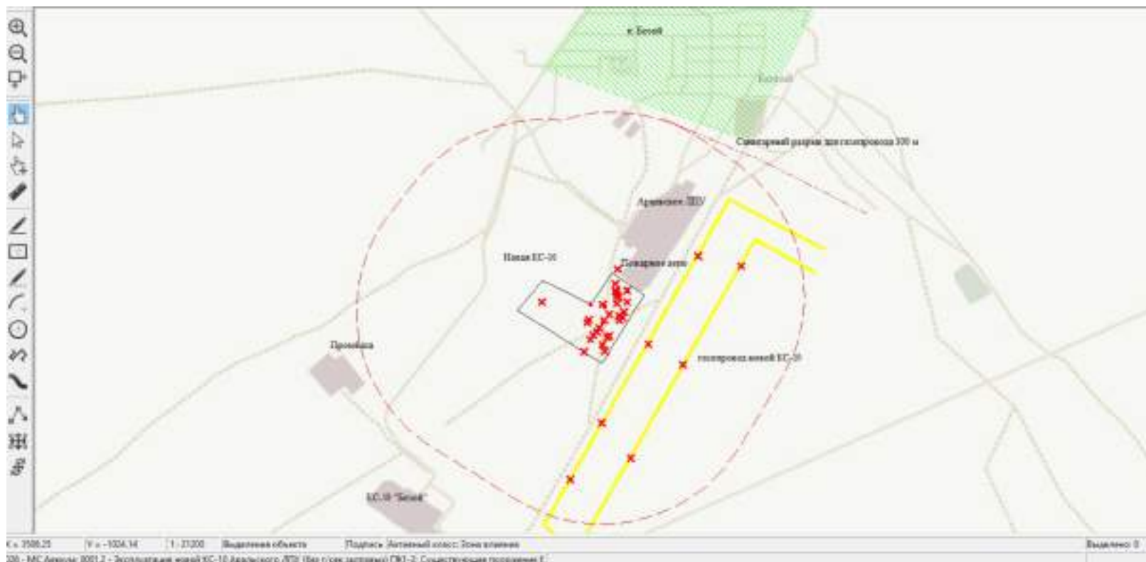
Рис. 37 Проектируемая новая КС-10 с СЗЗ 1000 м
