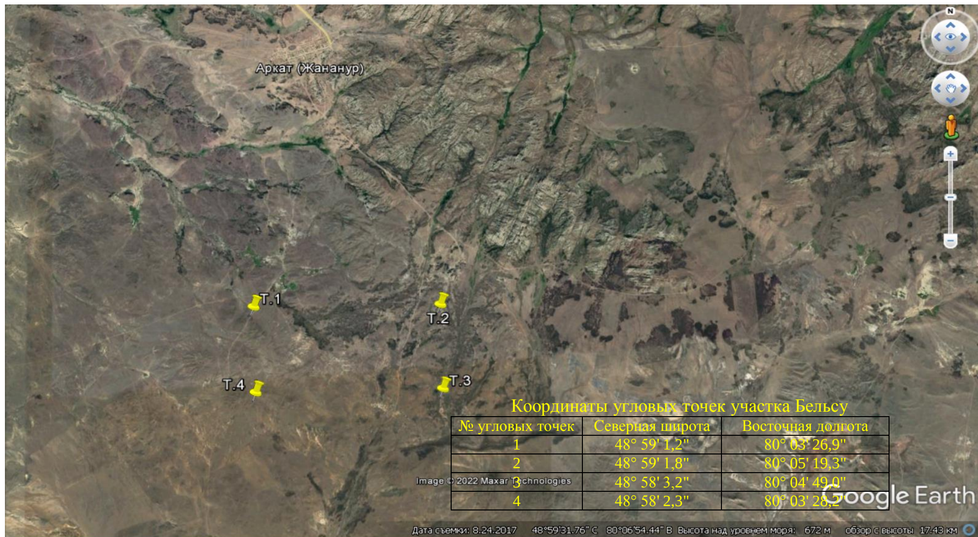
Рисунок 2 - Координаты месторождения
