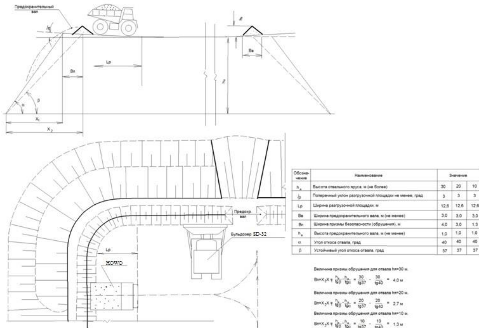
Рисунок 8 - Технологическая схема отвалообразования
