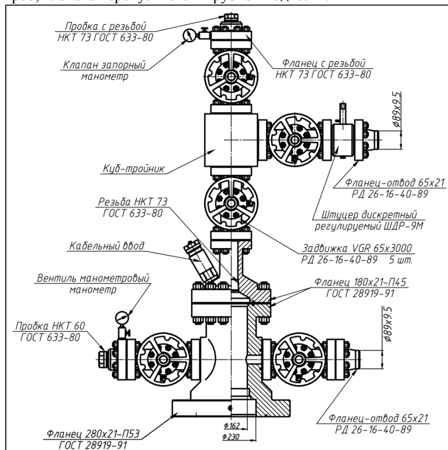
Рисунок Ошибка! Текст указанного стиля в документе отсутствует. 1. Устьевая арматура УЭЦН
