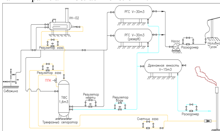
Рисунок 8. Принципиальная индивидуальная технологическая схема сбора жидкости по скважинам на период пробной эксплуатации месторождения Майкыз
