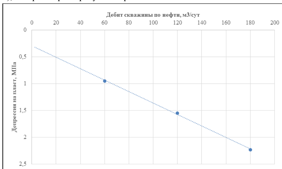
Рисунок 4. Индикаторная диаграмма по скважине М-4. Интервал опробования – 1703,0-1710,0 м
