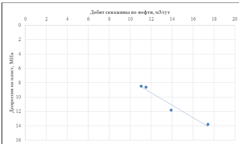
Рисунок 5. Индикаторная диаграмма по скважине ЮМ-1. Интервал опробования – 2073,2-2075,8 м
