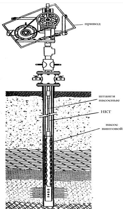
Рисунок 7. Винтовой насос с приводом на устье скважины
