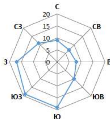
Рисунок 2.2 – Годовая роза ветров
