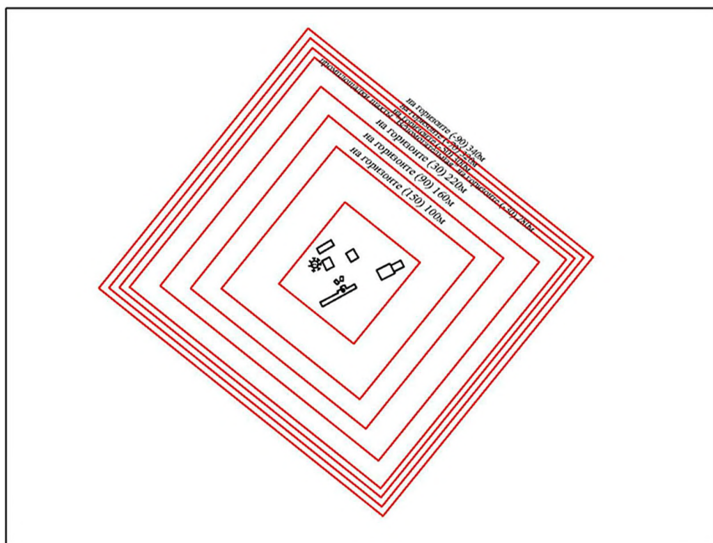
Рисунок 4. Схема размещения охранного целика шахты «Вспомогательная»
