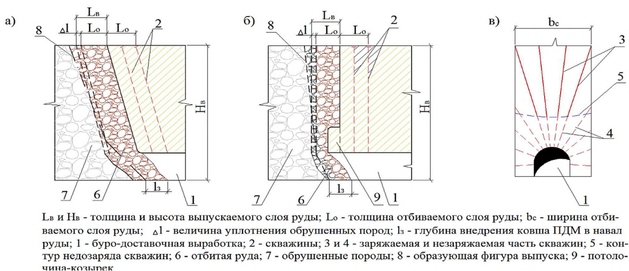
Рисунок 20. Технологические схемы послойного торцевого выпуска руды с отбойкой наклонными (а) и вертикальными (б) скважинами; формирование потолочины-козырька недозарядом скважин (в).
