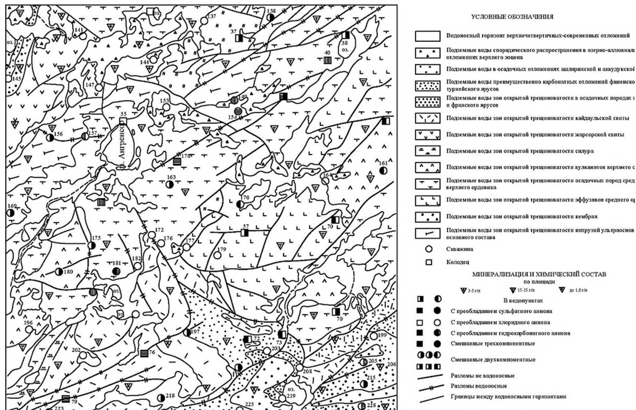
Рисунок 3. Схематическая гидрогеологическая карта.
