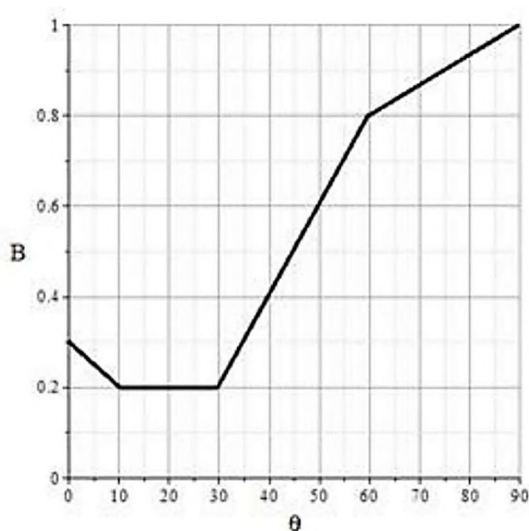
Рисунок 24. График для определения параметра В.
