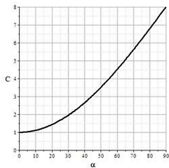
Рисунок 25. График для определения параметра С.
