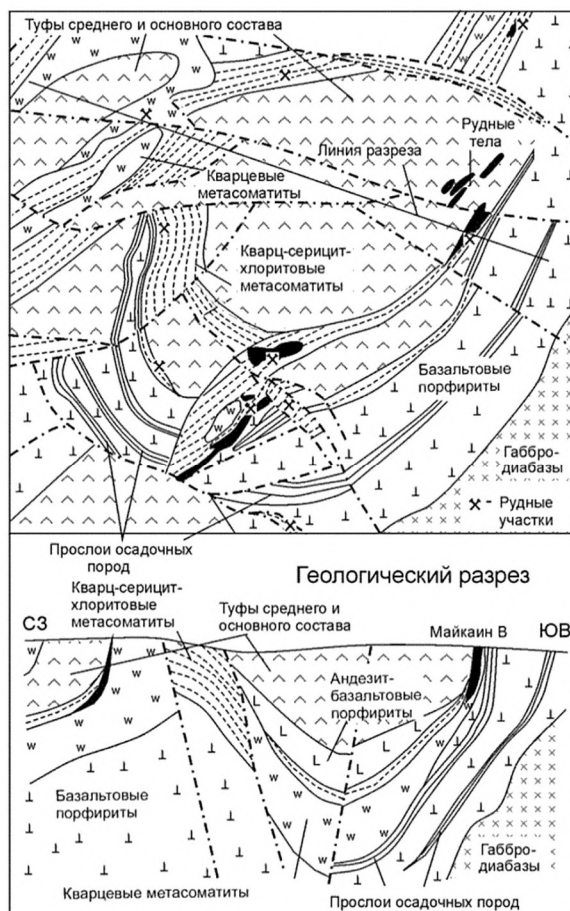
Рисунок 2. Схема геологического строения и геологический разрез Майкаинского рудника.
