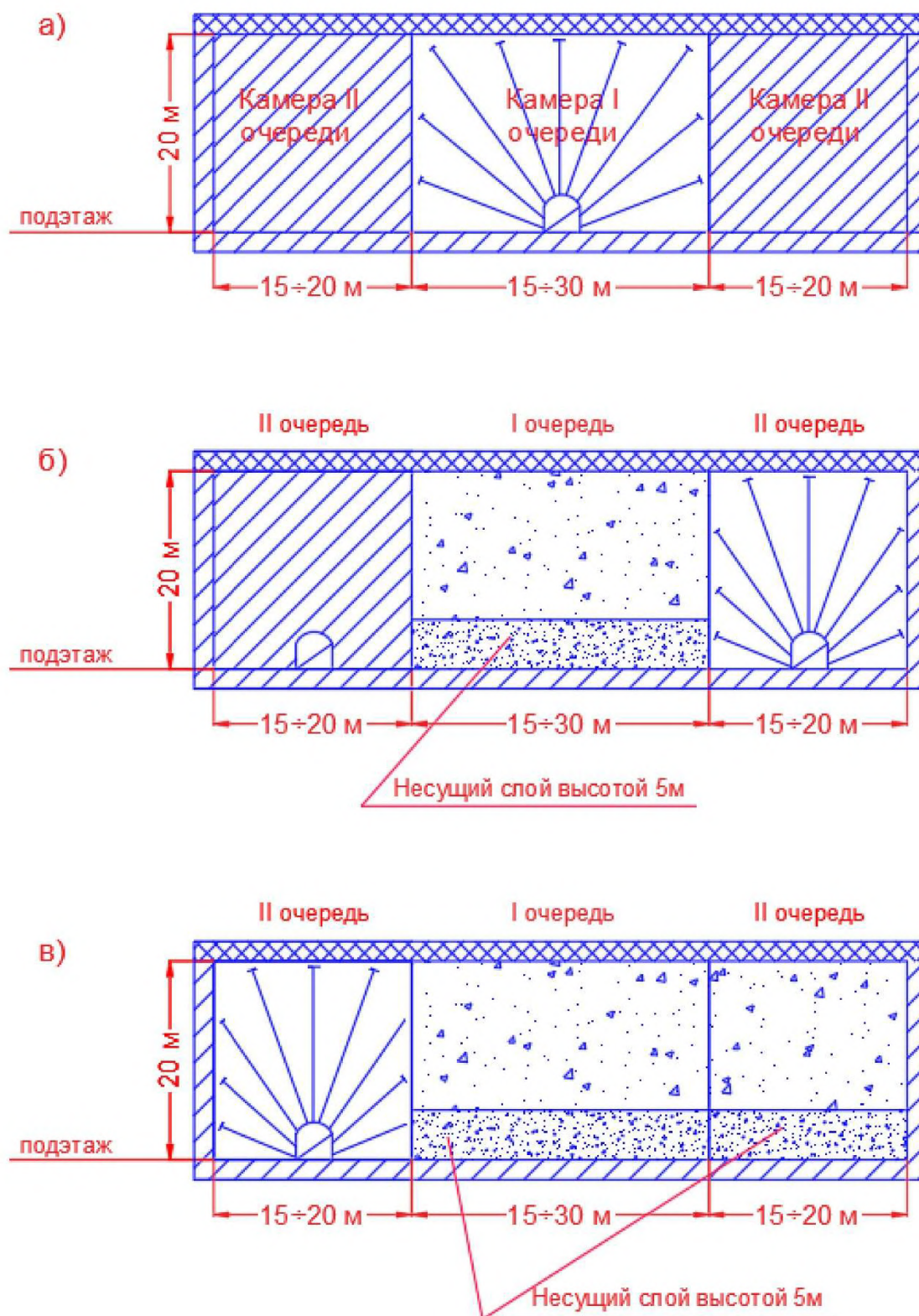
Рисунок 13. Порядок отработки запасов блока на подэтаже при подэтажно-камерной системе разработки с твердеющей закладкой выработанного пространства.
