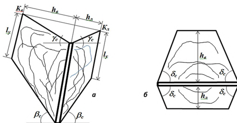
а – на разрезе вкрест простирания (длина обрабатываемого блока по простиранию больше пролета по падению); б – в плане.
