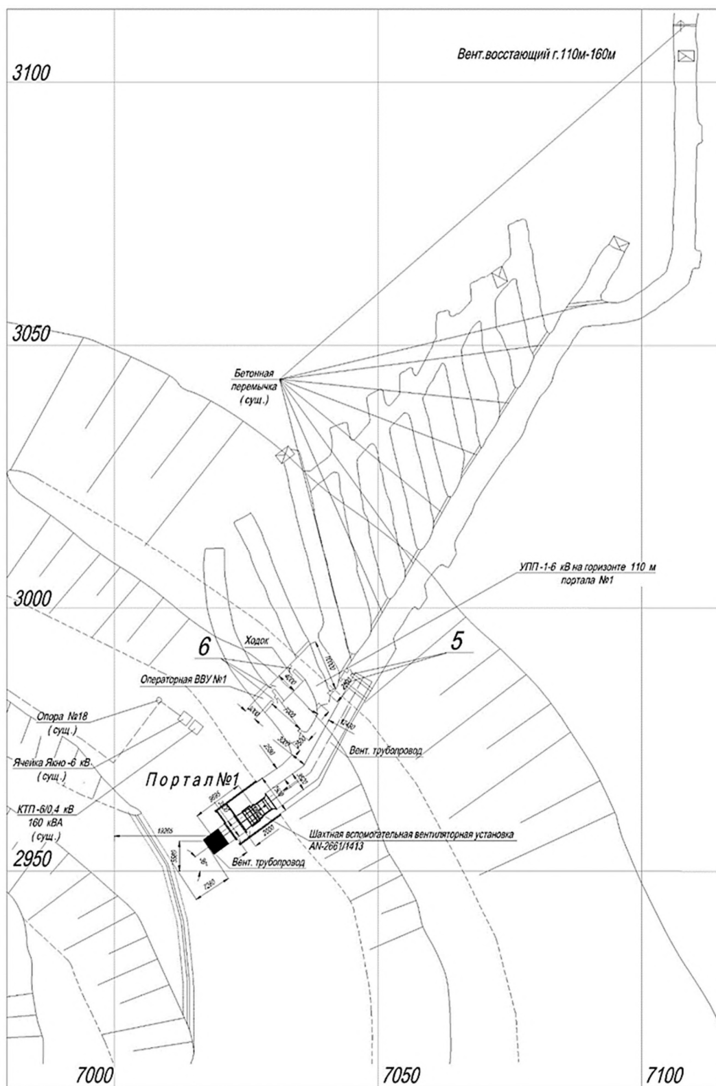
Рисунок 10. Схема размещения вспомогательной вентиляционной установки на плане портала № 1 горизонта 110 м.
