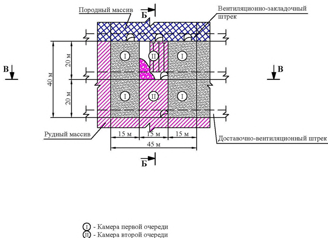
Рисунок 14. Схема отработки двух смежных подэтажей при подэтажно-камерной системе разработки с твердеющей закладкой выработанного пространства.
