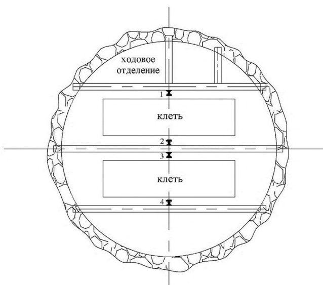
Рисунок 8. Схема сечения ствола шахты «Капитальная».
