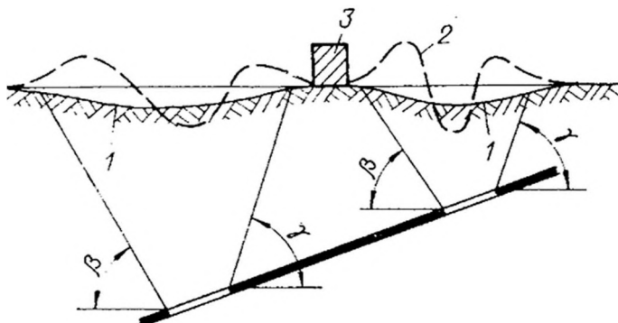
Рисунок 7. Схема построения охранного целика.
