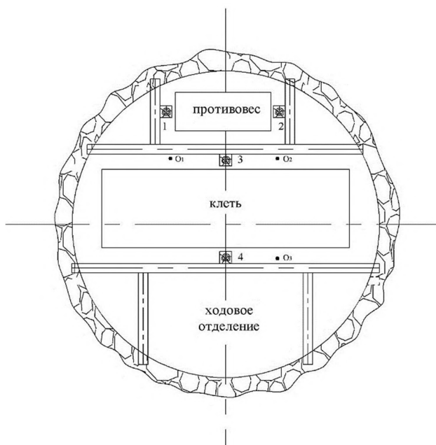
Рисунок 9. Схема сечения ствола шахты «Вспомогательная».
