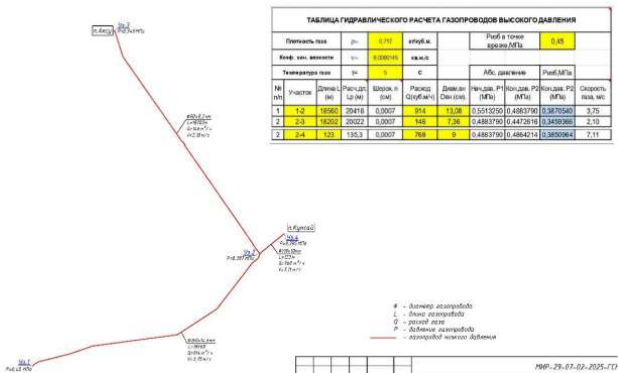
Гидравлический расчет газопровода высокого давления
