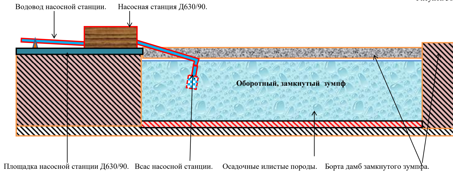
Схема насосной станции – Д 630/90 в замкнутом, оборотном зумпфе.
