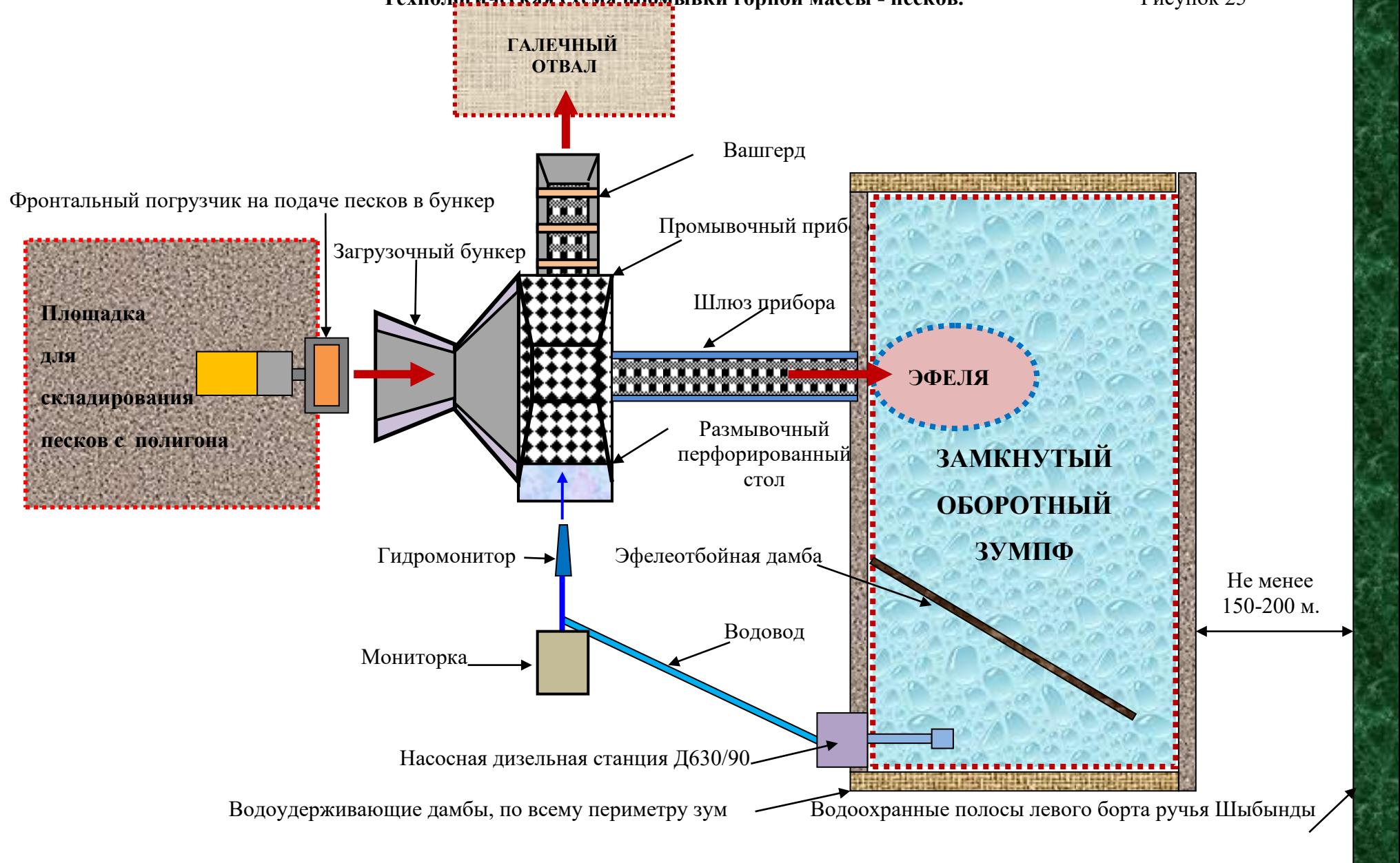
Технологическая схема промывки горной массы - песков.
