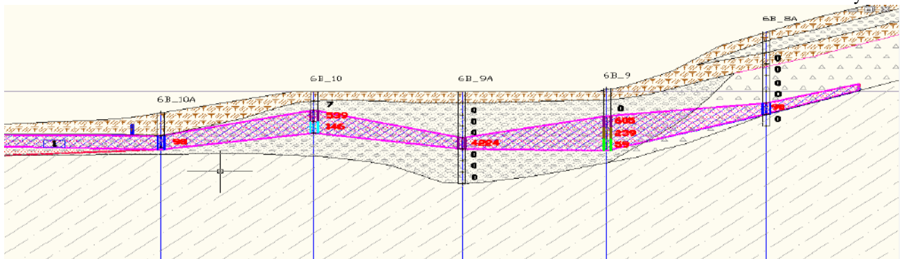
Вертикальный разрез по линии 6Б.
