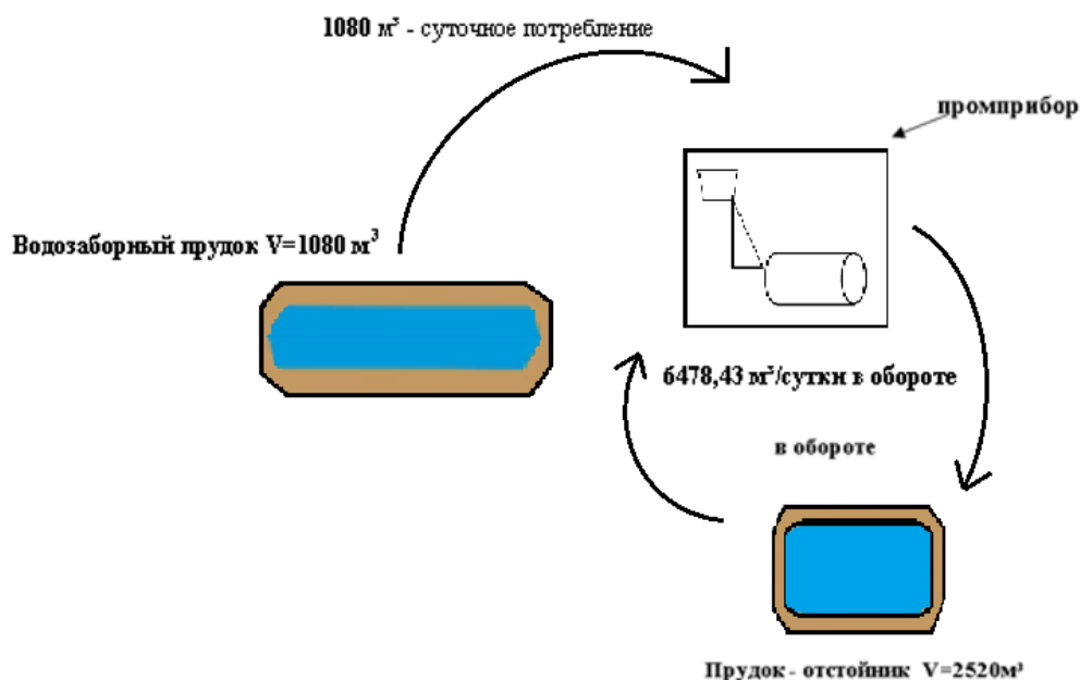
Рисунок – Схема движения воды для технологического процесса
