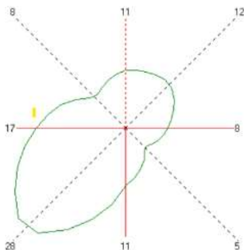
Рисунок 20.1 Среднегодовая роза ветров, %
