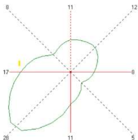
Рисунок 1.2 Среднегодовая роза ветров, %
