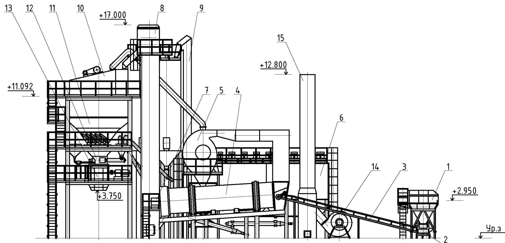
Рисунок 4 – Схема асфальто-бетонного завода марки QLB-2000
