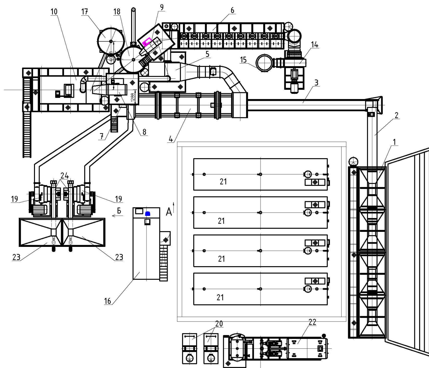
Рисунок 3— Схема асфальто-бетонного завода марки QLB-2000
