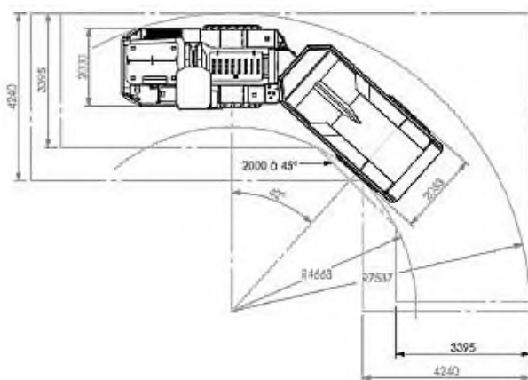
РАДИУС ПОВОРОТА
