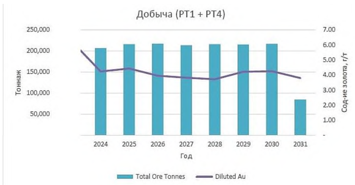
Рисунок 20. График объемов добычи руды (Рудное тело 1 + Рудное тело 4), включая руду с проходки.
