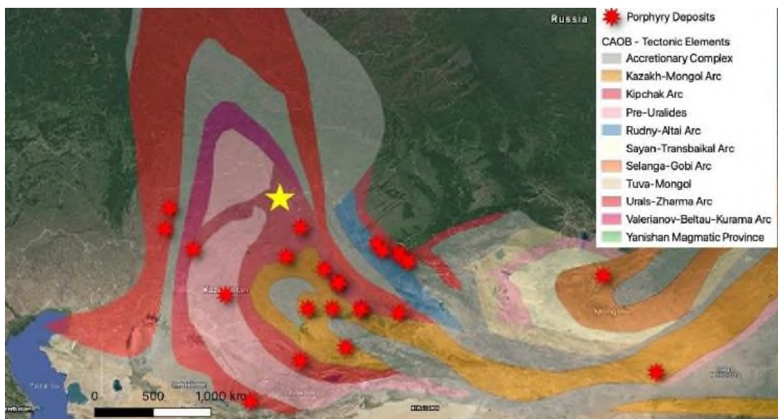
Рисунок 2. Схематическая карта палеозойских отложений Казахстана, показывающая положение месторождения Кварцитовые горки в пределах Казахстанского орогена; месторождение Кварцитовые горки показано желтой звездой (заимствовано у Windley и др. (2007 г.) и переработано).
