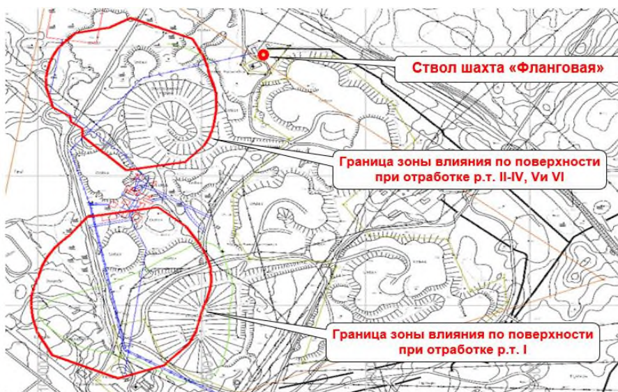
Рисунок 19. Границы зоны влияния по поверхности при отработке запасов рудных тел.
