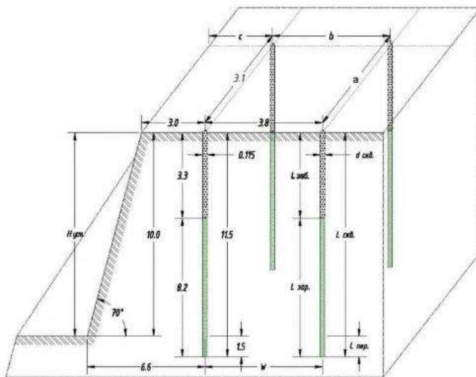
Рисунок 1.3 Параметры конструкции скважинного заряда на вскрыше
