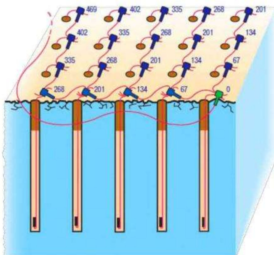
Рисунок 1.5 Схема монтажа взрывной сети при производстве буровзрывных
